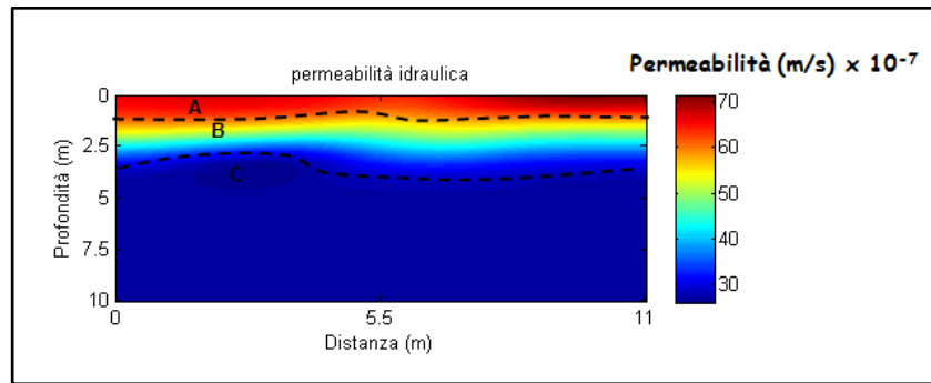
FIG. 30 - Modello di distribuzione della permeabilità e della resistenza meccanica a compressione a varie profondità.
