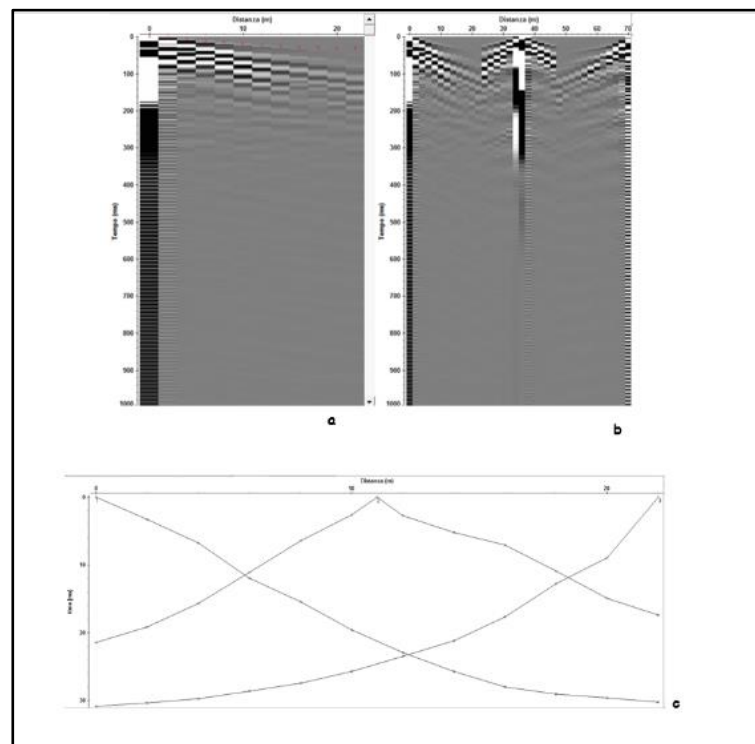
FIG. 32 - a) sismogrammi delle 3 energizzazioni; b) esempio di picking dei primi arrivi; c) Dromocrone relative al profilo sismico.
