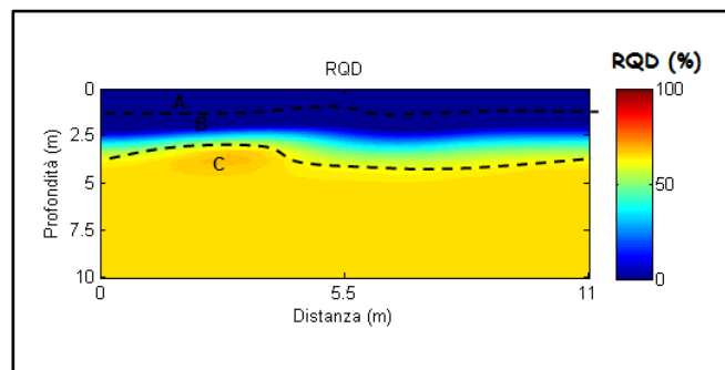
FIG.28 - Modello di distribuzione di RQD a varie profondità.
