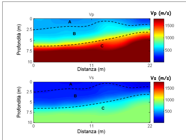
FIG.33 - Modello di distribuzione delle velocità V_p e V_s a varie profondità.
