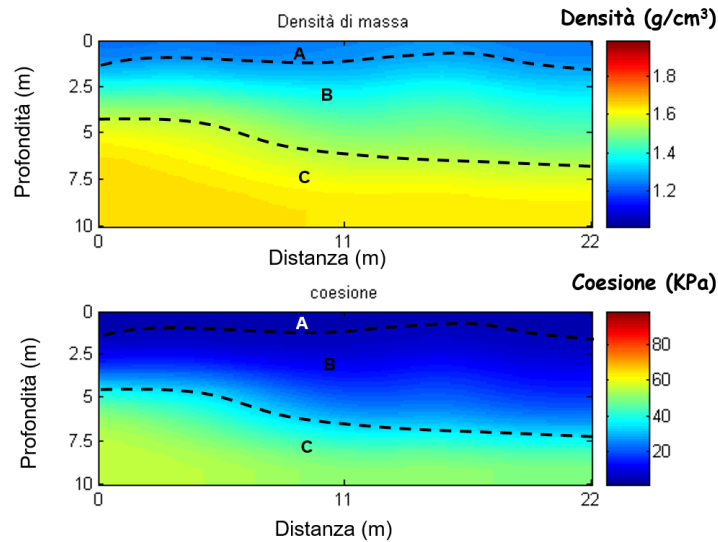
FIG.23 - Modello di distribuzione della densità di massa e della coesione a varie profondità.
