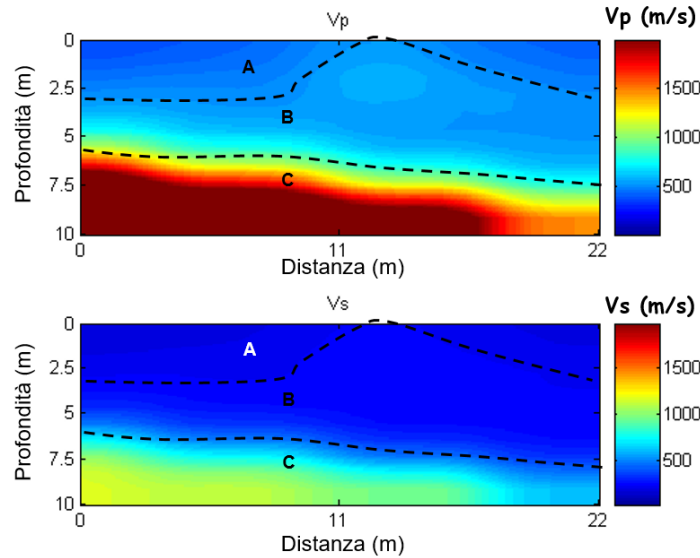
FIG.15 - Modello di distribuzione delle velocità V_p e V_s a varie profondità.
