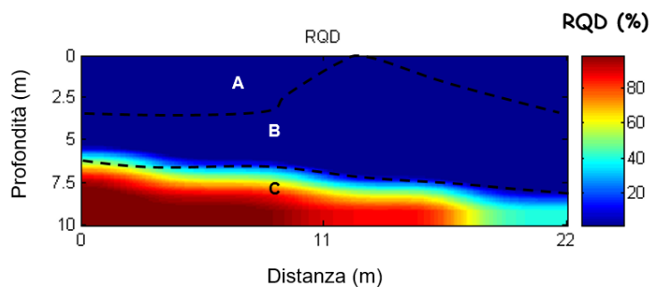
FIG.16 - Modello di distribuzione di RQD a varie profondità
