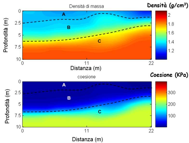
FIG.35 - Modello di distribuzione della densità di massa e della coesione a varie profondità.
