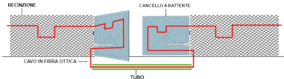
Figura 4.12 - Schema di installazione cavo in fibra ottica su recinzione.
