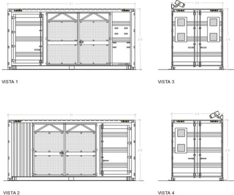
Figura 4.7 – Posizionamento sistema video sorveglianza e illuminazione esterna Power Station
