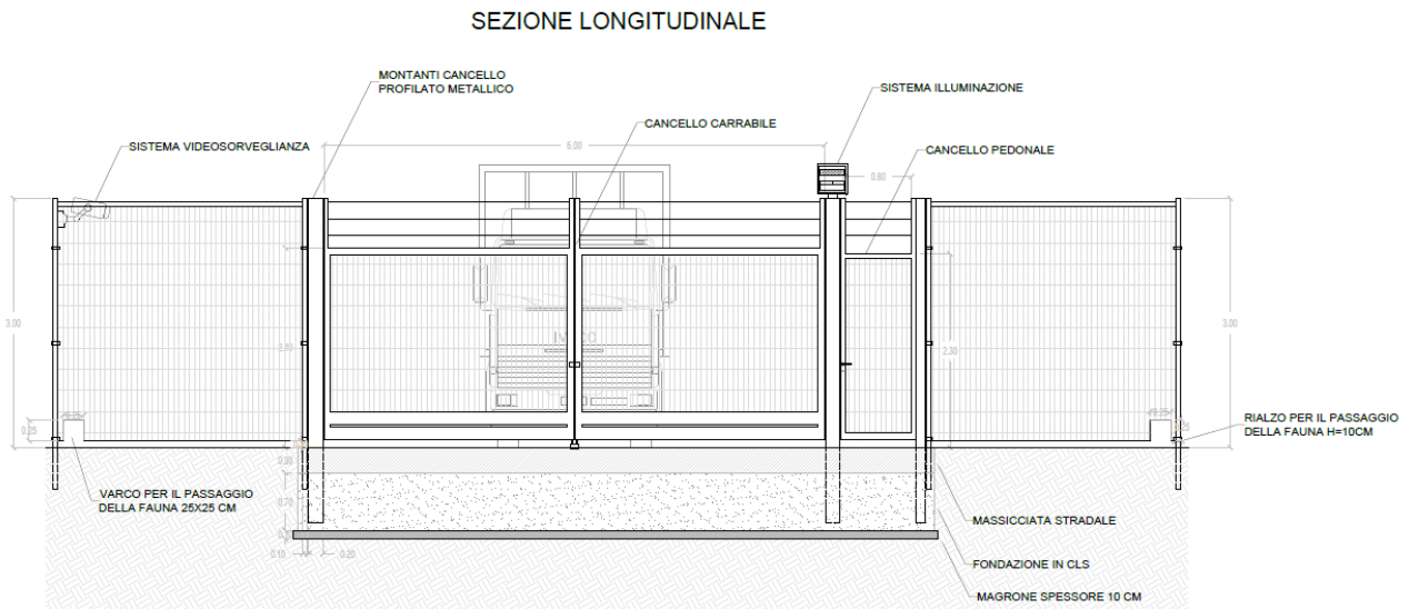
Figura 4.9 - Posizionamento sistema video sorveglianza e illuminazione esterna cancelli
