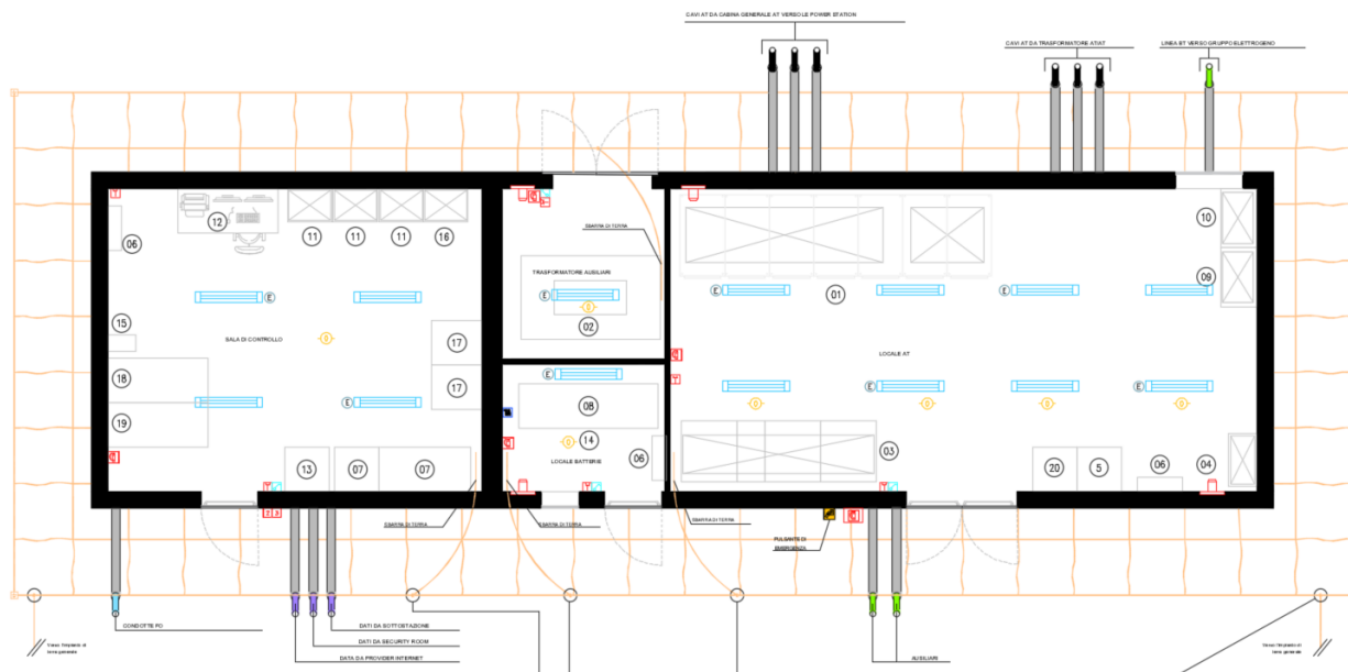
Figura 4.4 - Posizionamento plafoniere nella cabina AT.
