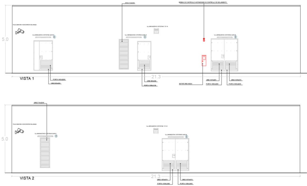
Figura 4.8 - Posizionamento sistema video sorveglianza e illuminazione esterna Gabina Generale AT
