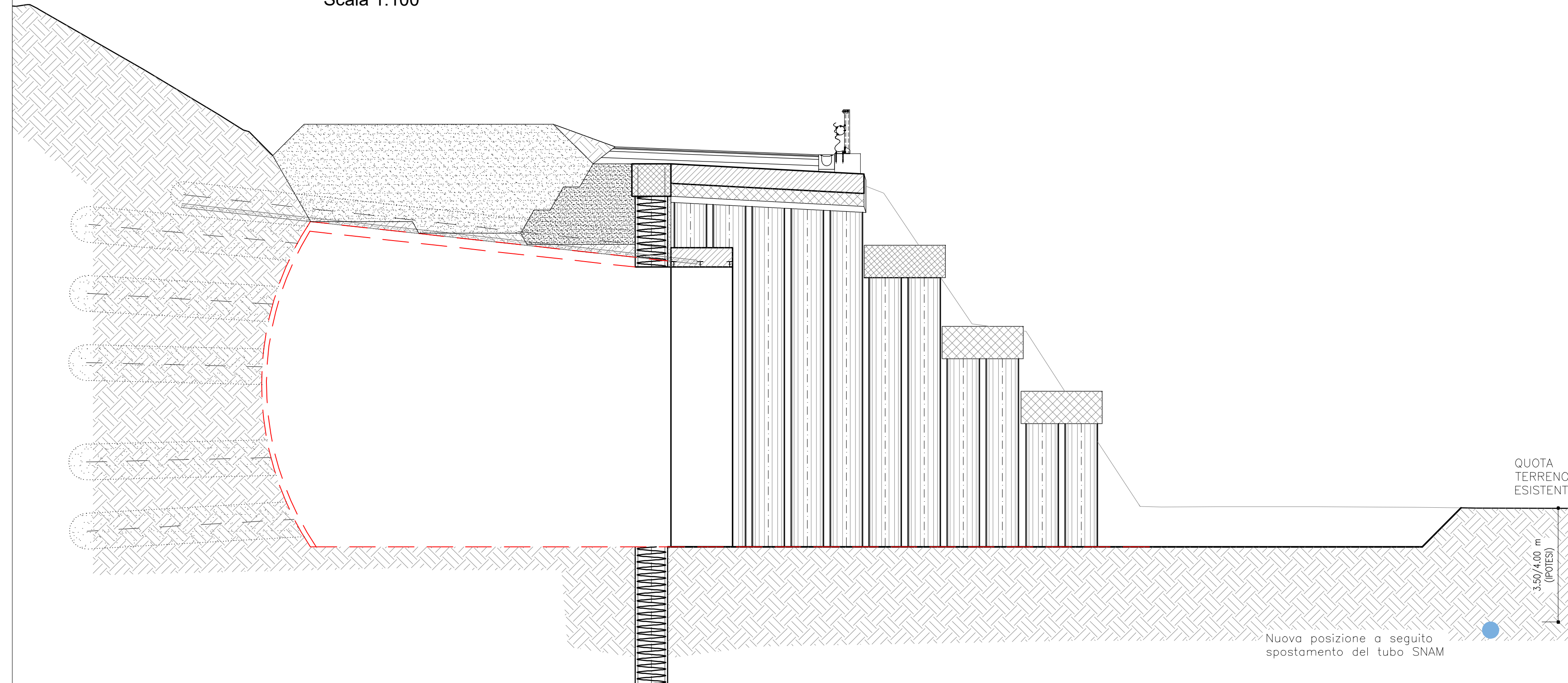
Fase 21: Scavo del primo conco e parziale getto dell'arco rovescio (le fasi costruttive del conco di attacco sono dettagliate negli elaborati specifici) Scala 1:100
