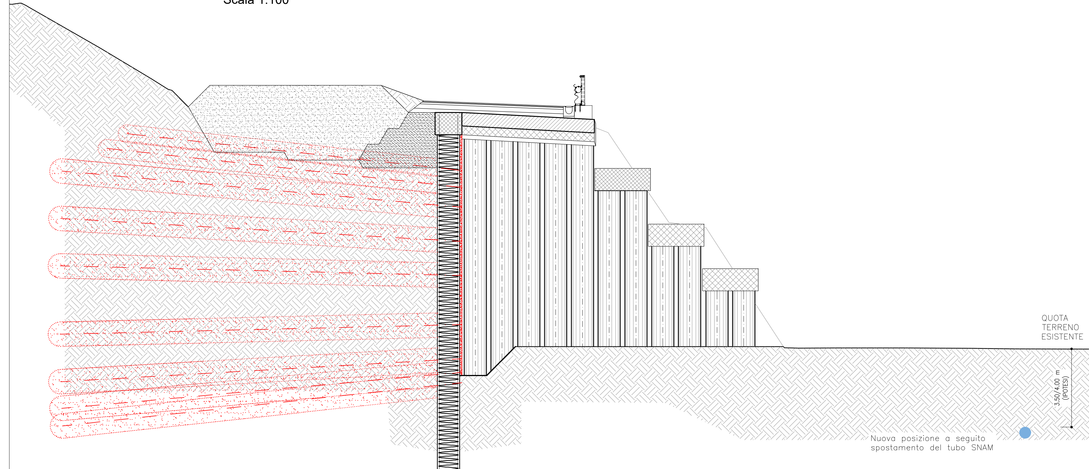
Fase 17: Applicazione di spritz-beton armato al fronte della paratia e realizzazione dei trattamenti in Jet Grouting al fronte e contorno Scala 1:100
