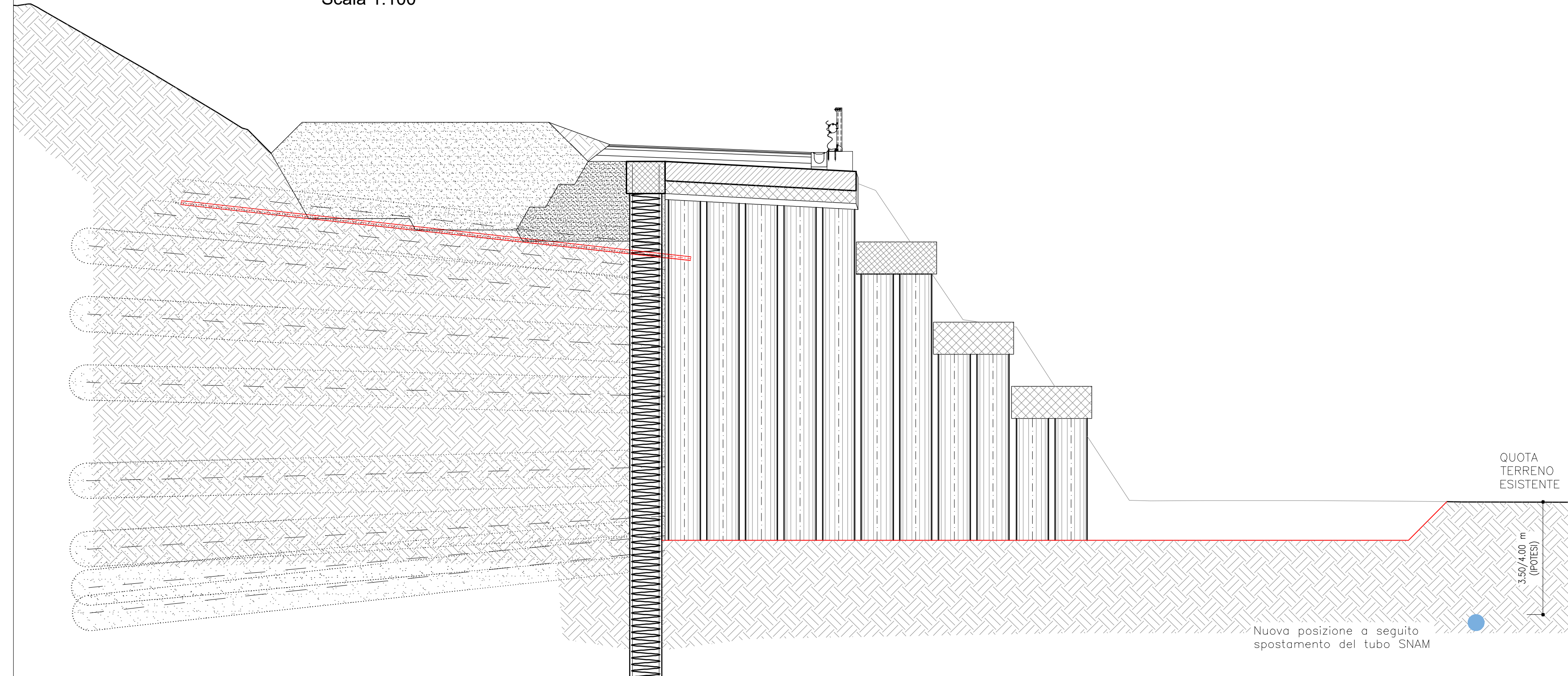
Fase 18: Realizzazione infilaggi metallici al fronte della galleria e abbassamento del fondo scavo alla quota di scavo della galleria Scala 1:100
