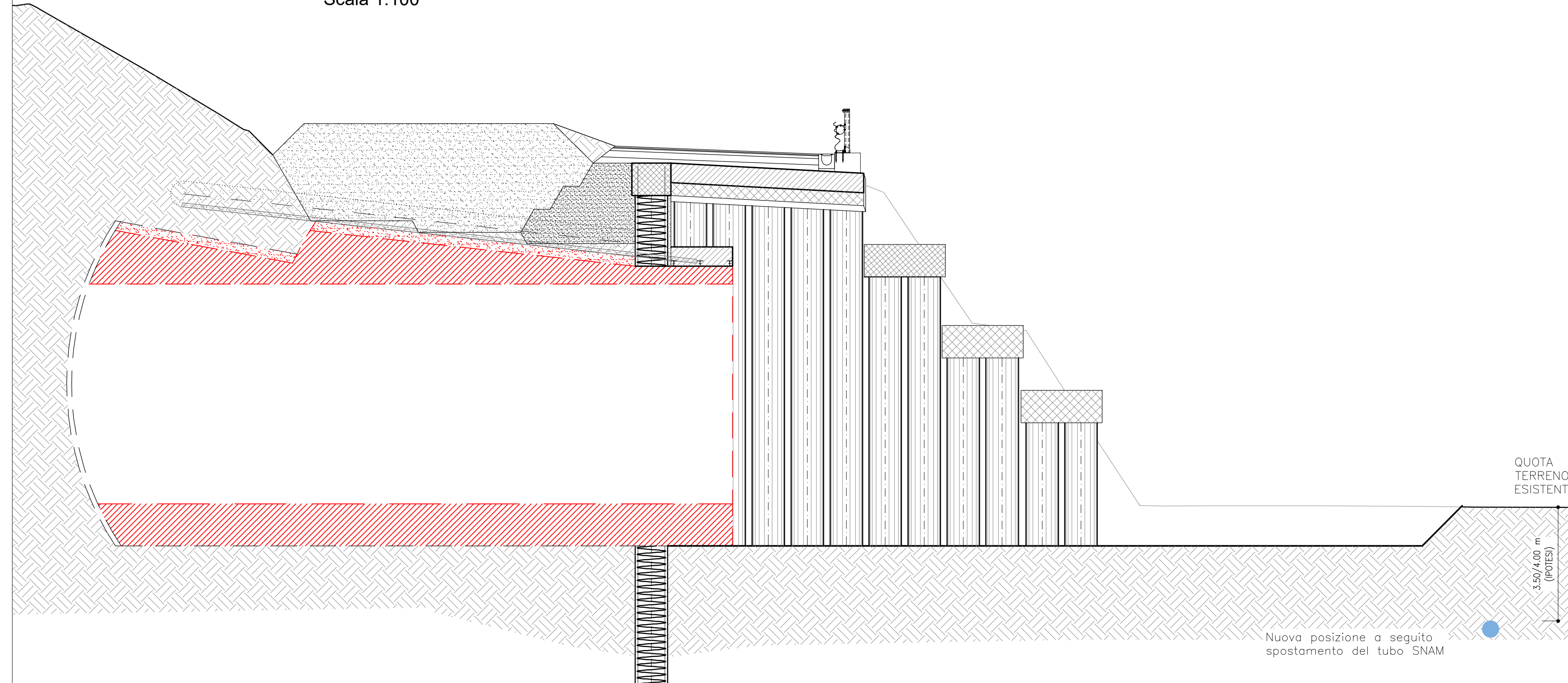
Fase 22: Realizzazione del rivestimento definitivo della sezione di attacco, scavo e rivestimento dei conchi successivi (come da tavole specifiche) Scala 1:100
