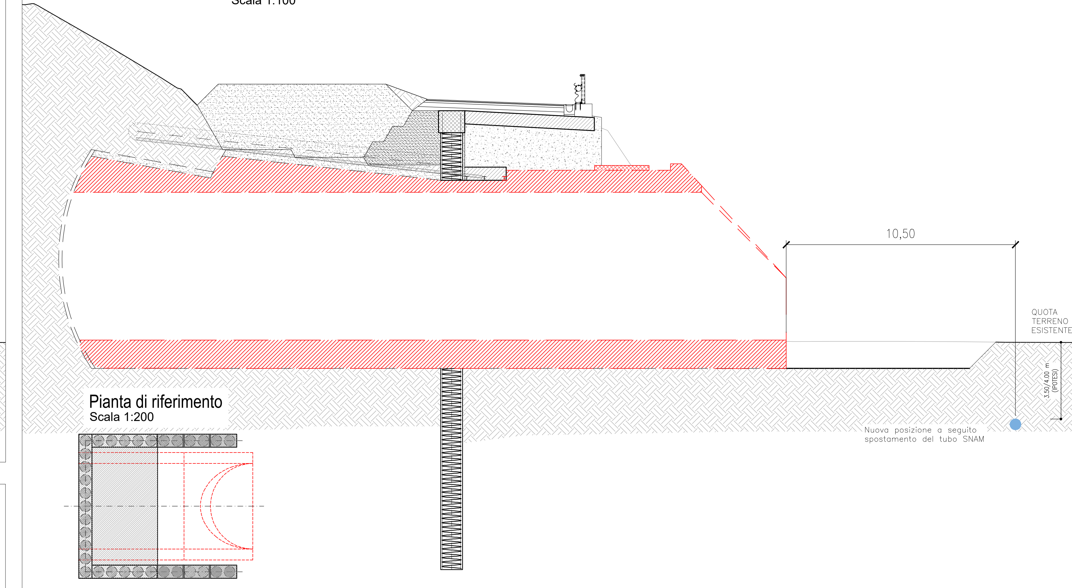
Fase 24: Demolizione protesi con ripristino dello stato dei luoghi a monte della SP 242 e sistemazione definitiva delle opere di imbocco Scala 1:100
