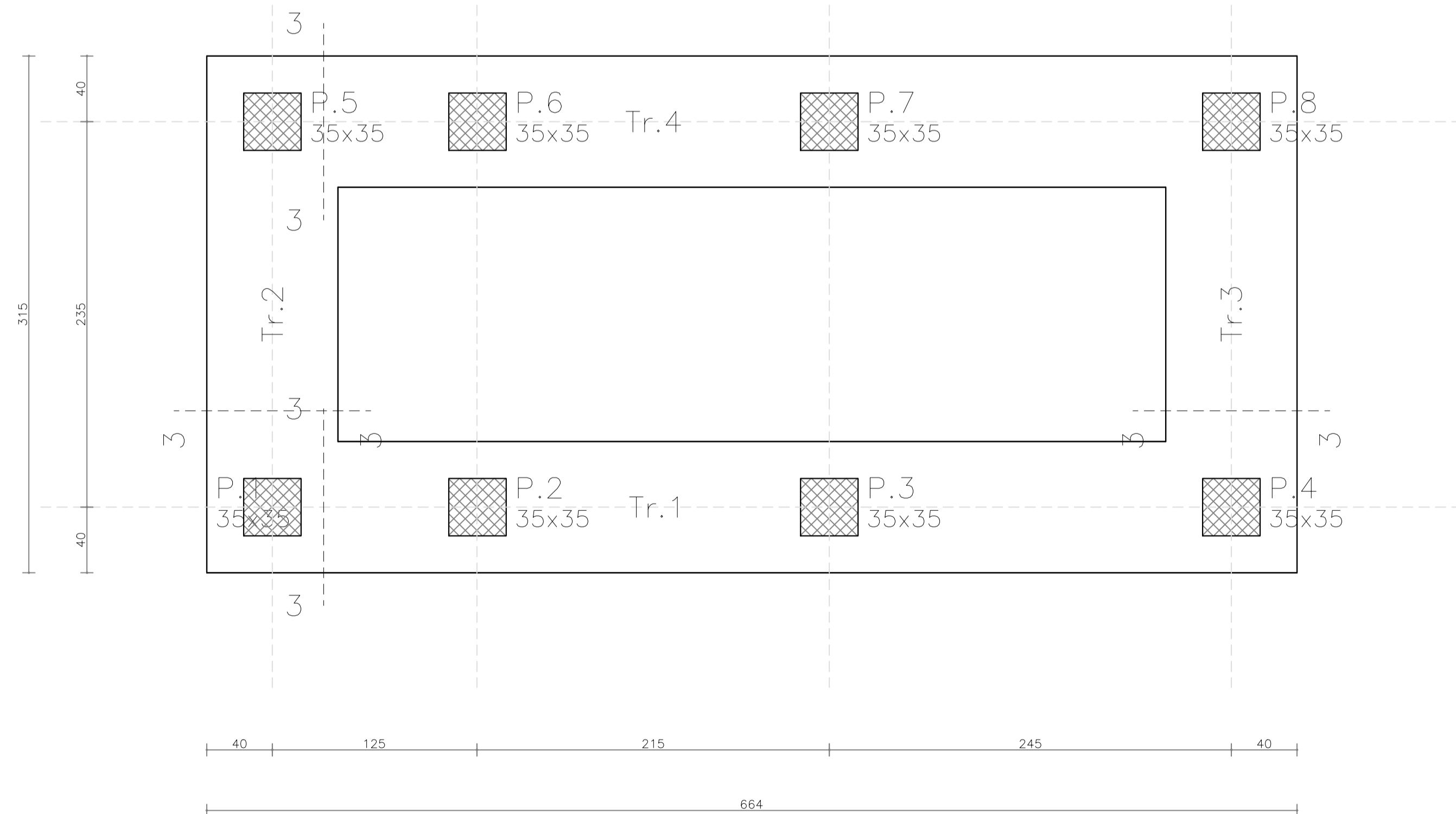
Pianta a quota -40,0
