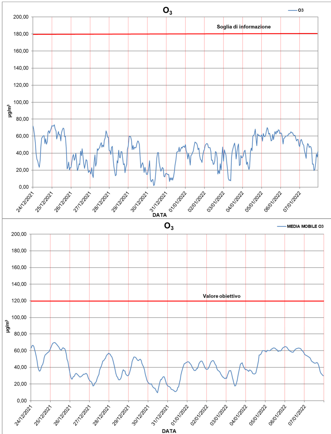
Figura 36 Confronto tra le concentrazioni medie orarie di ozono su 24 h e su 8h e limiti normativi (rispettivamente soglia di informazione e valore obiettivo)
