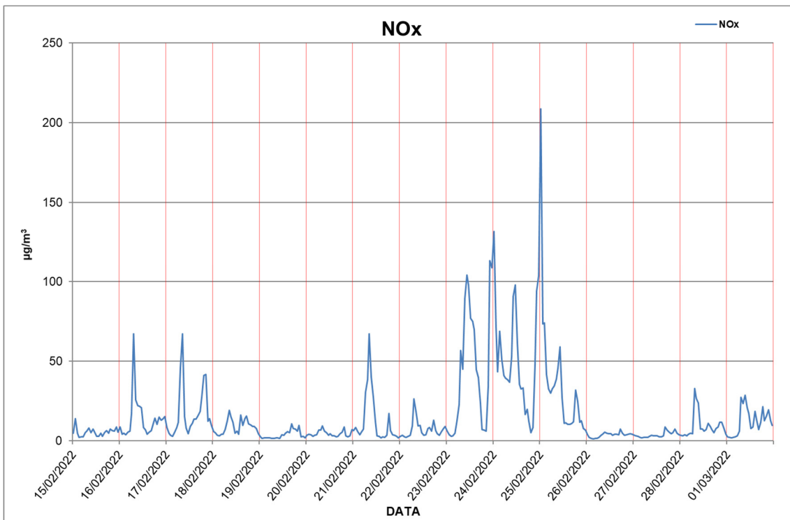
Figura 53 Concentrazioni medie orarie rilevate di Nox
