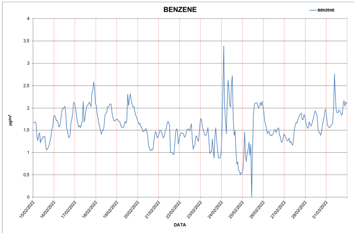
Figura 55 Concentrazioni medie orarie rilevate di benzene
