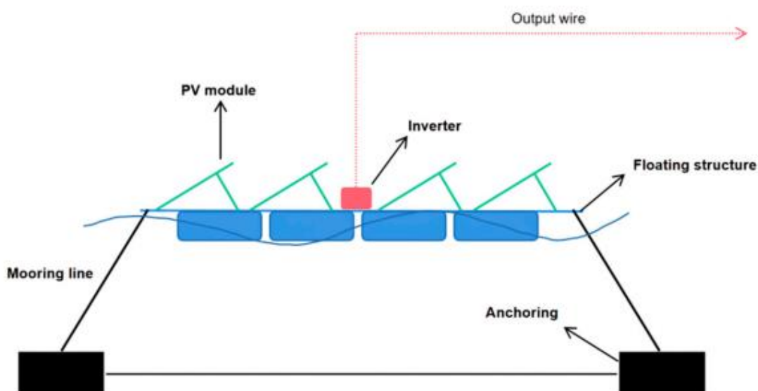
Figura 5-3. Ancoraggio tramite catenarie tensionate
