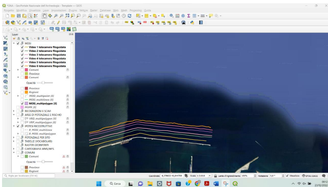
Figura 9-8: Tracciato delle 6 rotte ROV per l’analisi ambientale (superiore di oltre il 50% l’area delle lavorazioni) posizionate sul Template ministeriale GNA mare
