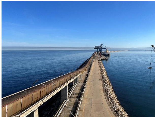
Figura 6-6: Area di radicamento della diga foranea e cavidotto
