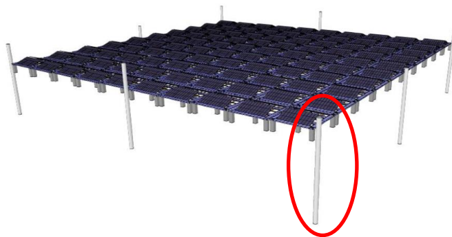
Figura 5-1: Ancoraggio tramite palificazione
