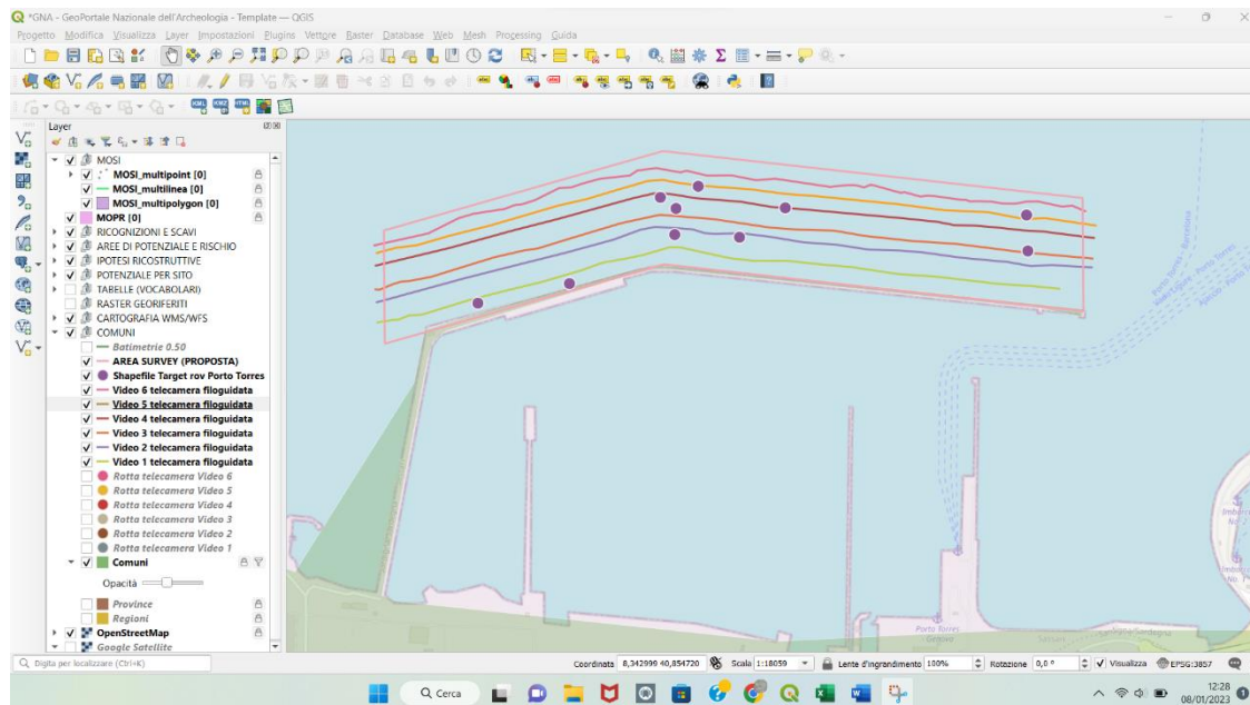
Figura 9–10: Sovrapposizione Target ROV, identificati per finalità ambientali, su rotte ROV
