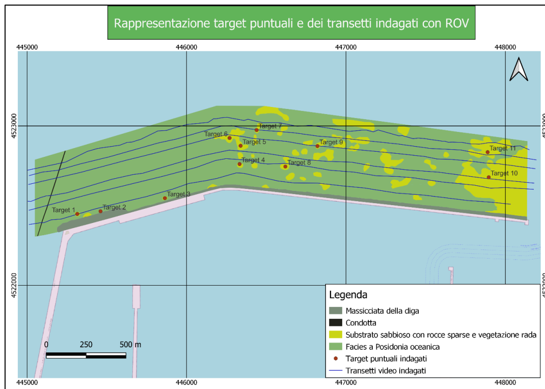
Figura 9-2: Rappresentazione target puntuali e dei transetti indagati con ROV. Da Relazione Ambientale, Rev. 01
