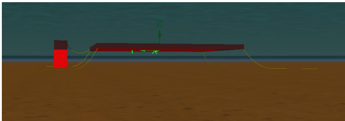
Figura 5-2: Ancoraggio tramite catenarie e corpi morti
