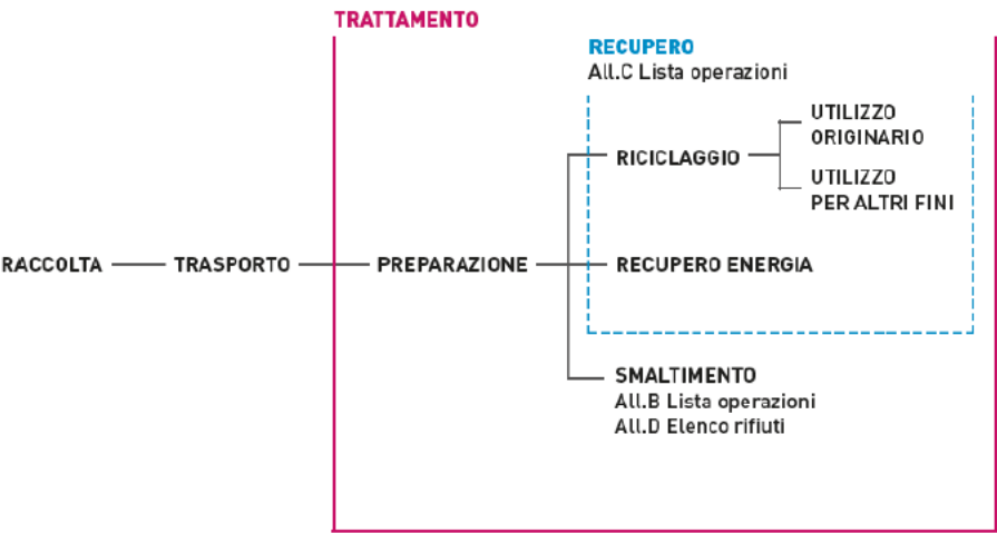
Fig.2 - Le fasi di gestione dei rifiuti generati da moduli fotovoltaici a fine vita (D.Lgs. 49/2014)
