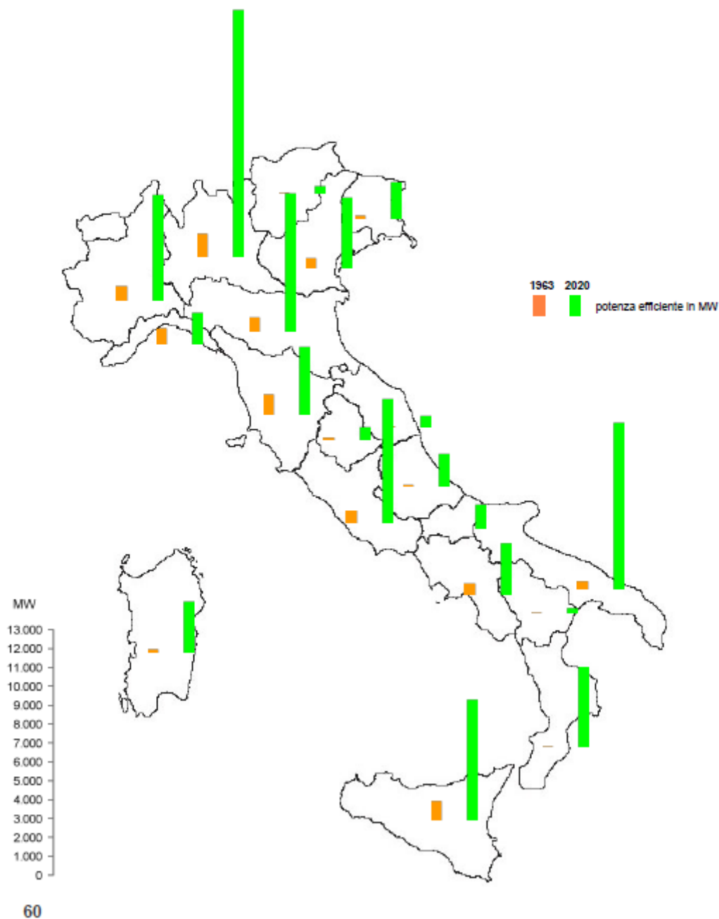
Figura 25 - Produzione termoelettrica regioni italiane
