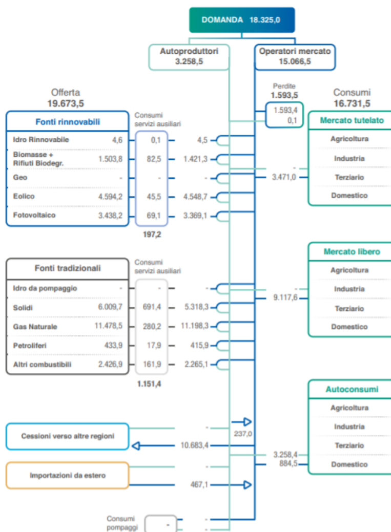
Figura 30 - flussi di energia elettrica, Puglia
