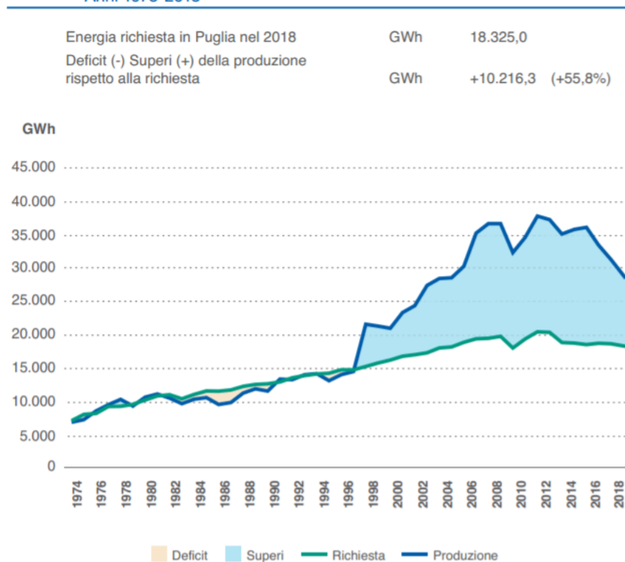
Figura 26- Puglia, bilancio energetico
