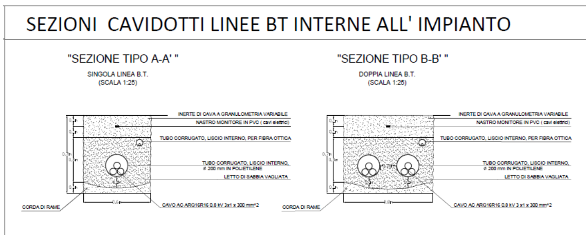
Figura 44- Cavidotti BT interni
