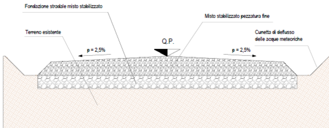
Figura 50- Sezione-tipo strade interne in misto stabilizzato
