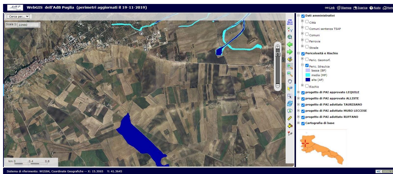
Figura 14 - aree di Pericolosità idrauliche
