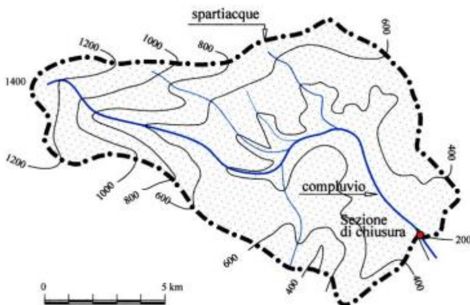
Figura 36 - Mappa bacino topografico
