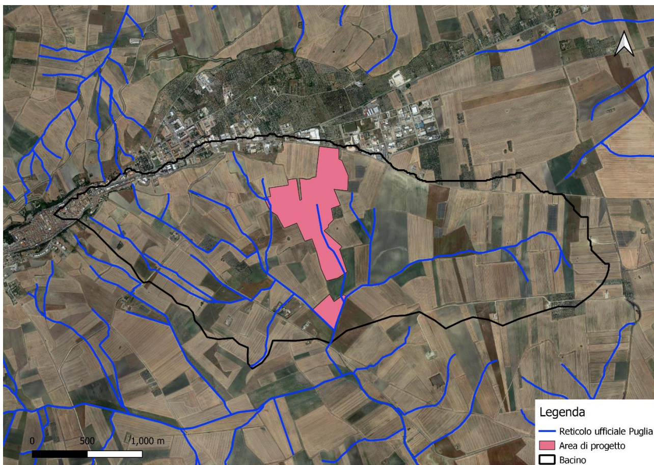
Figura 75 - Idrologia del sito
