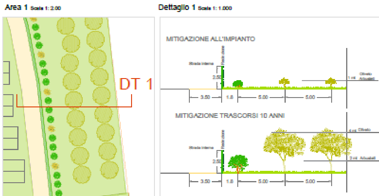
Figura 107 - Esempio, particolare mitigazione piastra 1
