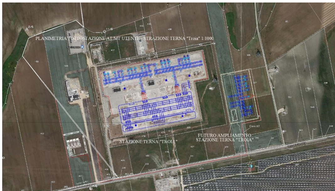
Figura 45- Sottostazione
