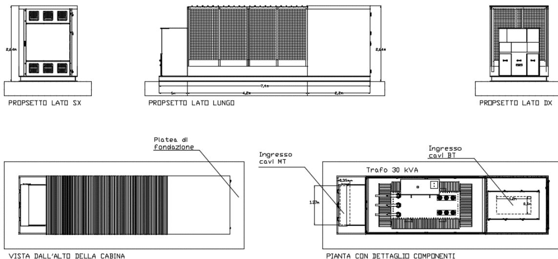
Figura 41 – Cabina tipo MT/BT
