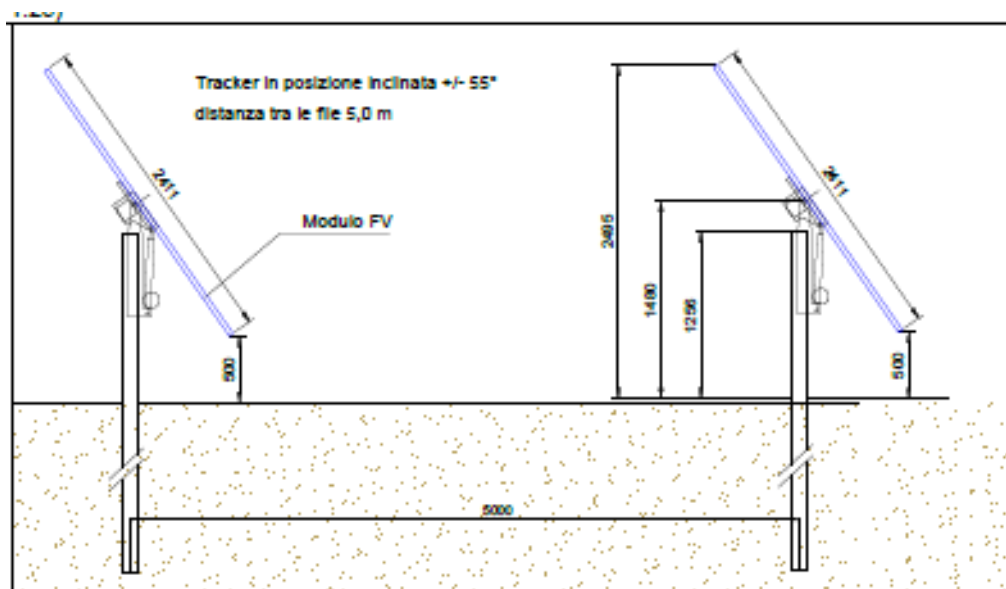
Figura 39- Tracker
