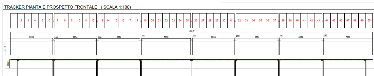
Figura 40 - Particolare del montaggio dei tracker Convert TRJ
