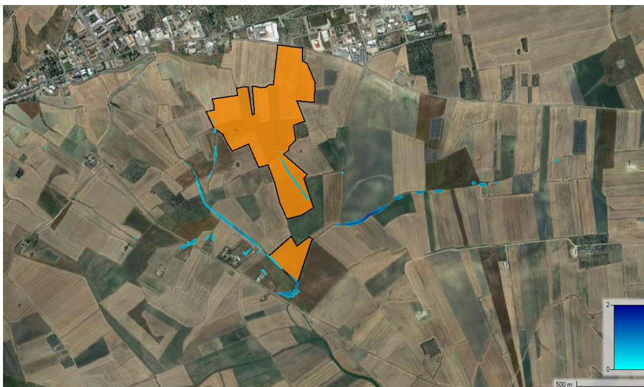
Figura 80- Mappatura delle aree a deflusso critico con Tempo di Ritorno a 200 anni e impianto
