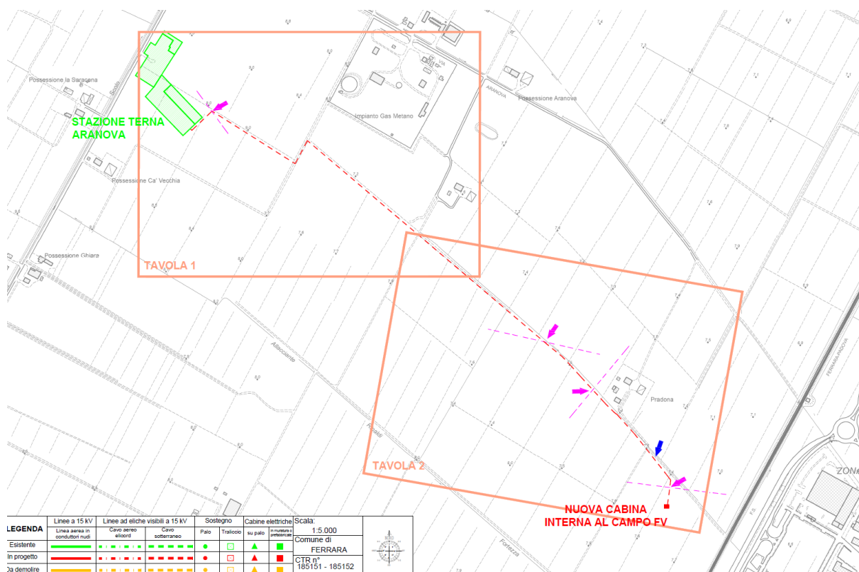
Figura 2: Tracciato elettrodotta interrato
