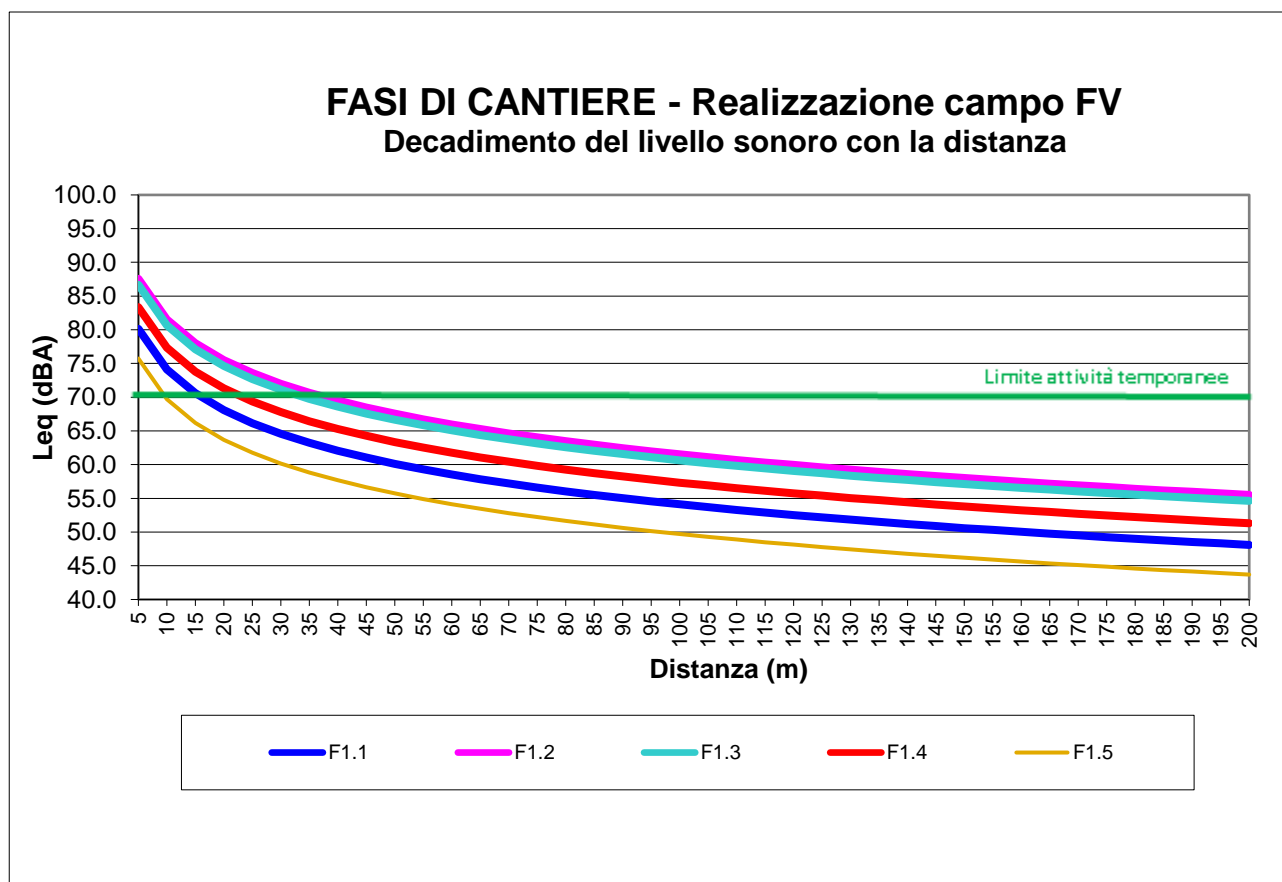
Figura 9: curve di decadimento dell'energia sonora relativa alle sottofasi di cantiere per la realizzazione del campo FV.
