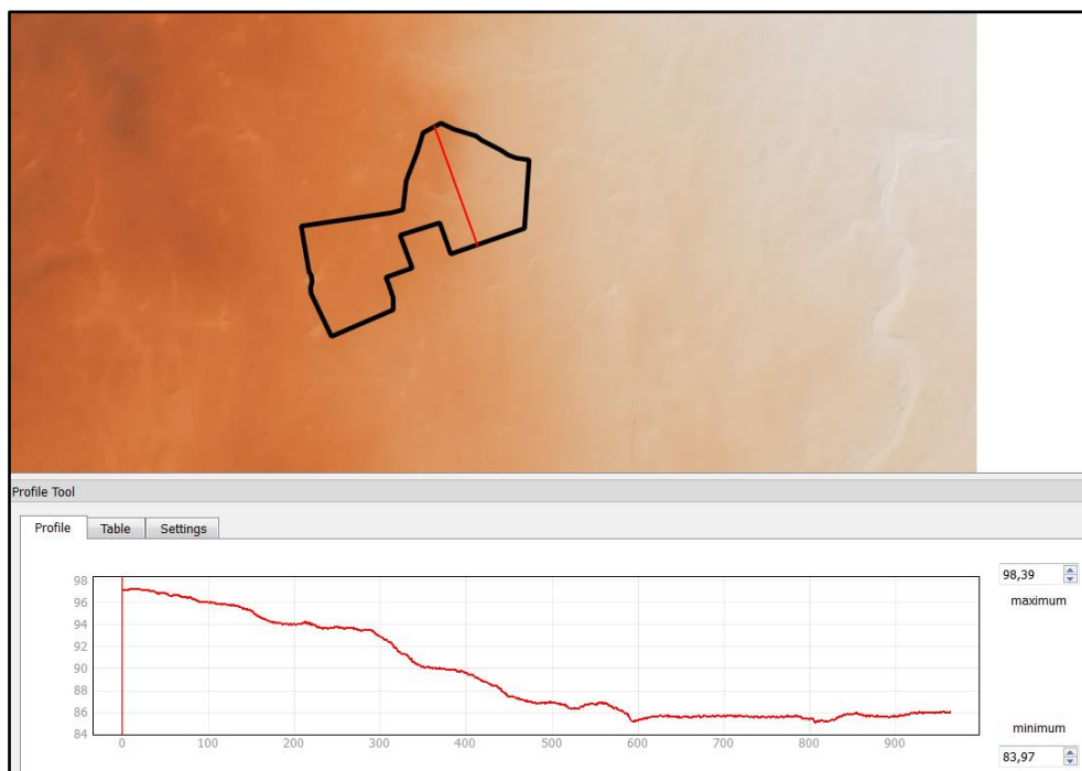
FIG 6B – Andamento topografico del terreno su sezione trasversale nell'area di progetto
