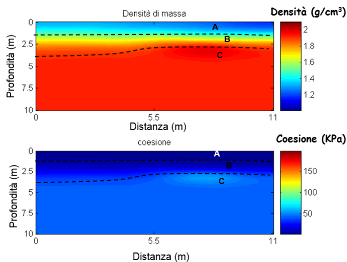
FIG.18 - Modello di distribuzione della densità di massa e della coesione a varie profondità
