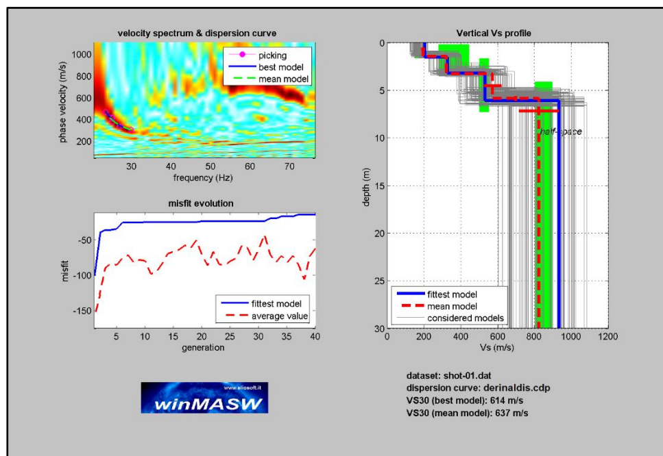
FIG.20 - Curva di dispersione con profilo verticale della velocità V_s al variare della profondità.
