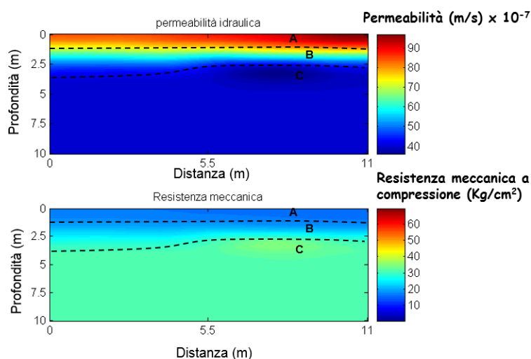
FIG. 19 - Modello di distribuzione della permeabilità e resistenza meccanica a compressione a varie profondità.
