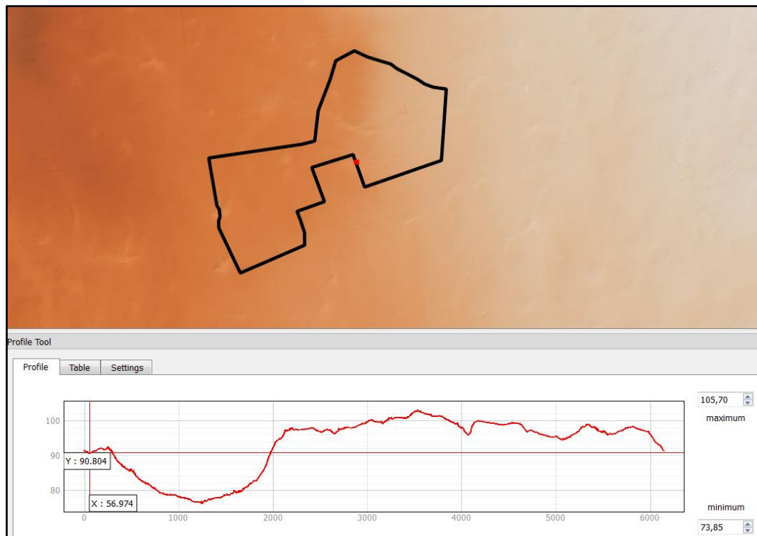
FIG 6C – Andamento topografico del terreno lungo il perimetro dell'area di progetto
