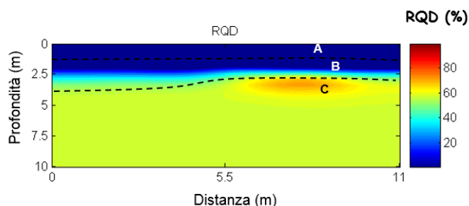
FIG.17 - Modello di distribuzione di RQD a varie profondità
