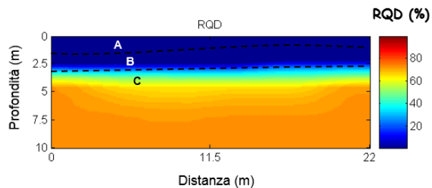
FIG.23 - Modello di distribuzione di RQD a varie profondità.
