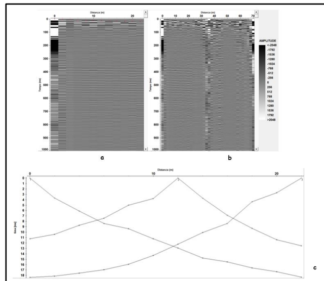
FIG. 21 - a) sismogrammi delle 3 energizzazioni; b) esempio di picking dei primi arrivi; c) Dromocrone relative al profilo sismico.
