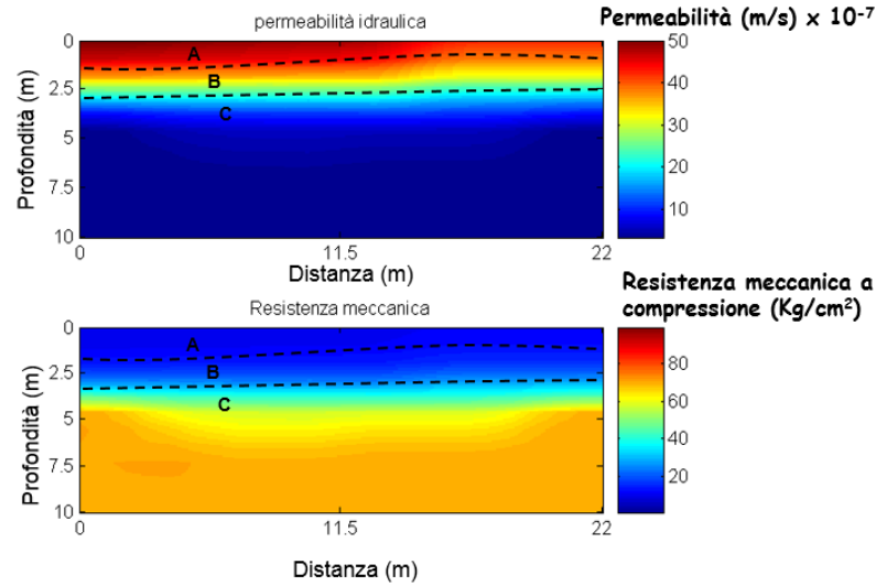
FIG. 25 - Modello di distribuzione della permeabilità e resistenza meccanica a compressione a varie profondità.
