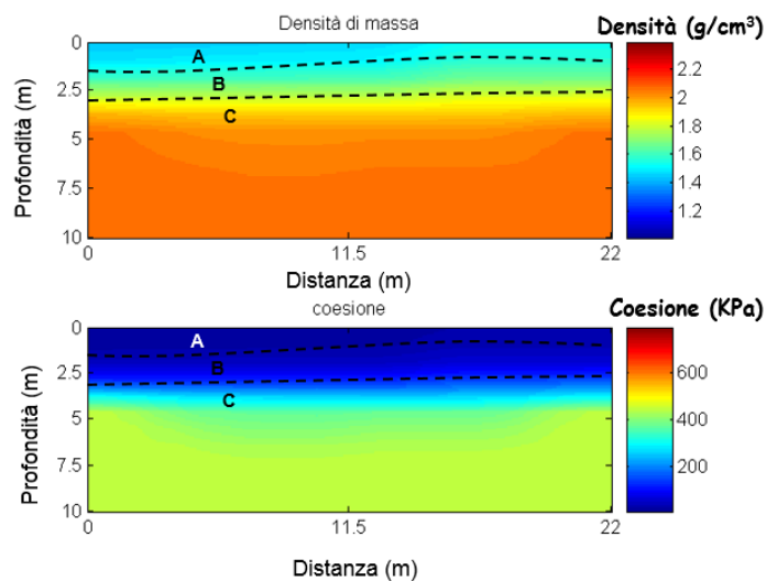
FIG.24 - Modello di distribuzione della densità di massa e della coesione a varie profondità.
