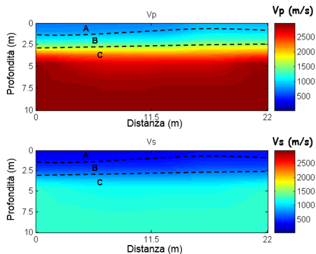
FIG.22 - Modello di distribuzione delle velocità V_p e V_s a varie profondità.
