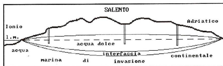
FIG 8 - Sezione idrogeologica schematica della Penisola Salentina
