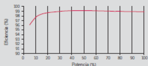
Rendimiento INGECON® SUN 160TL [600 Vac] V dc = 1.075 V
