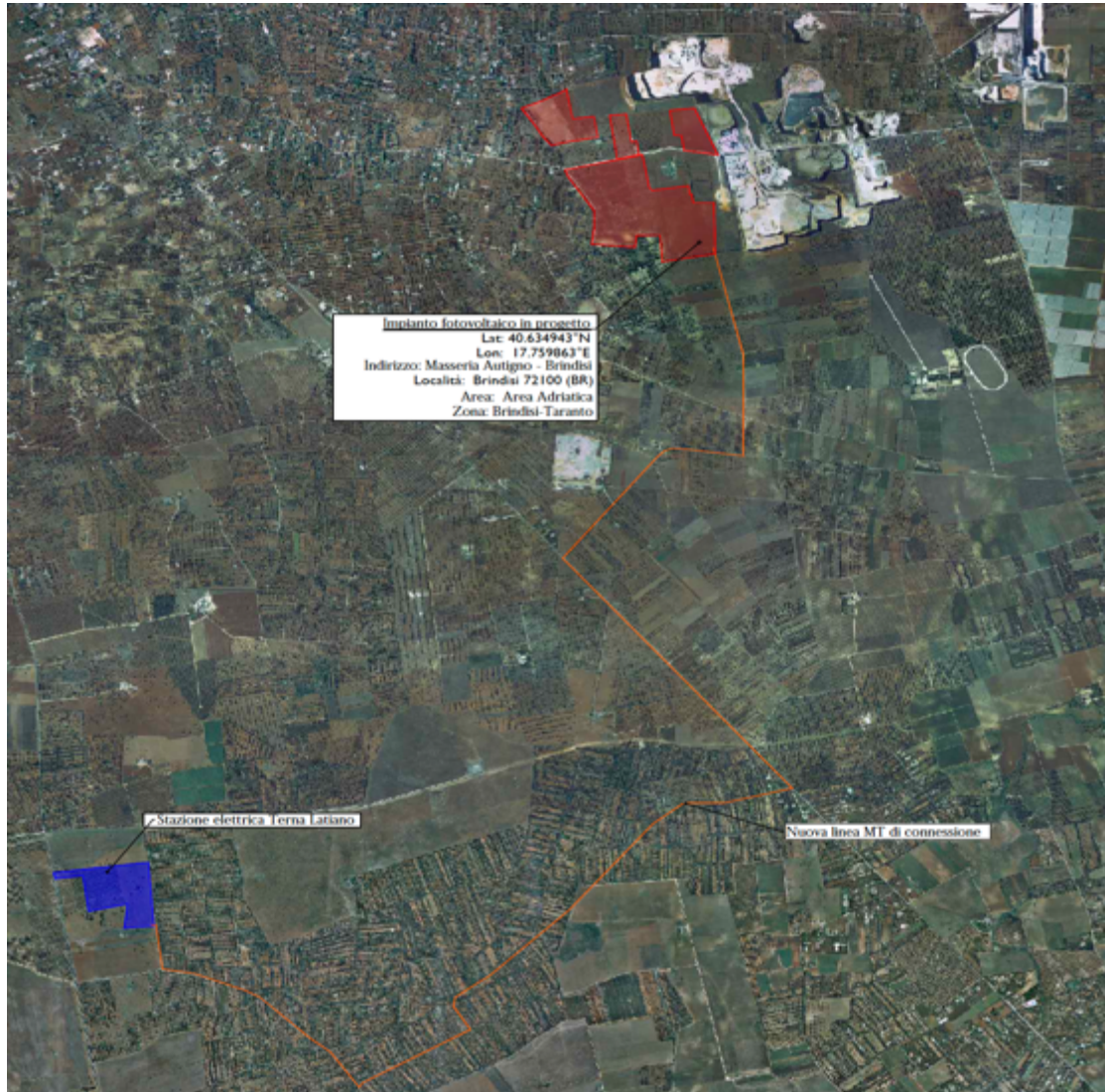
Tavola n. 5 : rappresentazione dei collegamenti previsti per l'impianto.
