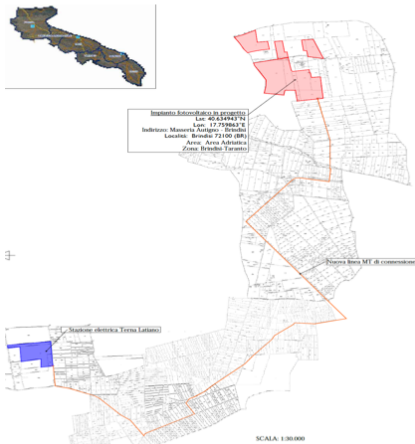
Tavola n. 2: Collegamento dell'impianto con la cabina di restituzione.
