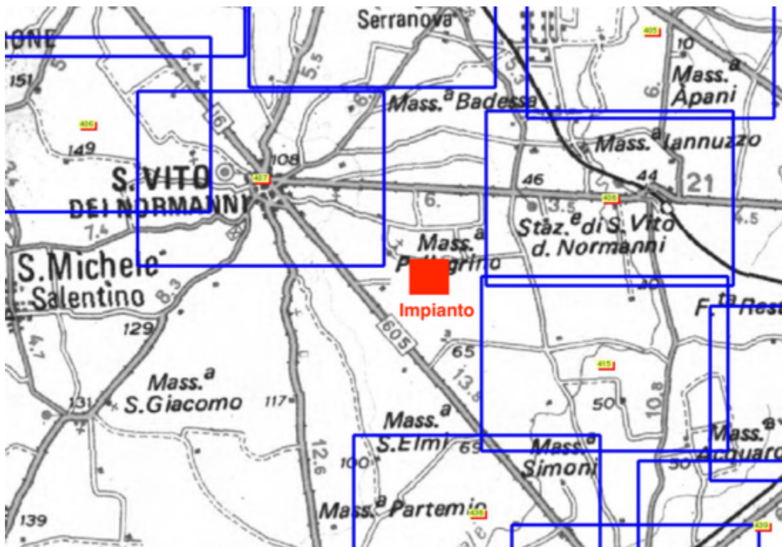
Tavola n. 3: Piano Regionale delle alluvioni. Ubicazione impianto
