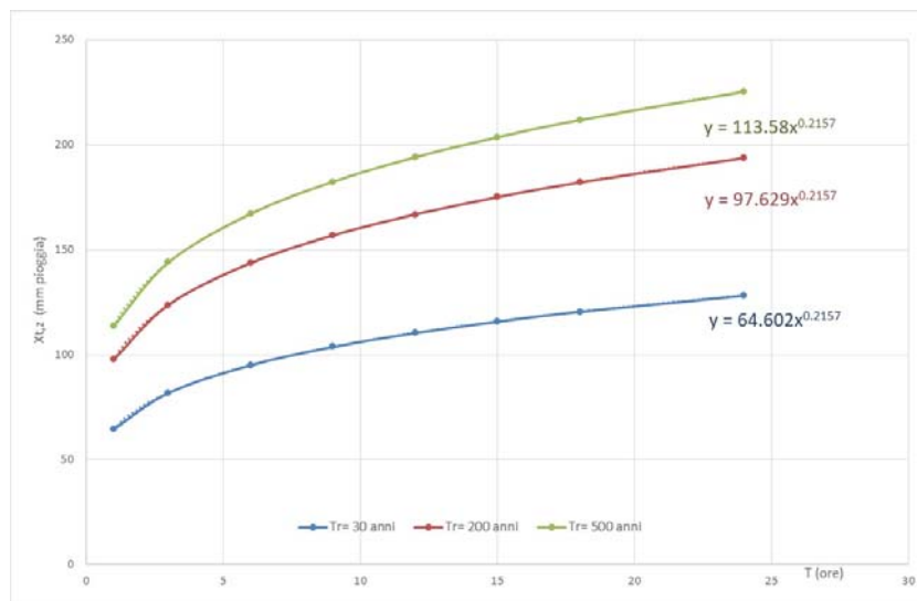
Grafico 2 - Curve di possibilità pluviometrica per Tr 30, 200 e 500 – Bacino 2
