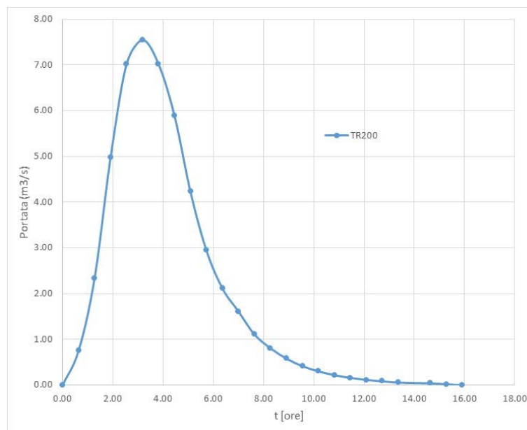
Grafico 10 - Idrogramma di Mockus TR200 – Bacino A
