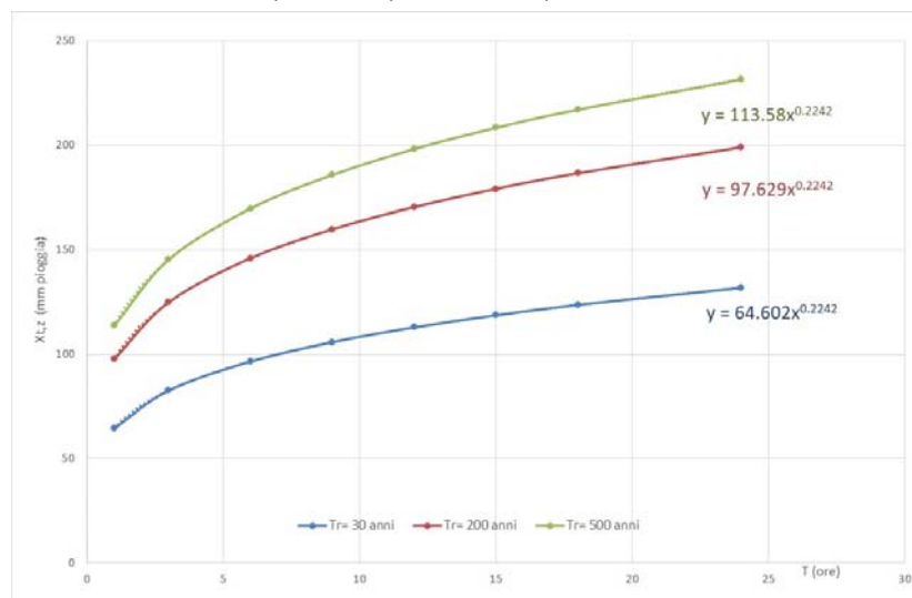
Grafico 5 - Curve di possibilità pluviometrica per Tr 30, 200 e 500 – Bacino B
