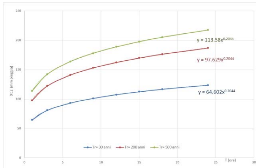
Grafico 4 - Curve di possibilità pluviometrica per Tr 30, 200 e 500 – Bacino A
