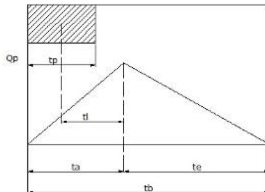
Grafico 6 - Idrogramma di Mockus
