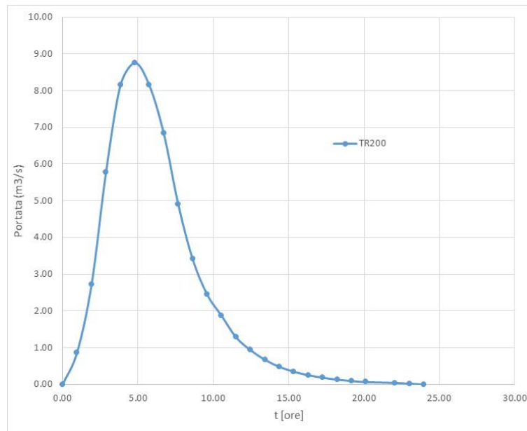
Grafico 9 - Idrogramma di Mockus TR200 – Bacino 3
