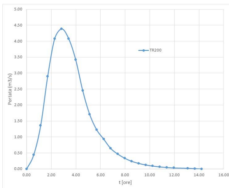
Grafico 7 - Idrogramma di Mockus TR200 – Bacino 1
