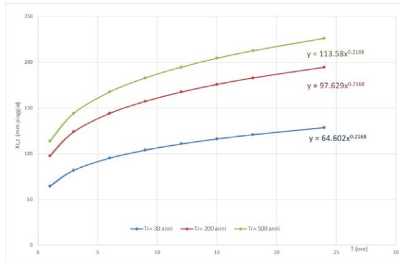
Grafico 3 - Curve di possibilità pluviometrica per Tr 30, 200 e 500 – Bacino 3
