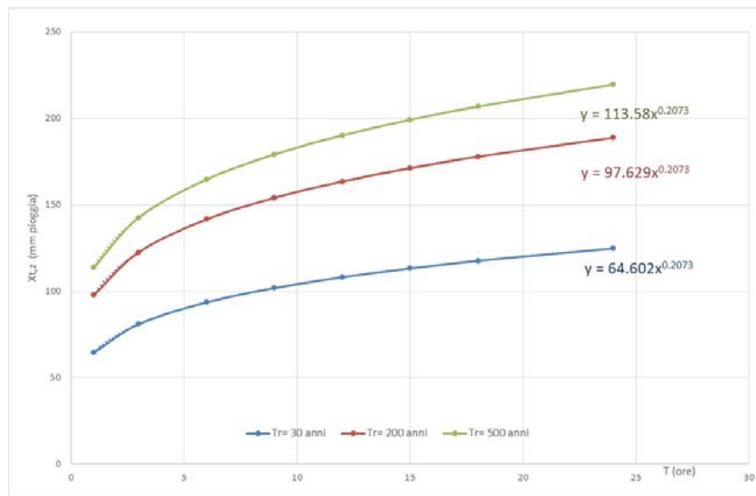
Grafico 1 - Curve di possibilità pluviometrica per Tr 30, 200 e 500 – Bacino 1
