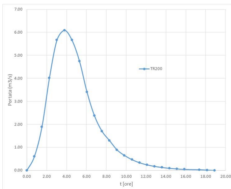
Grafico 8 - Idrogramma di Mockus TR200 – Bacino 2
