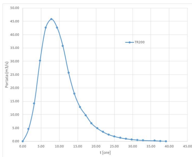
Grafico 11 - Idrogramma di Mockus TR200 – Bacino B
