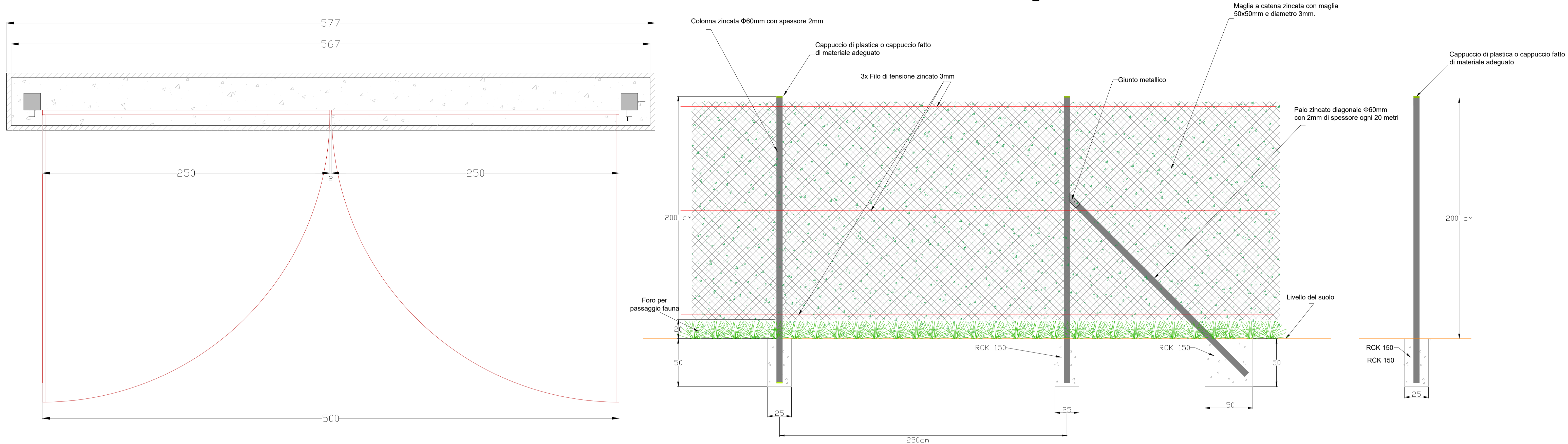
5.00 M CANCELLI PER PORTE ANTE DOPPIE VISUALIZZAZIONE DEL PIANO
