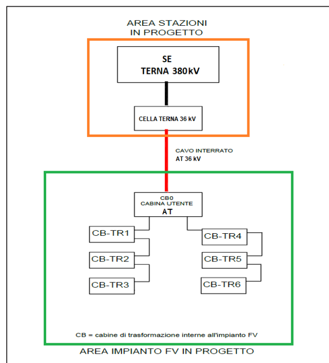
FIGURA 5: SCHEMA A BLOCCHI IMPIANTO
