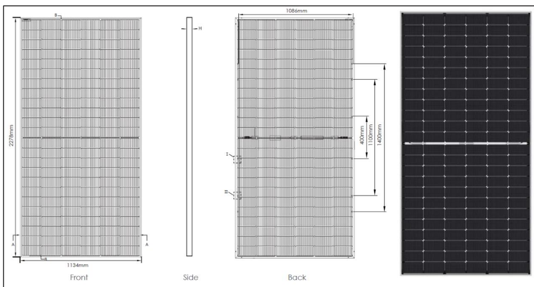
FIGURA 6: PANNELLO FV PARI A 570 WP CON DIMENSIONI 2278 x 1134 x 30 MM
