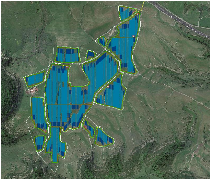
FIGURA 4: LAYOUT D' IMPIANTO
