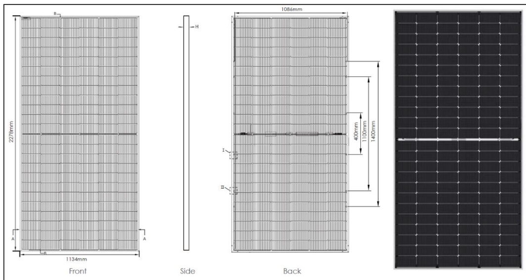
FIGURA 5: PANNELLO FV PARI A 570 WP CON DIMENSIONI 2278 X 1134 X 30 MM
