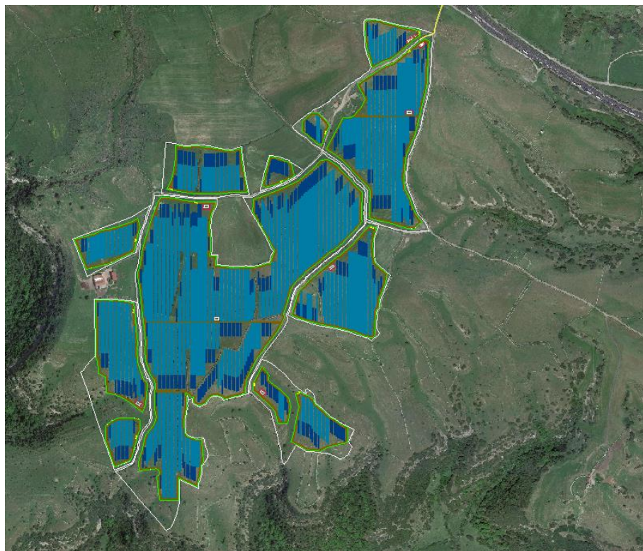
FIGURA 1: LAYOUT D' IMPIANTO
