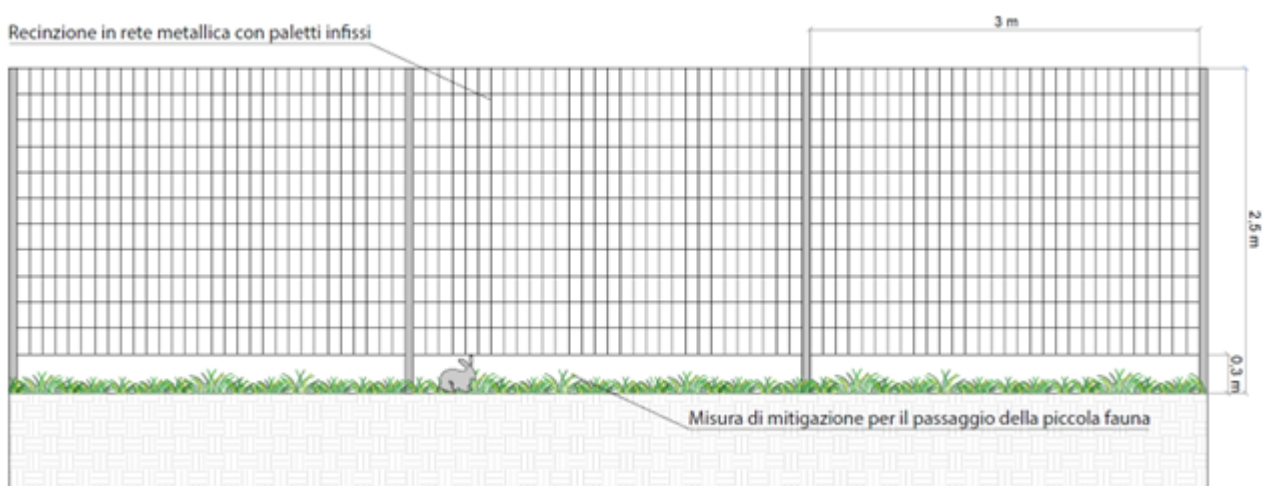
FIGURA 18: RECINZIONE TIPO
