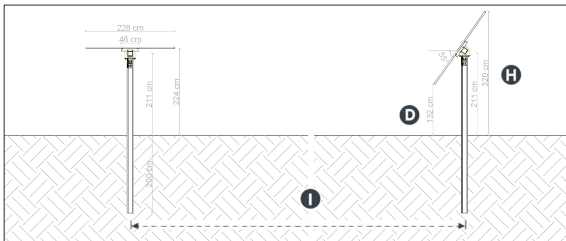
FIGURA 3: DEFINIZIONE DELLE DIMENSIONI DEI TRACKER
