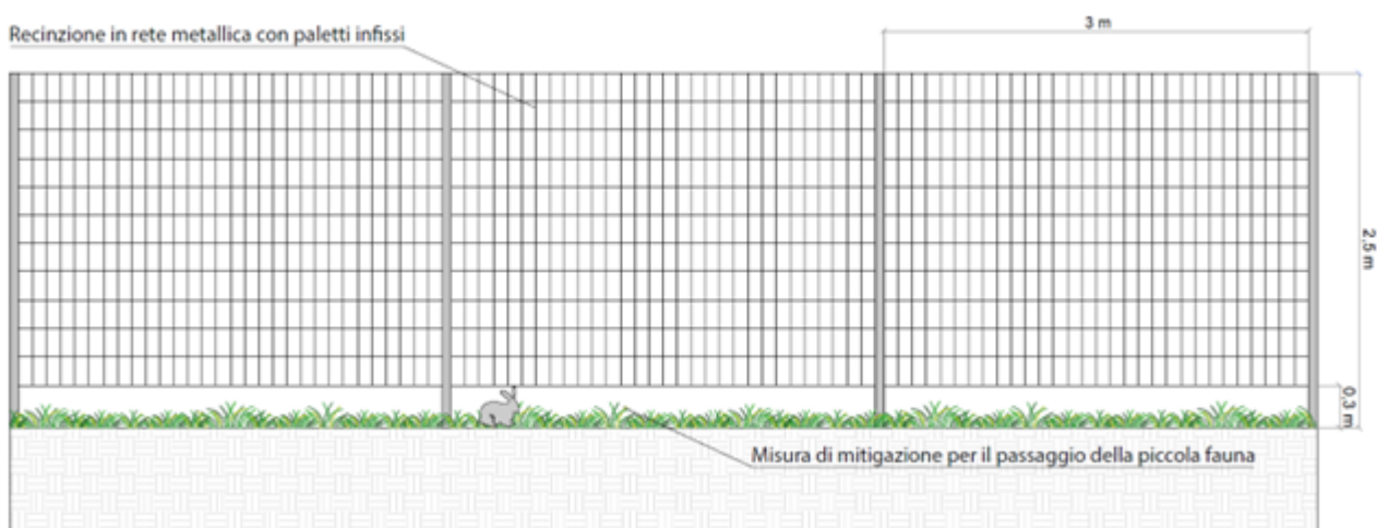
FIGURA 9: RECINZIONE TIPO
