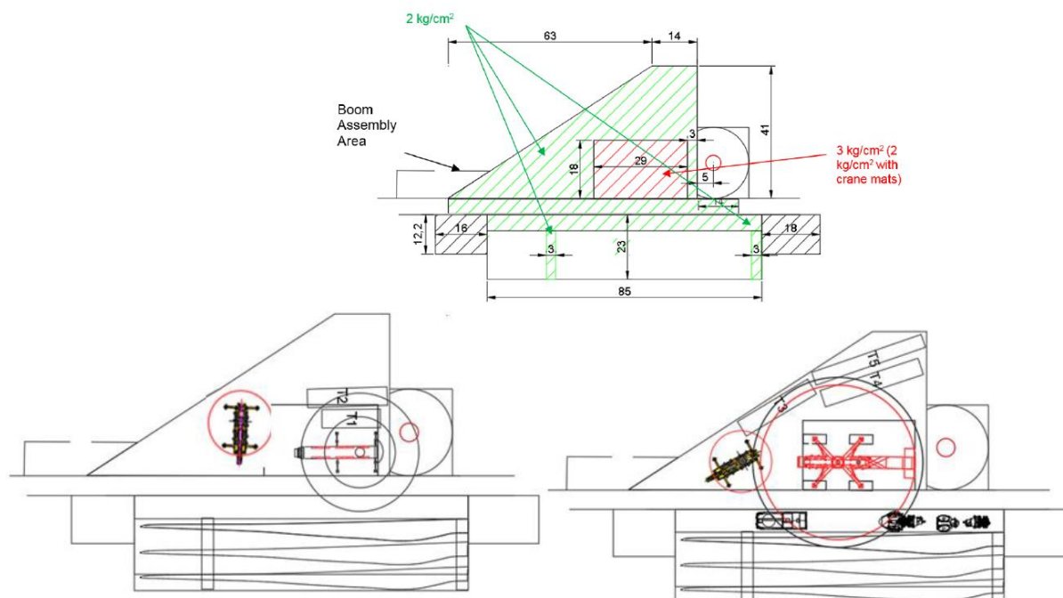
Figura 4.2 – tipologico per il sistema di montaggio “Partial storage”
