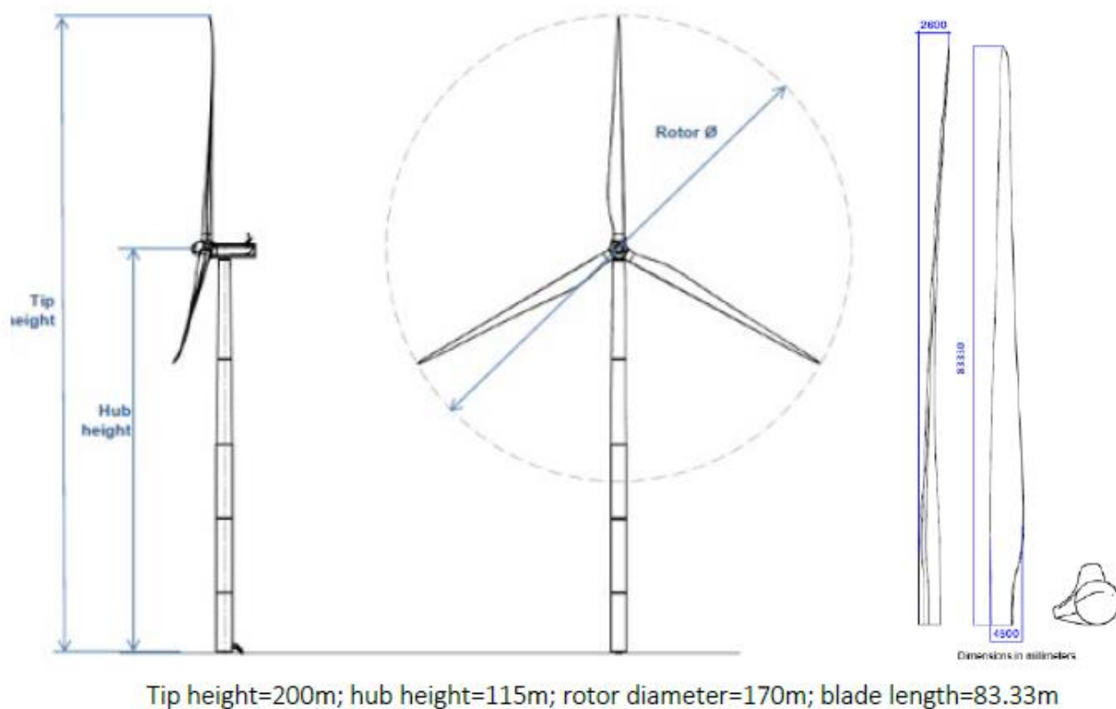
Figura 4.1: Struttura aerogeneratore
