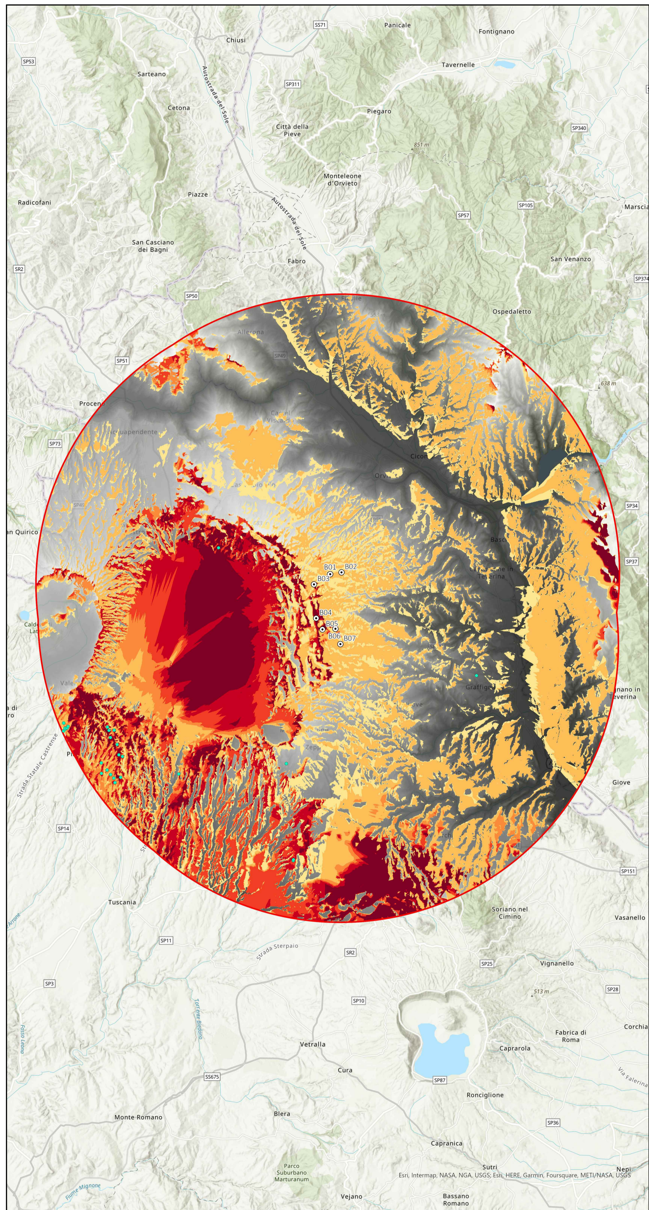
CARTA DELL'INTERVISIBILITA' TEORICA CUMULATA ALL'INTERNO DELL'AP
