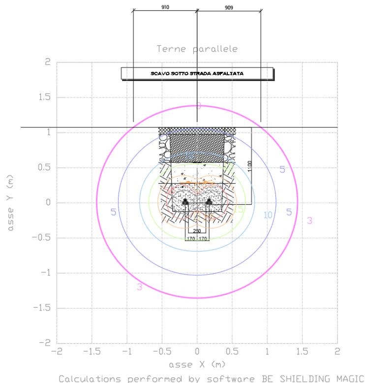
Figura 1 – Livelli di campo magnetico per il cavidotto MT 30kV
