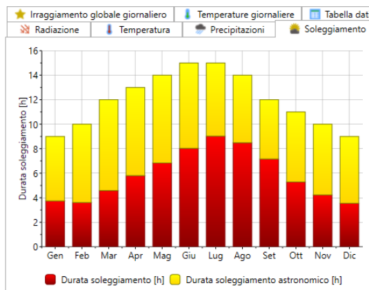
Fig. 27 – Dati di radiazione, temperatura, precipitazioni e soleggiamento (Riferiti al sito di Palata)
