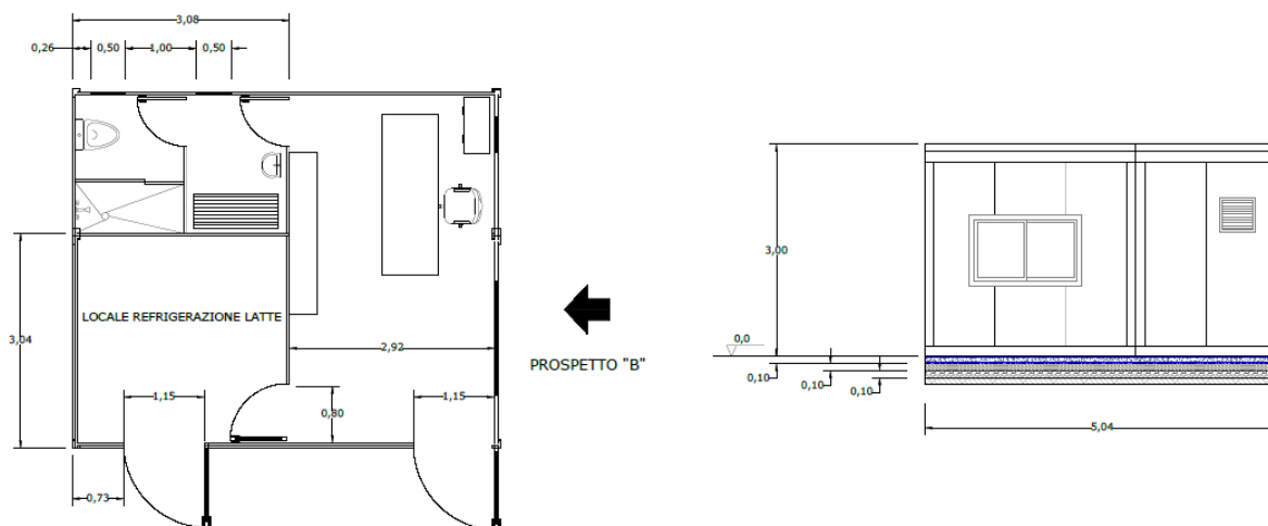
Fig. 23 – Ufficio/Locale tecnico
