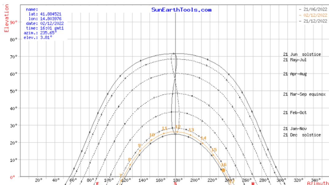
Fig. 29 - Diagramma Solare Polare (Palata)
