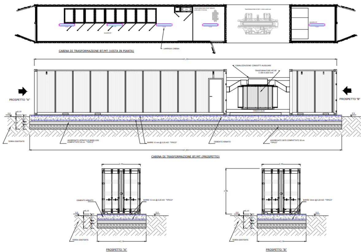
Fig. 18 - Cabina di trasformazione BT/MT
