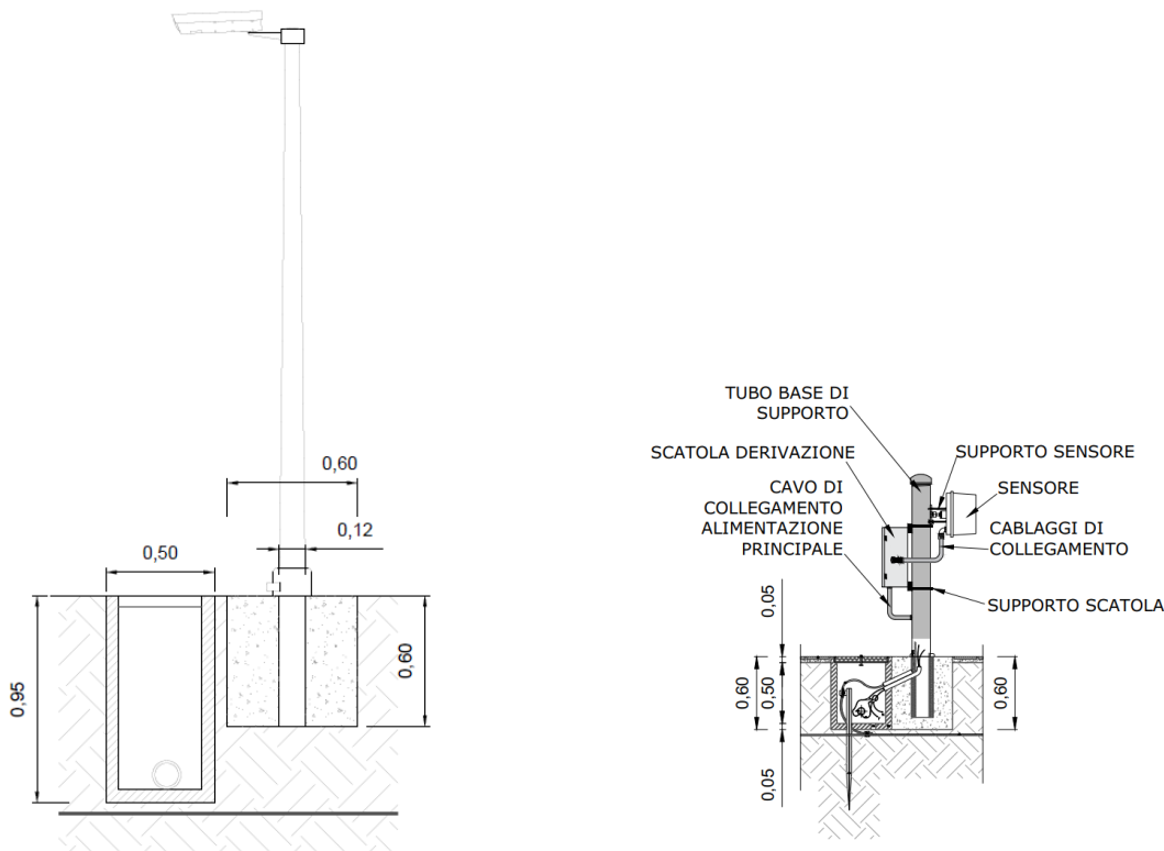
Fig. 25 – Sistema antintrusione
