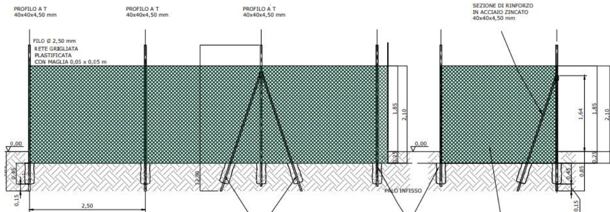
Fig. 14 – Recinzione perimetrale
