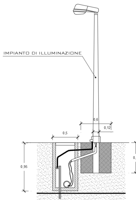
Fig. 26 – Sistema di illuminazione
