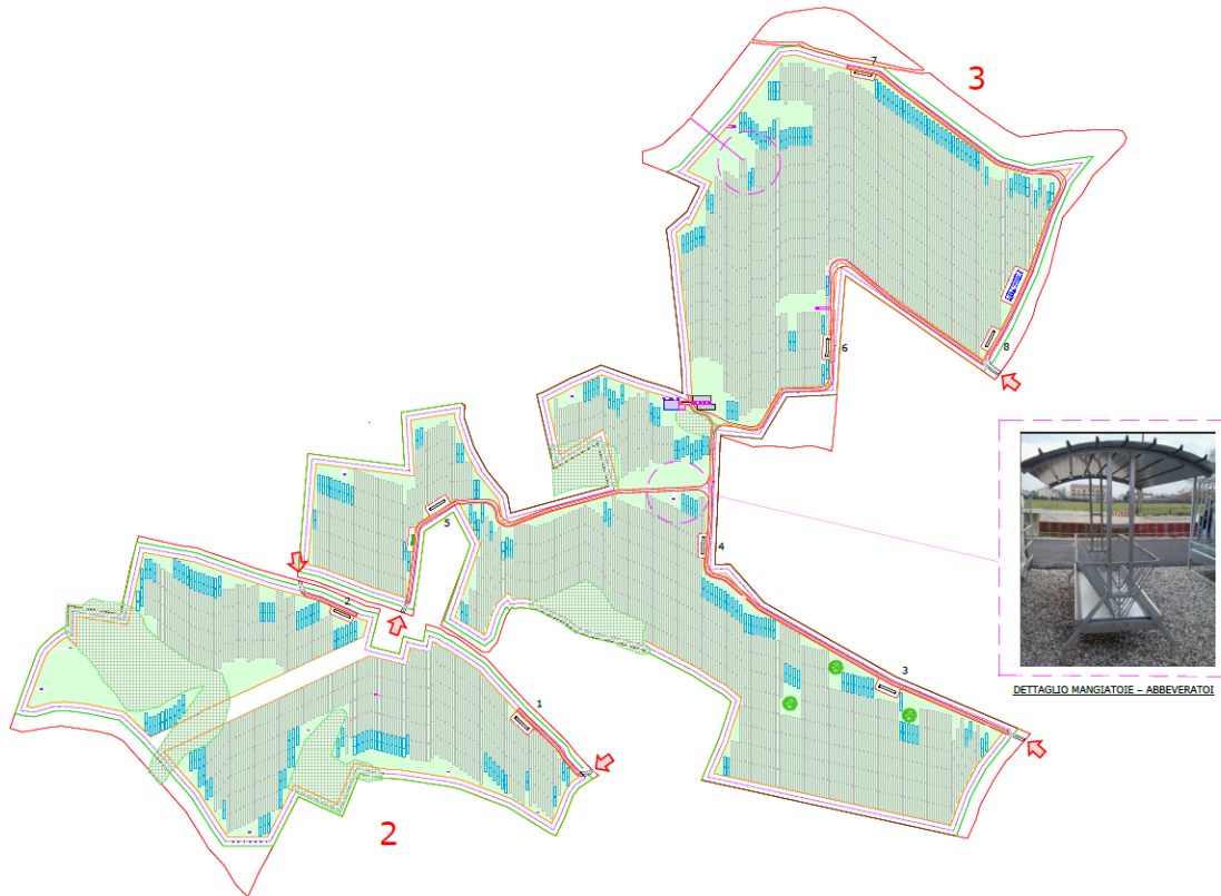
Fig. 3 – Esempio di “area di impianto” ovivoltaico
