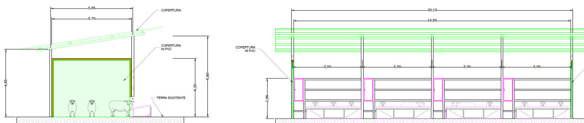
Fig. 21 – Esempio di struttura di ricovero ovini
