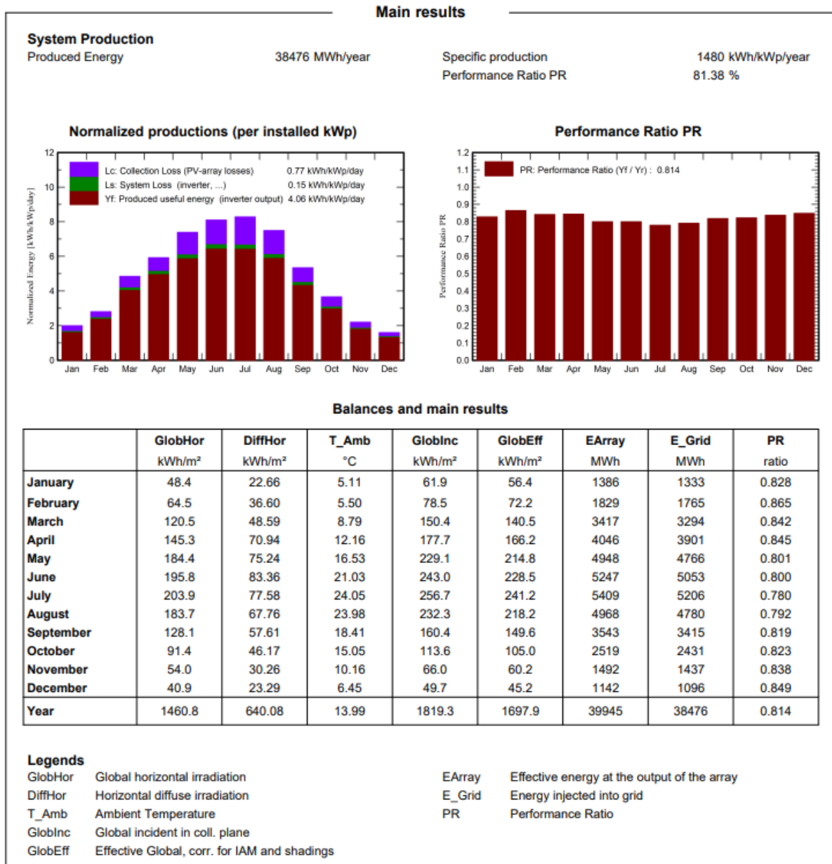
Fig. 30 - Risultati di calcolo (Fonte: PVsyst - Meteonorm)
