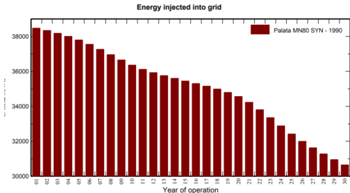
Fig. 31 – Producibilità dell'impianto con degrado moduli (30 anni)
