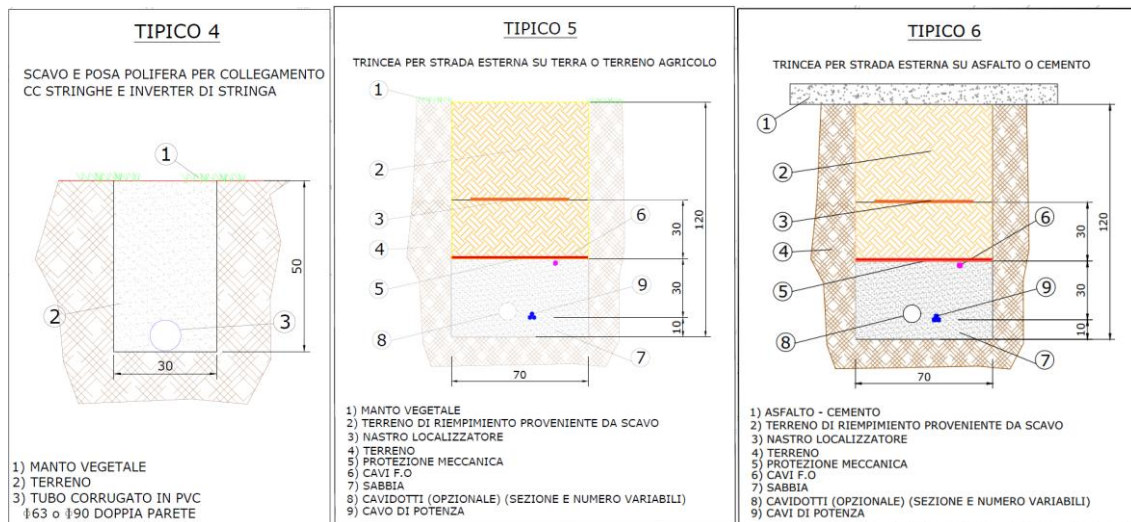
Fig. 17 – Tipici scavi e posa cavi
