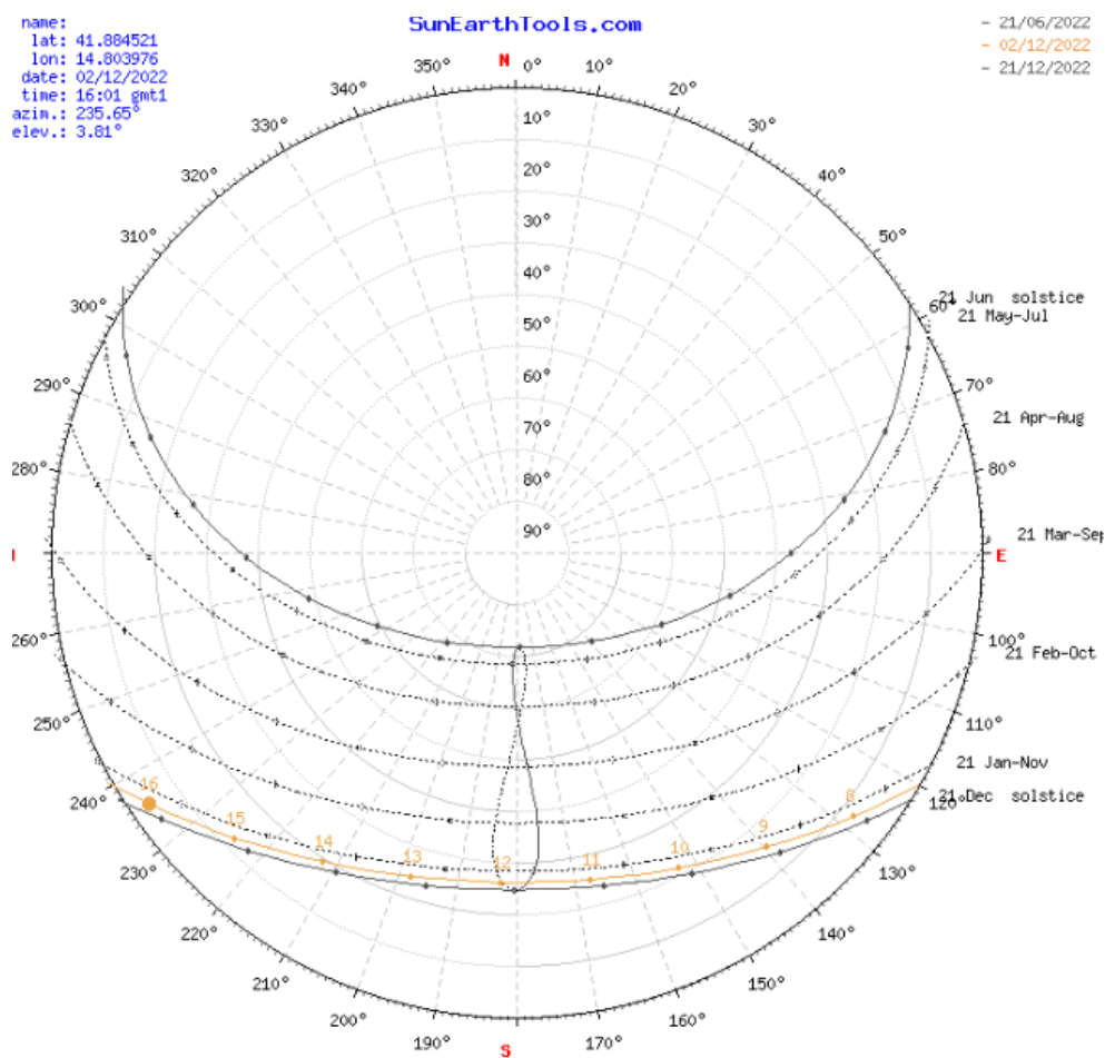
Fig. 28 - Diagramma Solare Polare (Palata)
