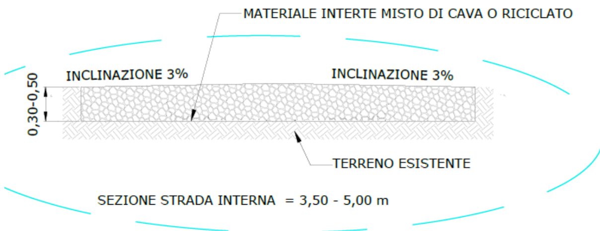
Fig. 16 – Viabilità interna
