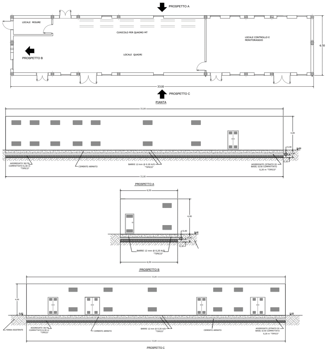
Fig. 19 - Cabina di ricezione
