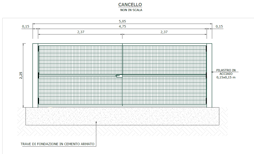
Fig. 15 – Cannello a doppia anta
