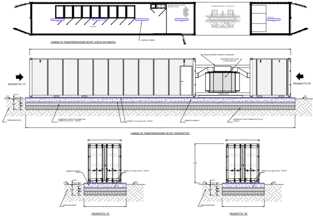
Fig. 12 - Cabina di trasformazione BT/MT
