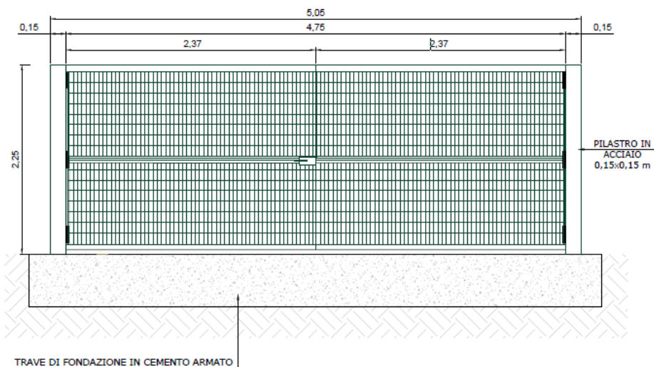
Fig. 17 – Cancellò carrabile
