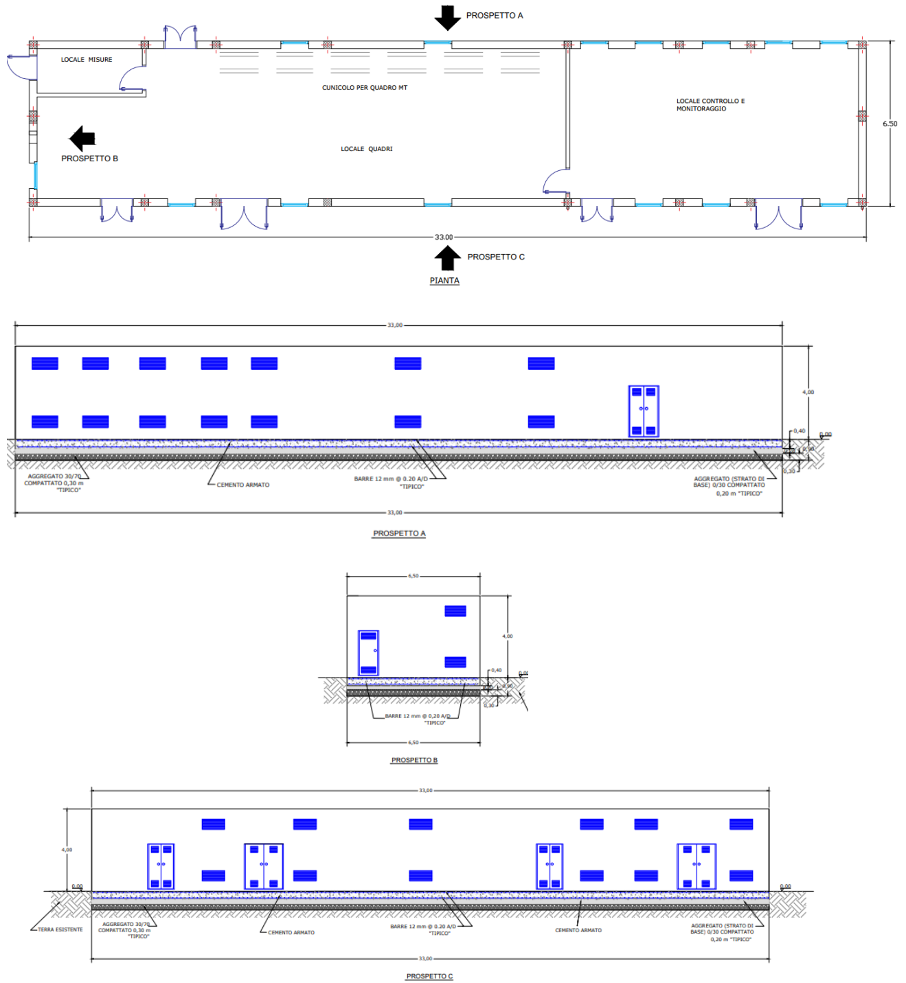
Fig. 13 - Cabina di ricezione
