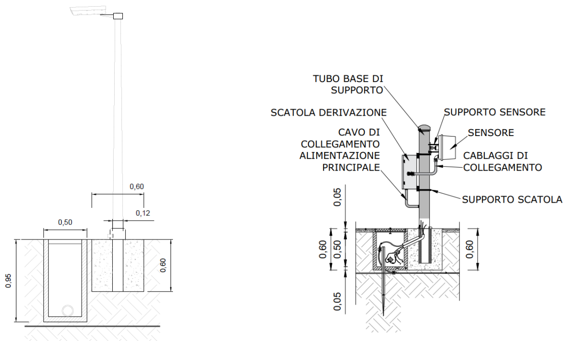
Fig. 19 – Sistema antintrusione
