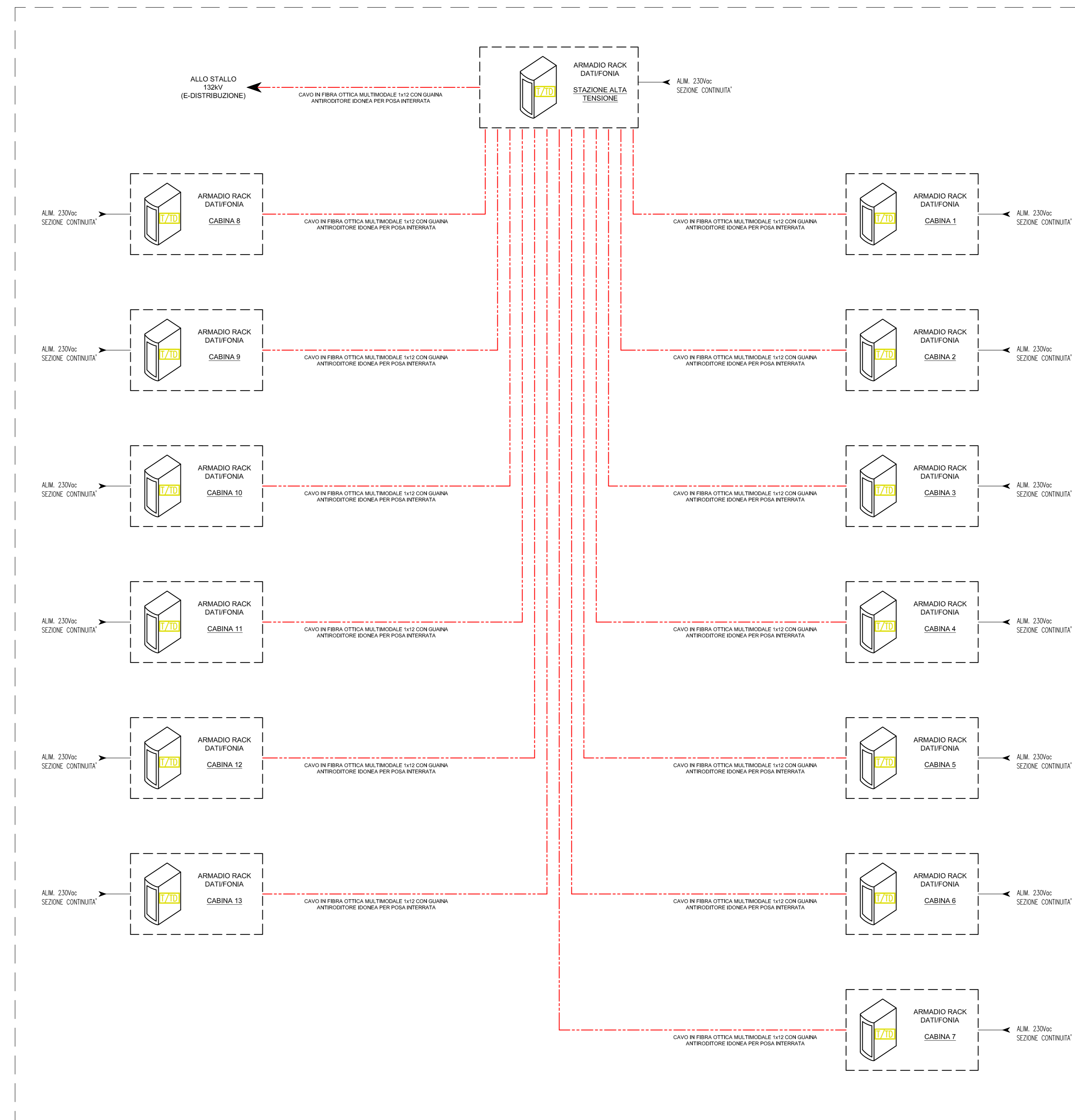
SCHEMA A BLOCCHI RETE TRASMISSIONE DATI
