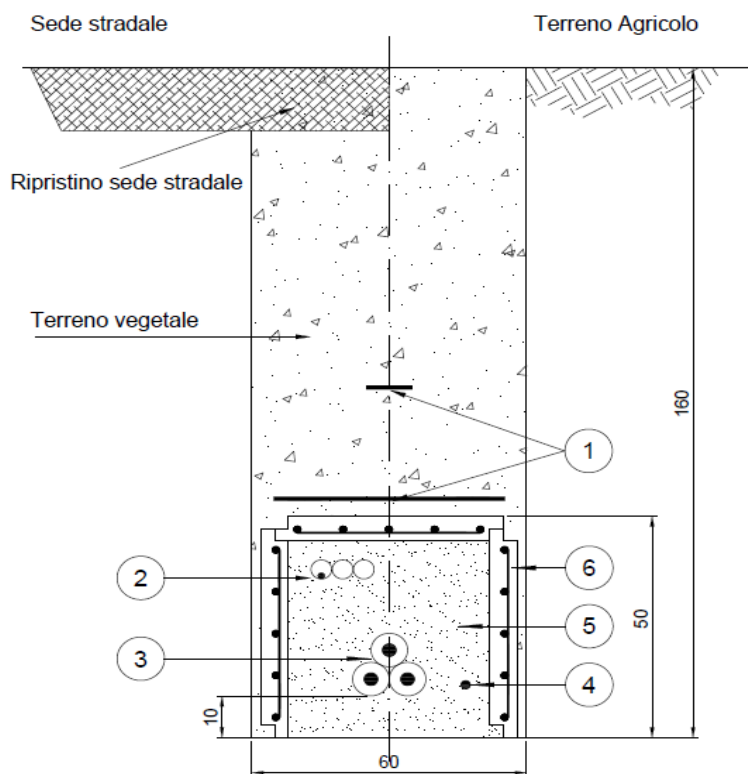
Figura 6: Sezione tipo - linea cavi 132 kV in cavi sotterranei unipolari, sezione trasversale di posa a trifoglio
