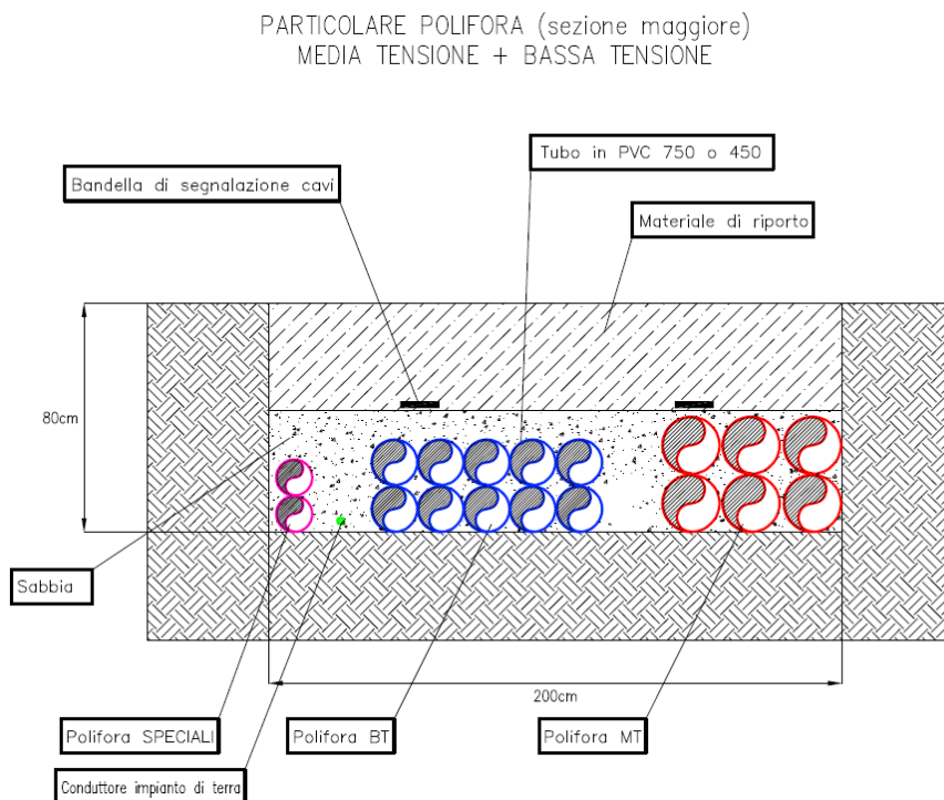
Figura 3: Sezione tipo di posa
