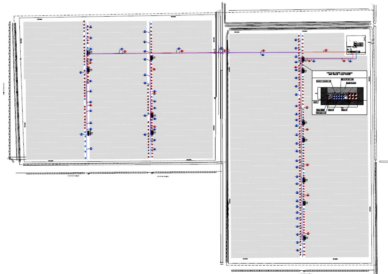
Figura 2: Traccia cavi BT e MT, con sezione tipo di scavo
