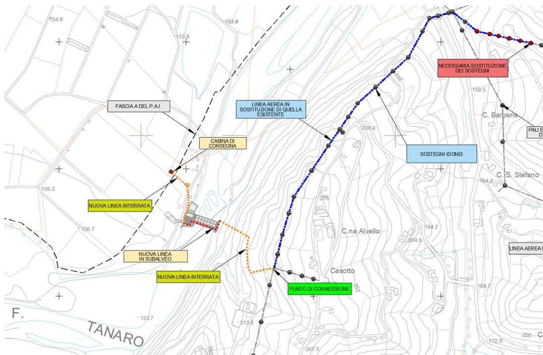
Figura 11 – Estratto della planimetria della connessione alla rete
