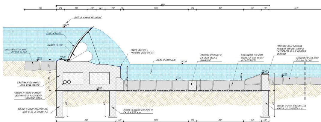
Figura 3 – Traversa in progetto
