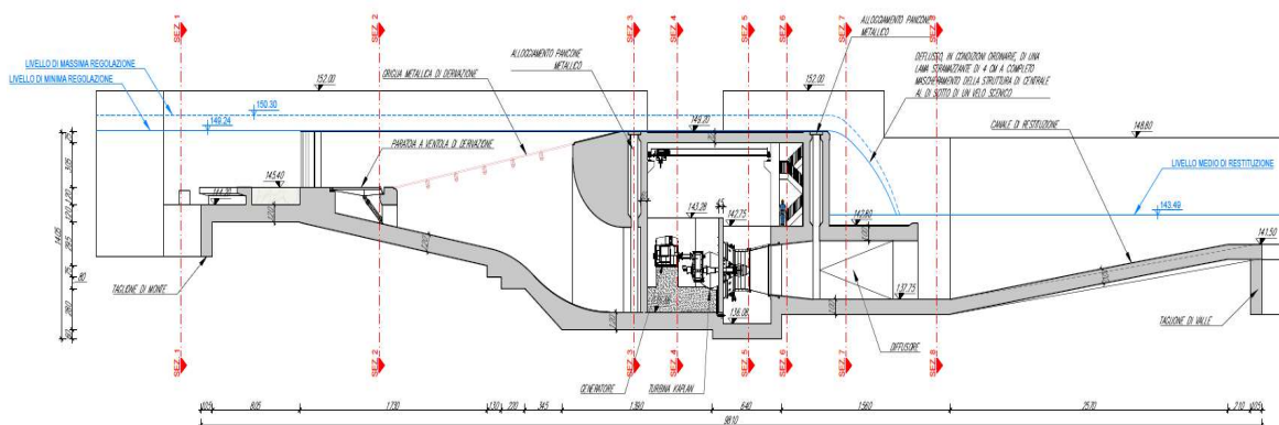
Figura 9 – Profilo di progetto dell'impianto idroelettrico
