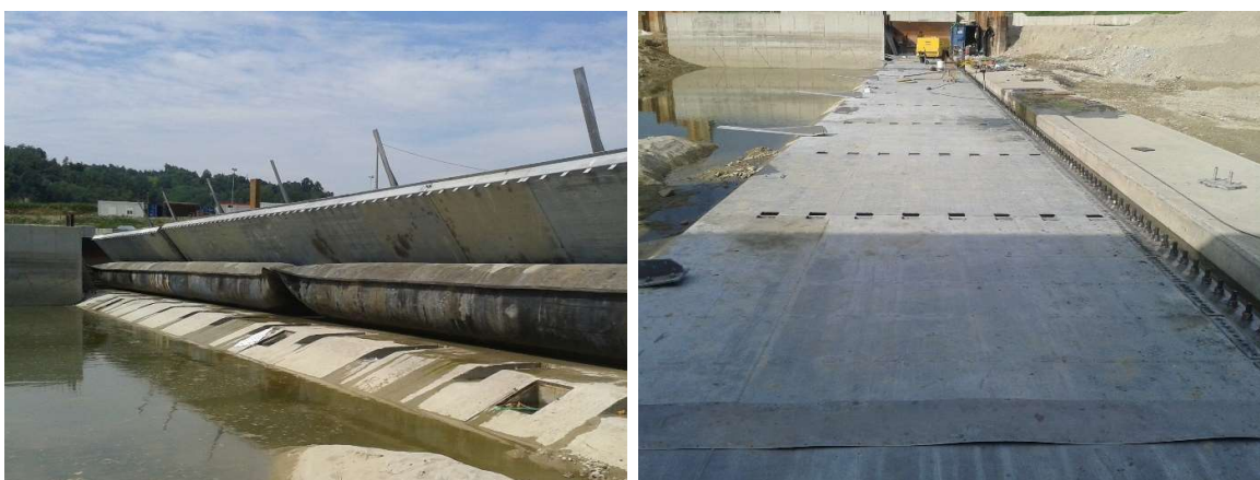
Figura 5 – Sbarramento gonfiabile scudato con singolo elemento elastomerico di gonfiaggio a valle di H=4,2 m e L=85 m analogo a quello previsto in progetto. Fasi di collaudo e gonfiaggio dell'elastomero (in sinistra) e fasi di installazione con sbarramento in posizione completamente abbattuta (in destra)
