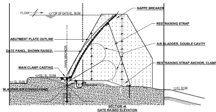
Figura 4 – Sezione tipo sopralzo abbattibile scudato
