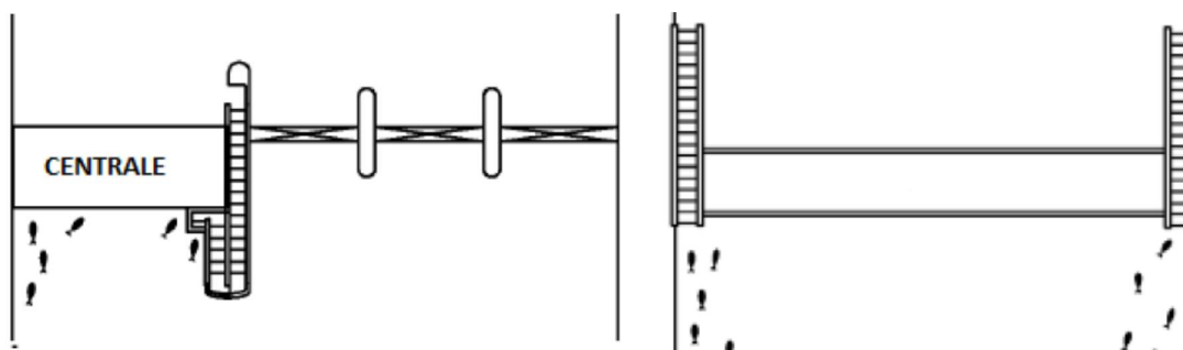
Figura 7 – Ubicazione corretta del passaggio per pesci in corrispondenza di una traversa interessata da un impianto idroelettrico e con elevata ampiezza dell'alveo. Tale configurazione è analoga a quella prevista dagli Scriventi
