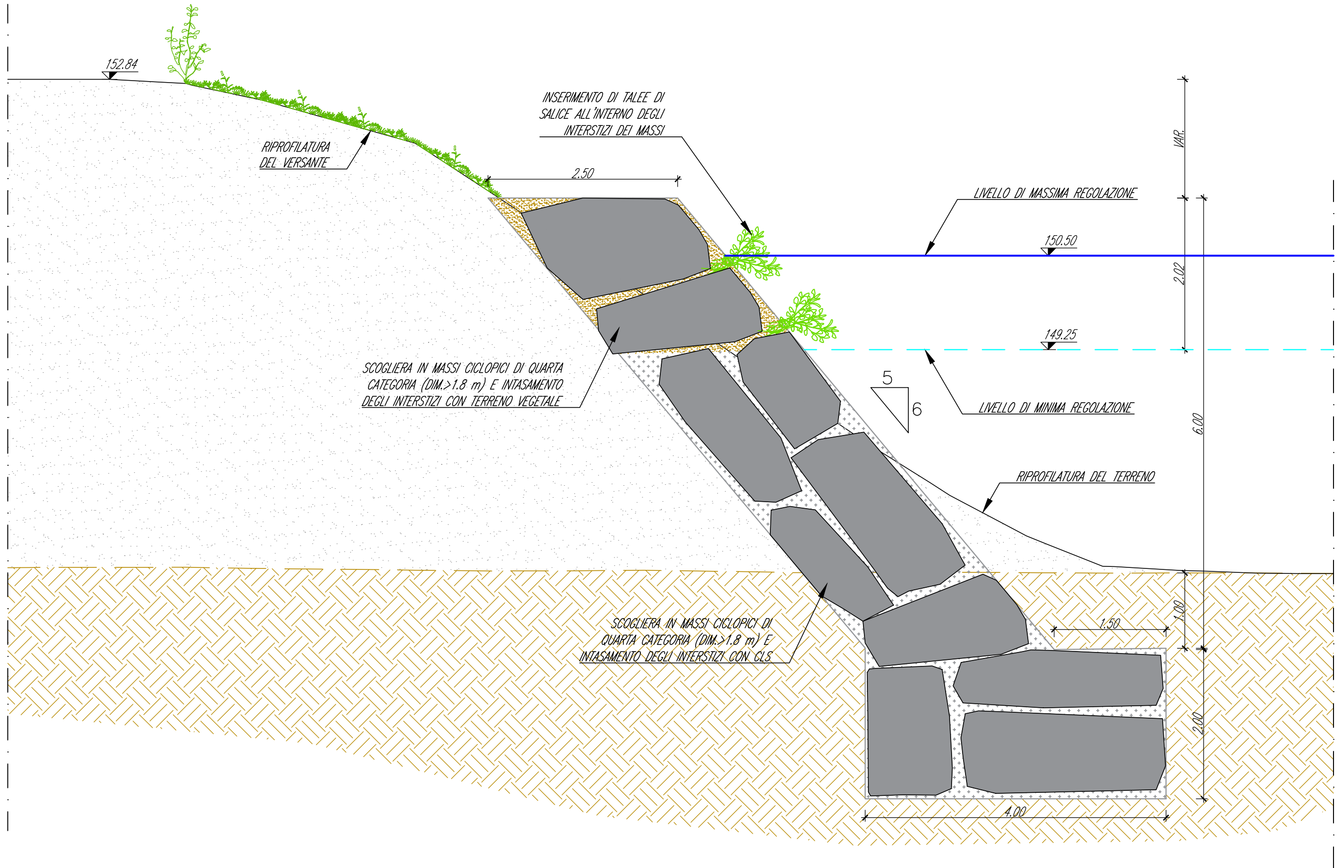
SEZIONE TIPO DELLA SCOGLIERA IN MASSI CICLOPICI Scala 1:50
