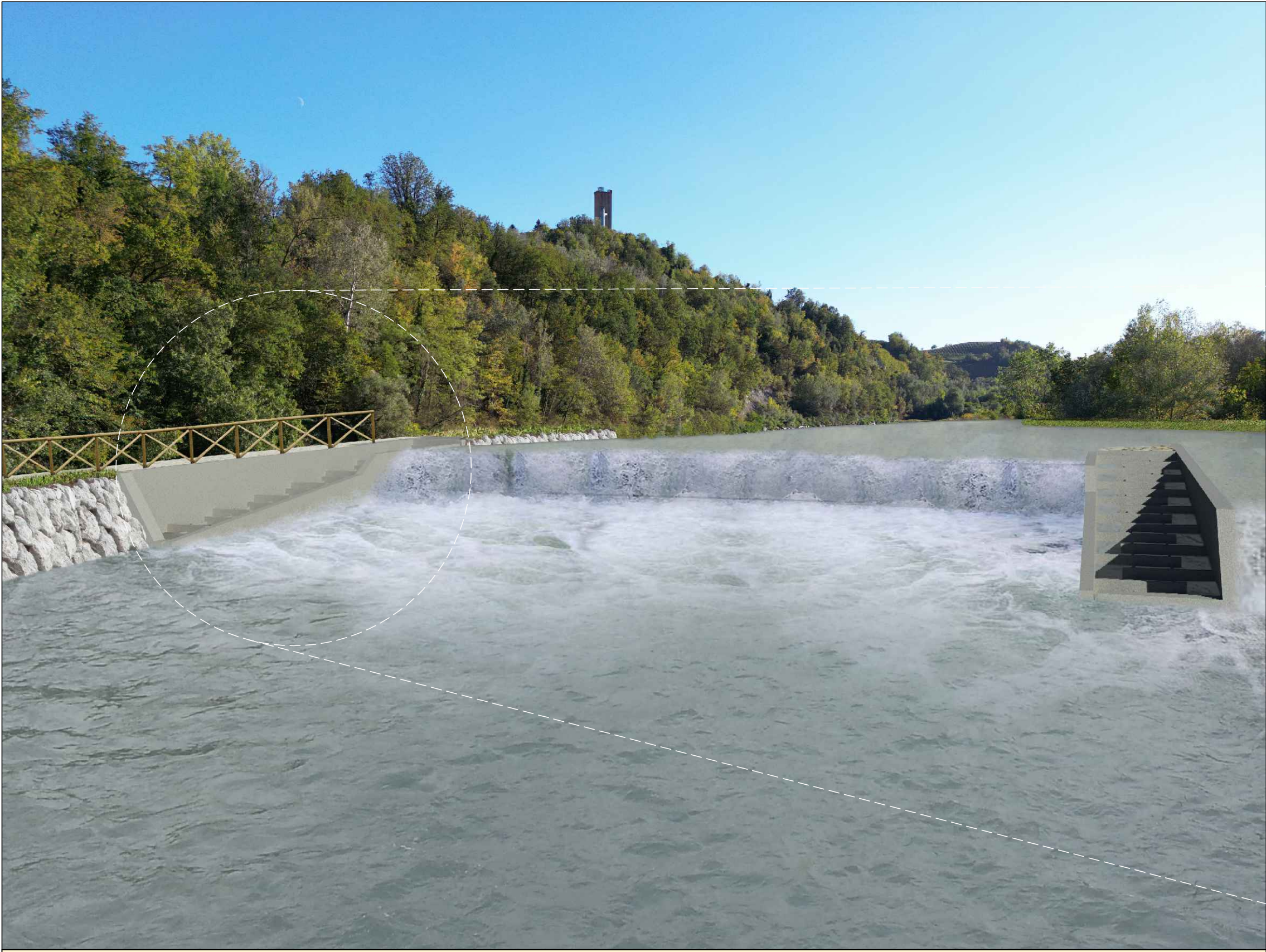
FOTOINSERIMENTO 06: VISTA DA VALLE, IN CONDIZIONI DI NORMALE REGOLAZIONE, DELL'IMPIANTO IDROELETTRICO
