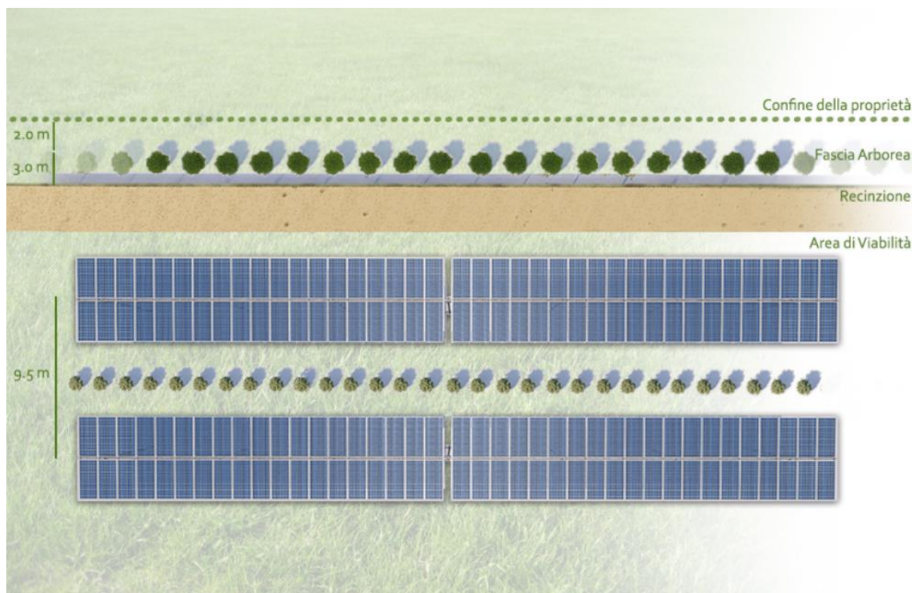
Figura 2-2: Soluzione Agro-Solare: barriera verde perimetrale, viabilità interna, tracker e componente agronomica
