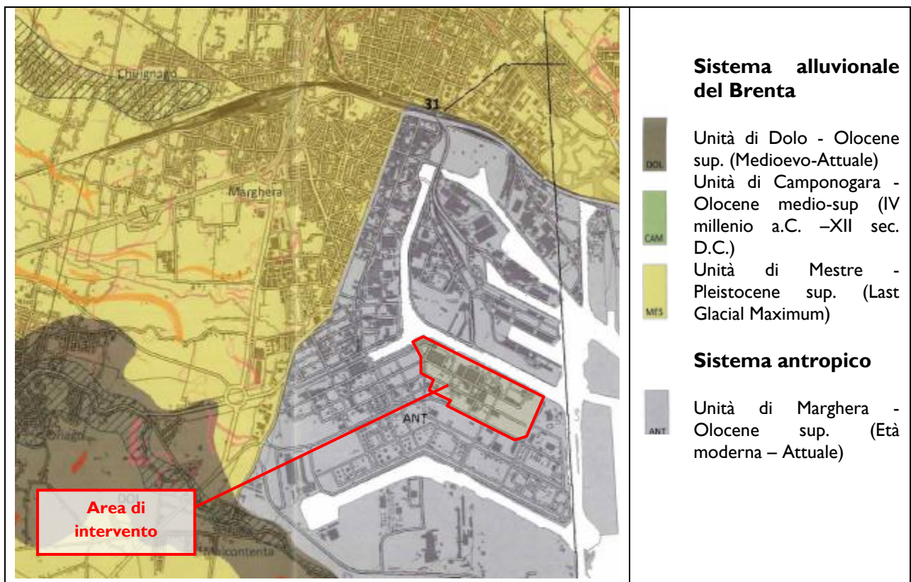
Figura 4.19. Estratto della Carta delle unità geologiche della Provincia di Venezia (2008)
