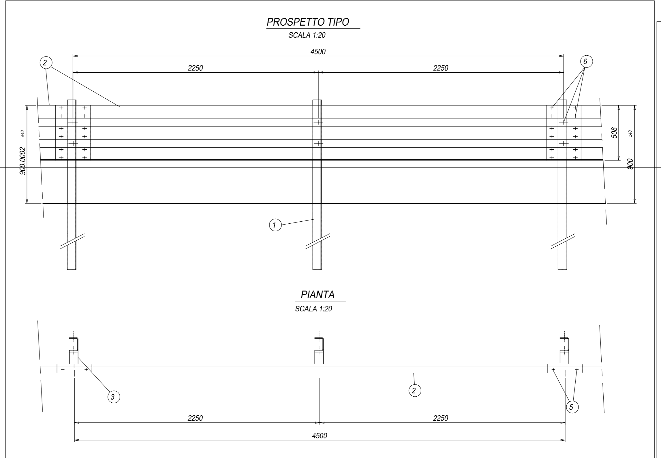
BARRIERA BORDO LATERALE DI CLASSE H2
