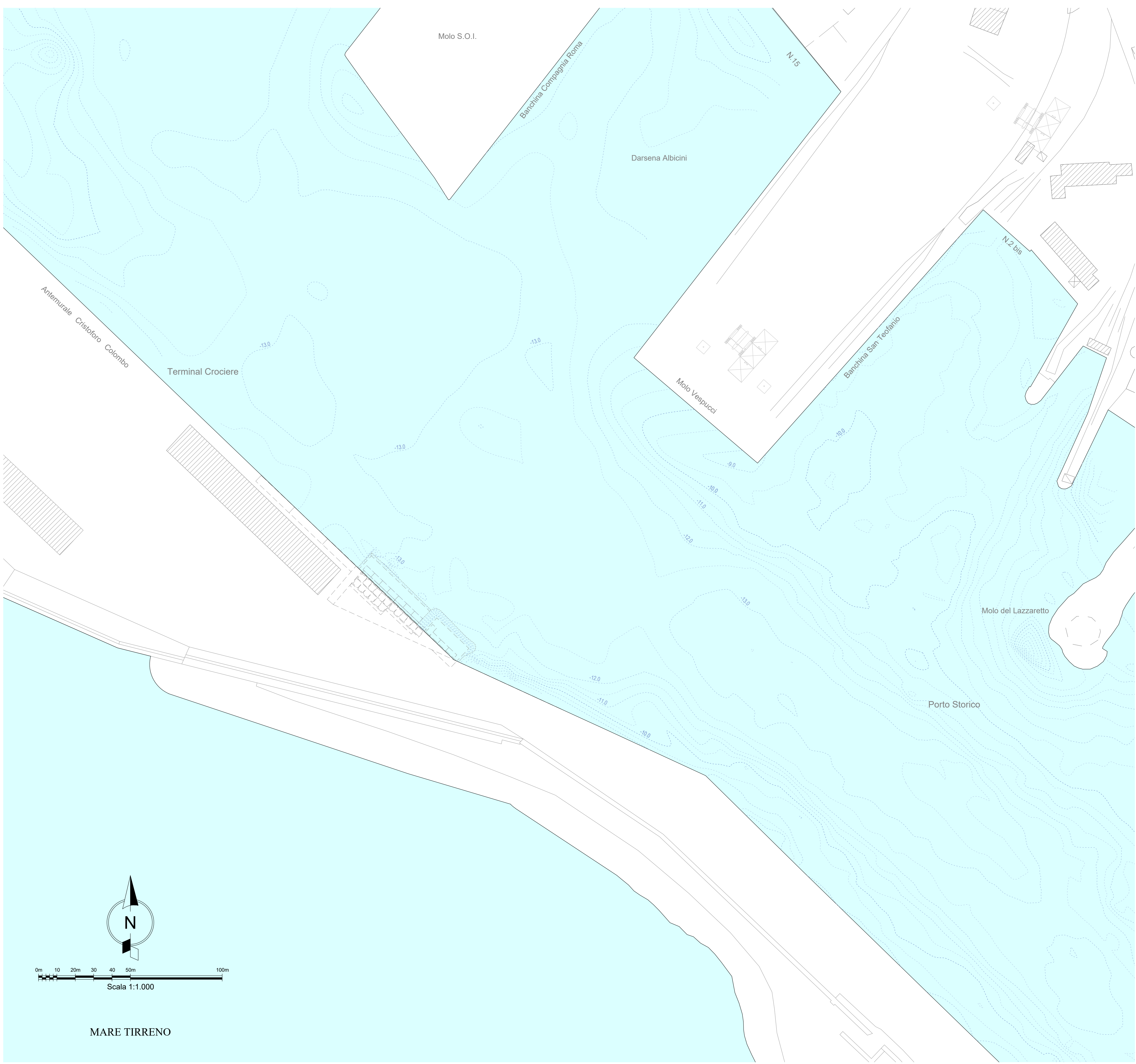
PIANTA CHIAVE
