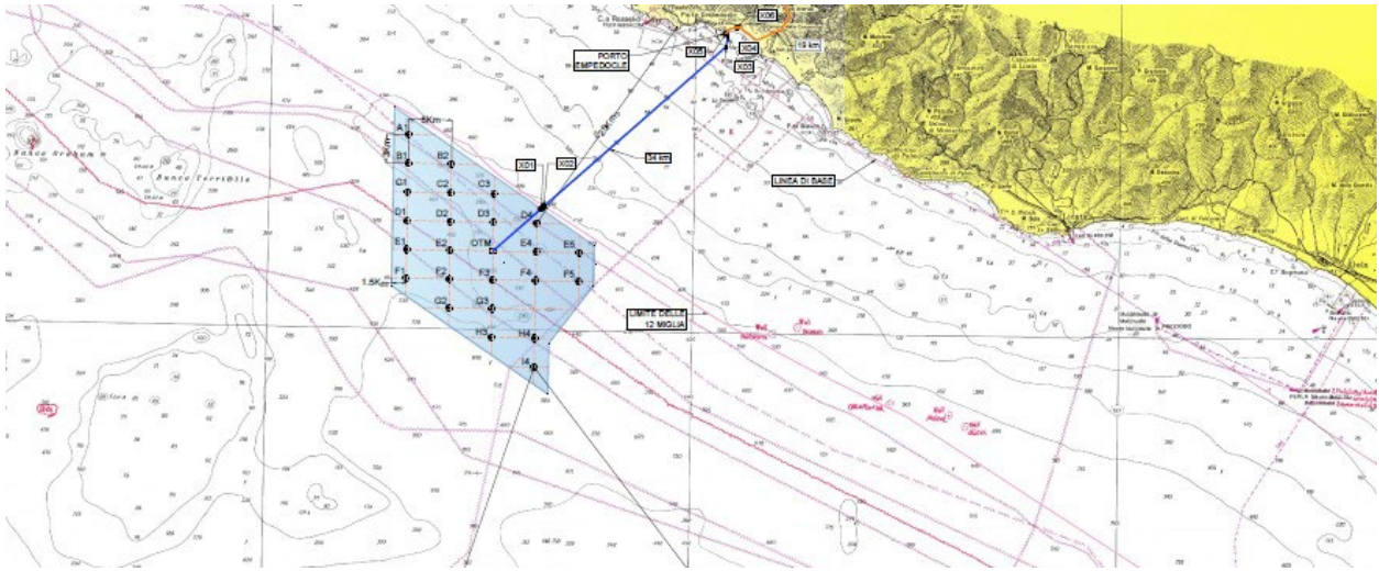
Figura 4 – Layout impianto su carta nautica di dettaglio.
