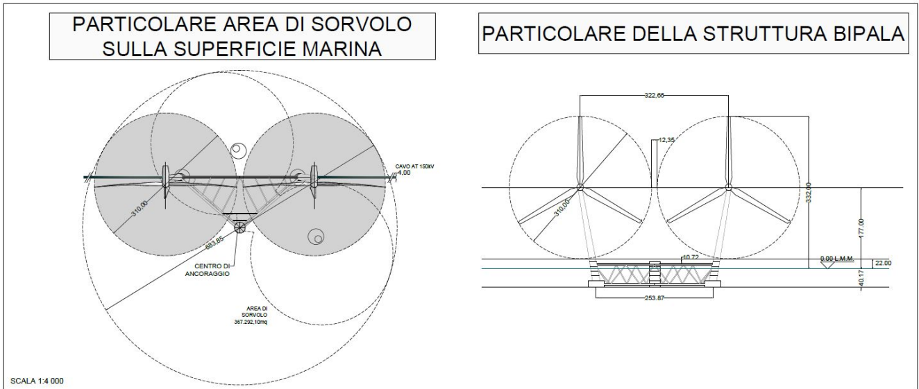
Figura 23 – Dimensionamento struttura "floating" tipo.
