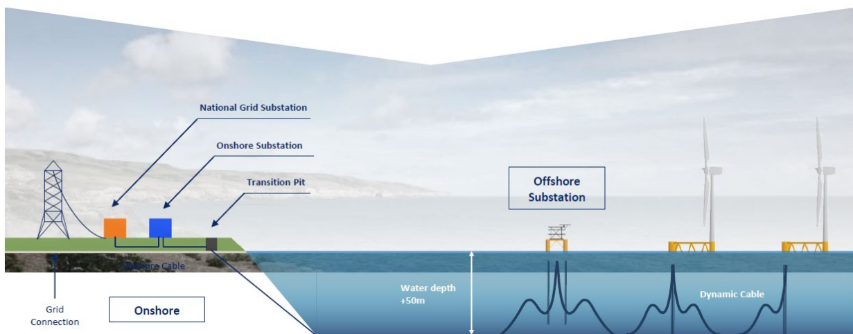
Figura 33 – Schema funzionale di collegamento elettrico.
