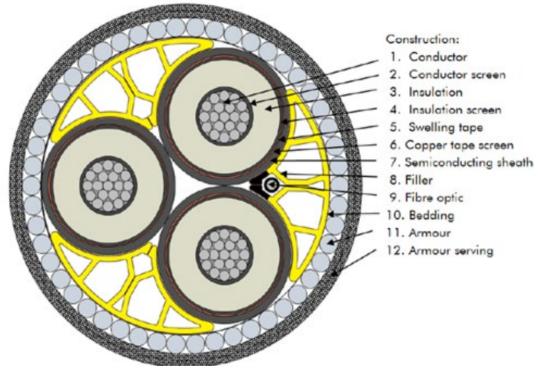
Figura 30 – Struttura cavo 150 kV.
