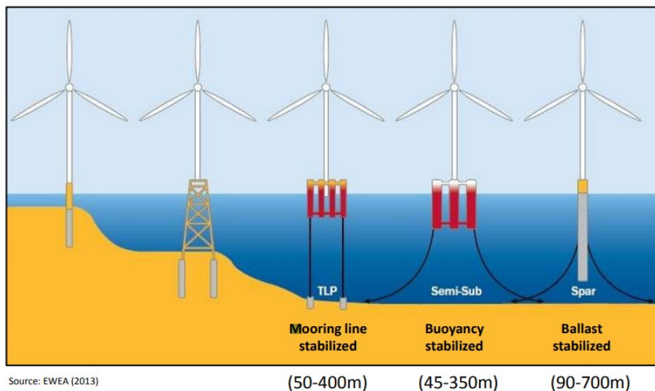
Figura 24 – Tipologie di fondazioni off-shore.
