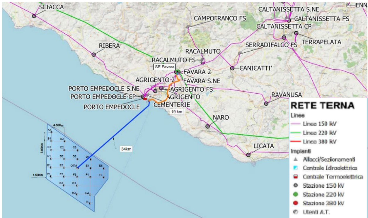
Figura 34 – Inquadramento SE Favara su Cartografia di Rete (Terna S.p.A.).
