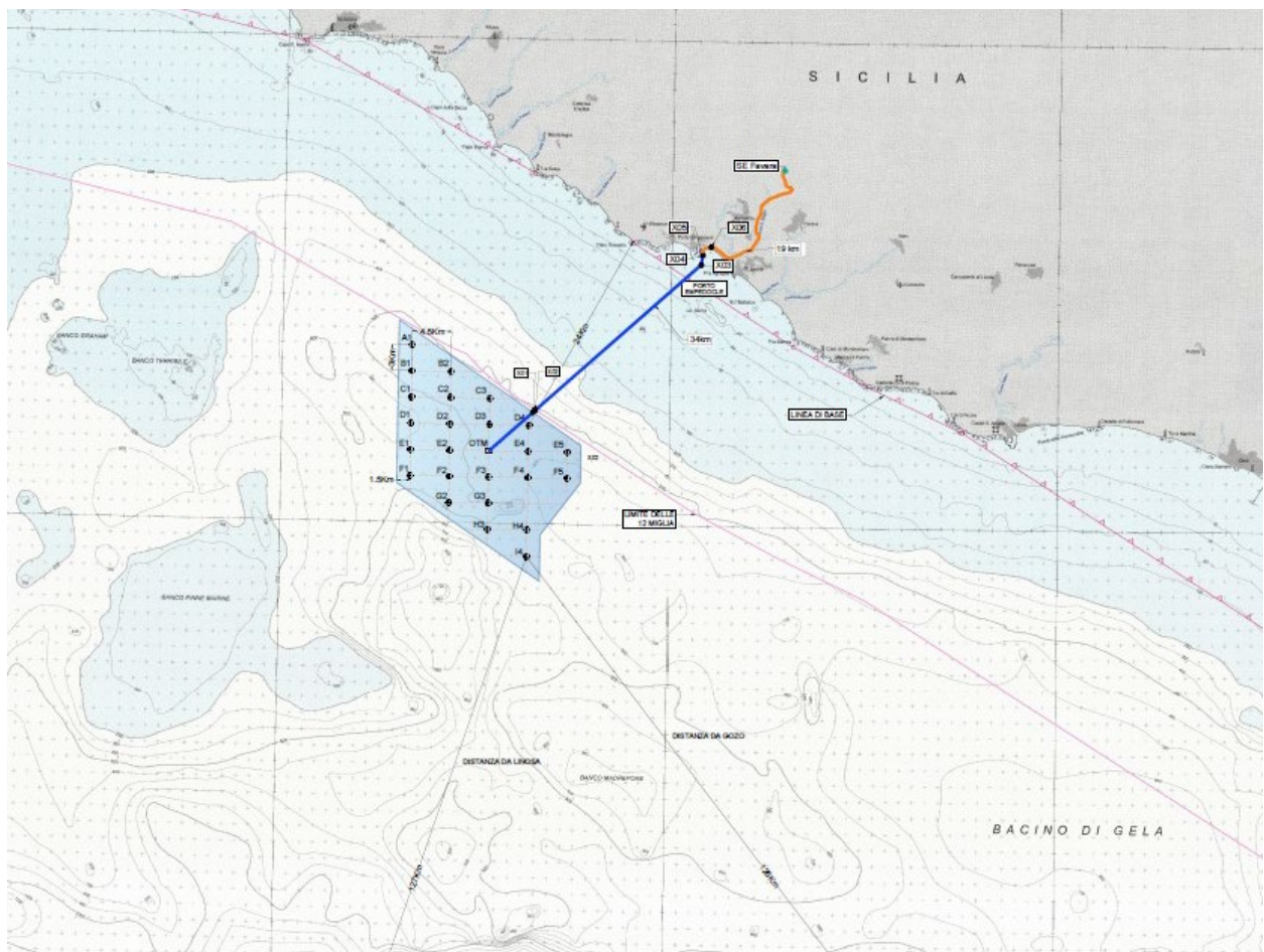
Figura 14 – Layout su carta batimetrica
