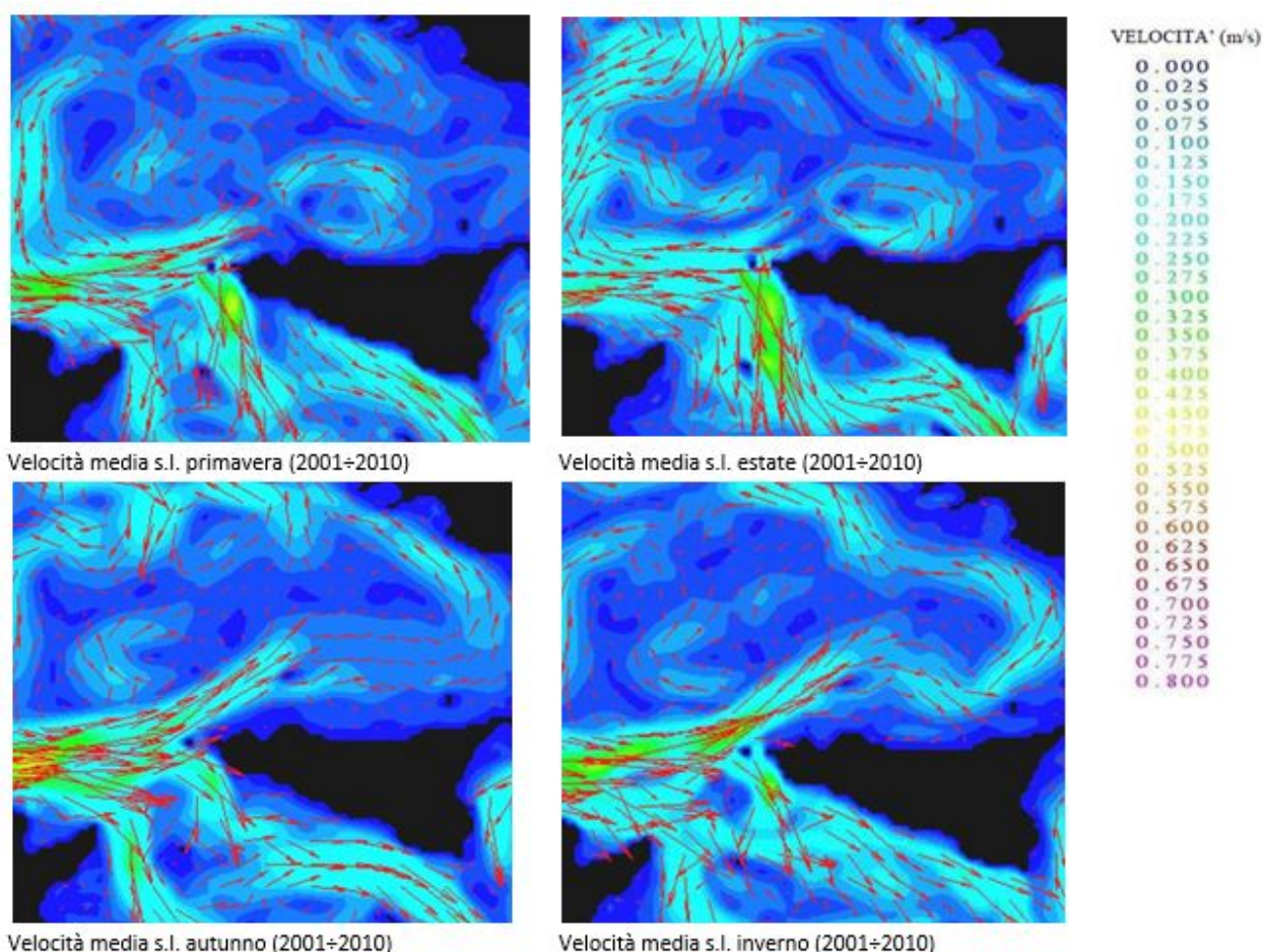
Figura 15 - Direzioni e velocità stagionali correnti marine
