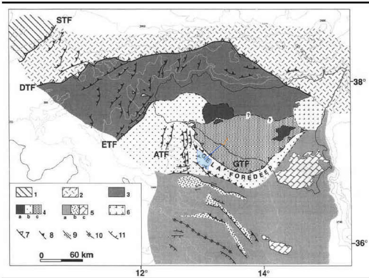
Figura 11 – Mappa geologica del Canale di Sicilia
