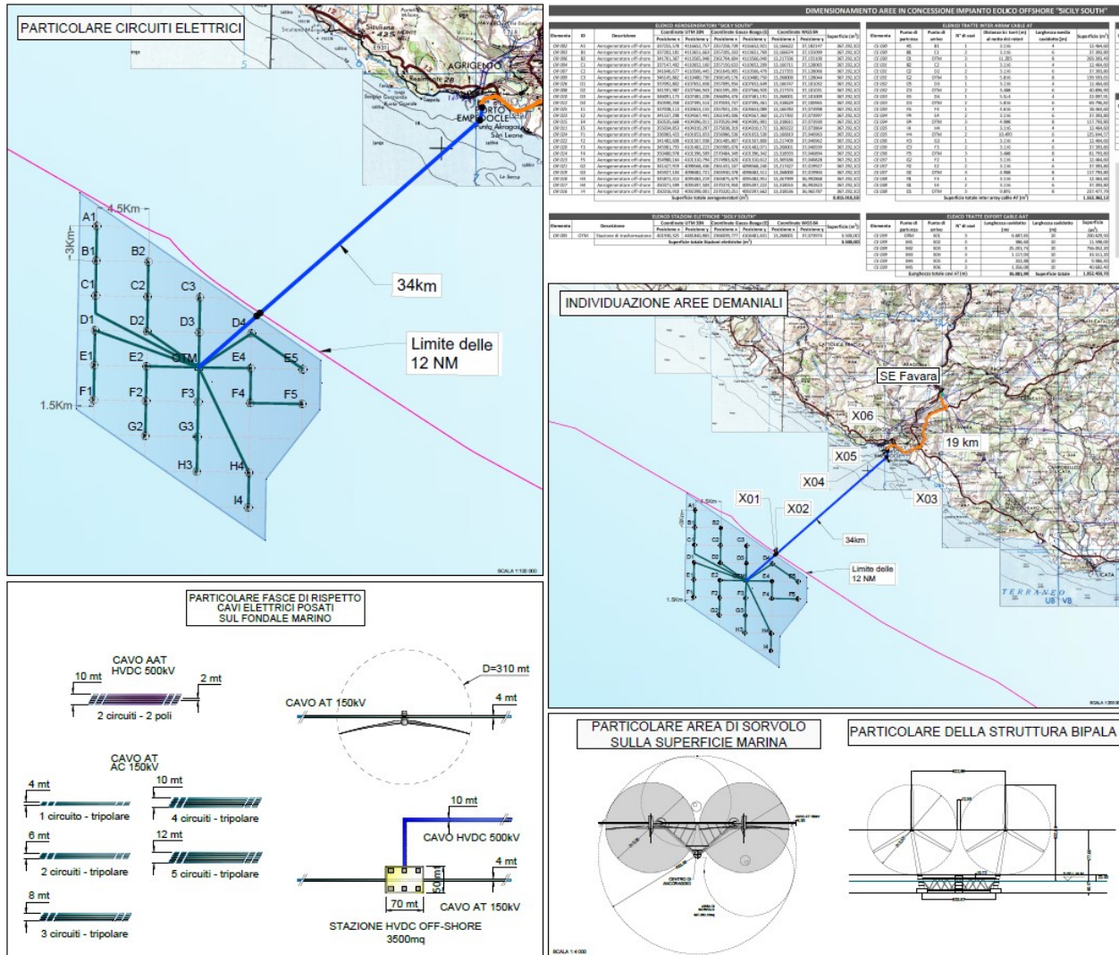
Figura 8 – Layout Parco eolico e particolare delle aree richieste in Concessione.
