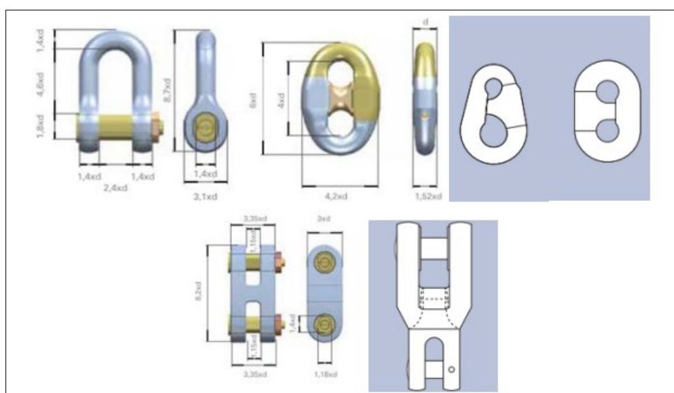
Figura 3.4: Giunti di connessione comunemente usati nell'industria offshore
