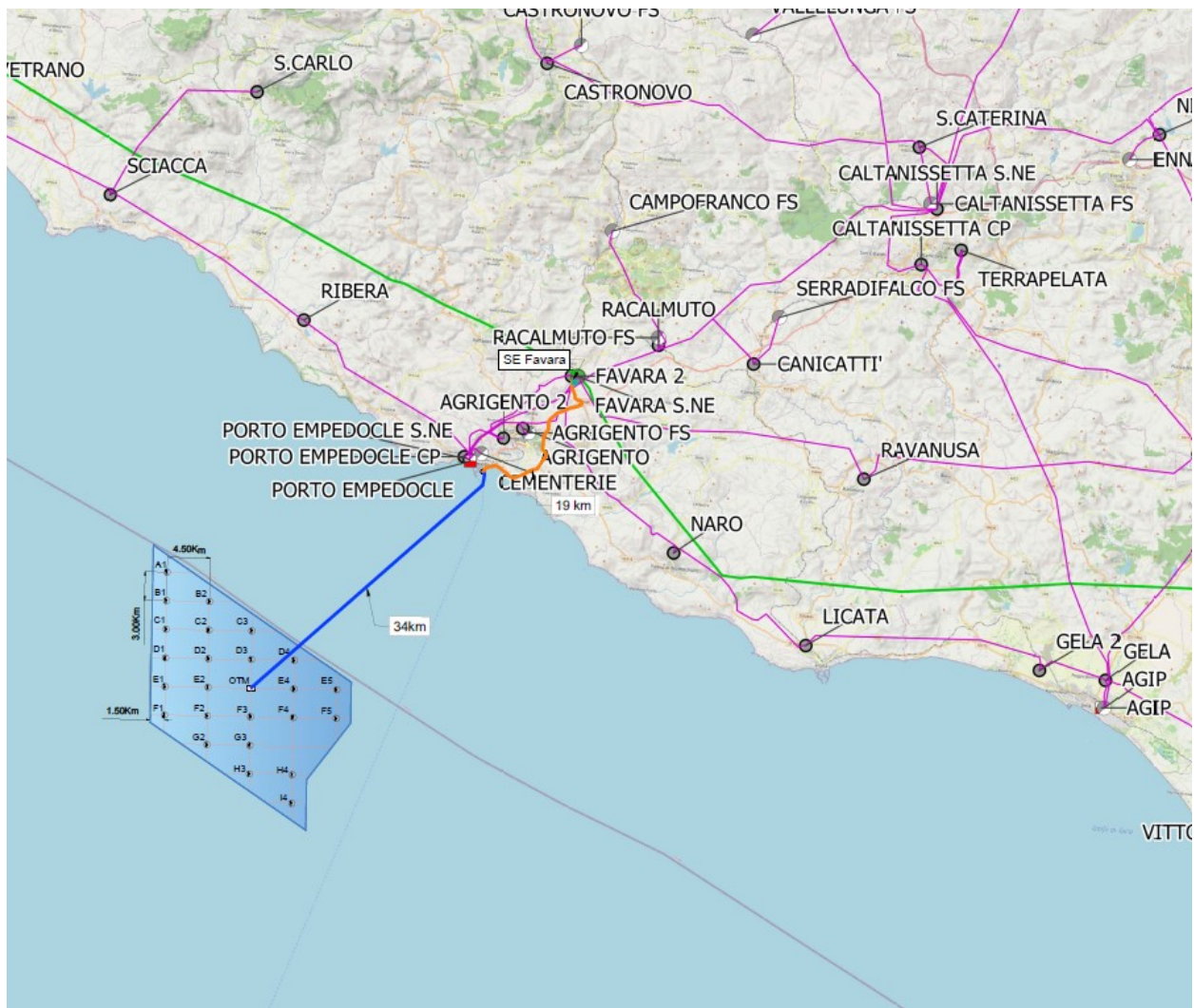
Figura 15 – Inquadramento su Atlante di Rete di Terna (Terna S.p.A.).
