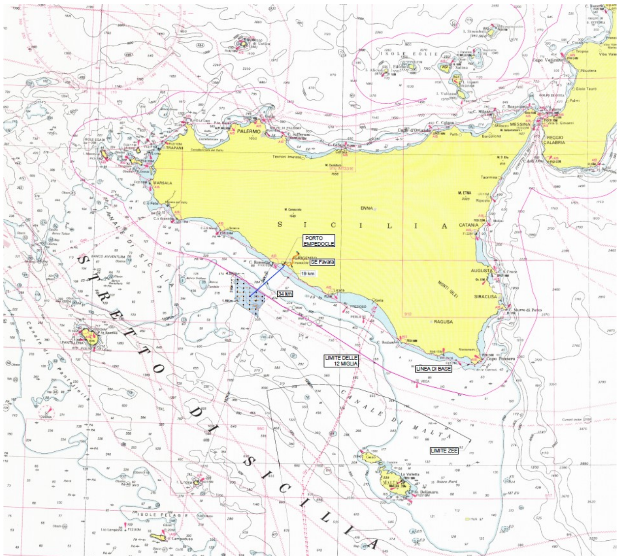
Figura 2 – Layout su carta nautica.
