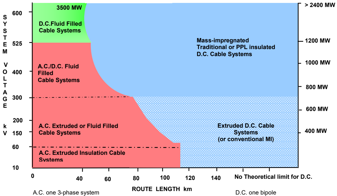
Figura 5 – Tecnologie dei cavi di trasmissione dell'energia.
