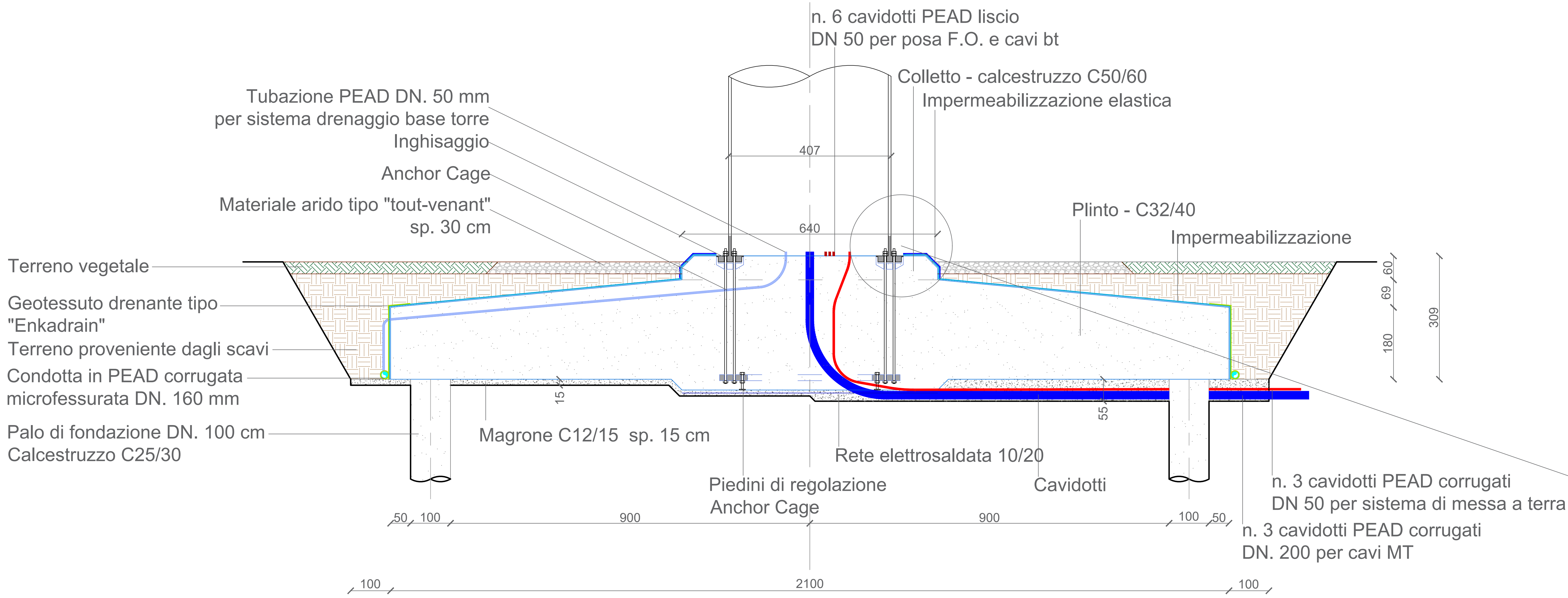
SEZIONE A-A'
