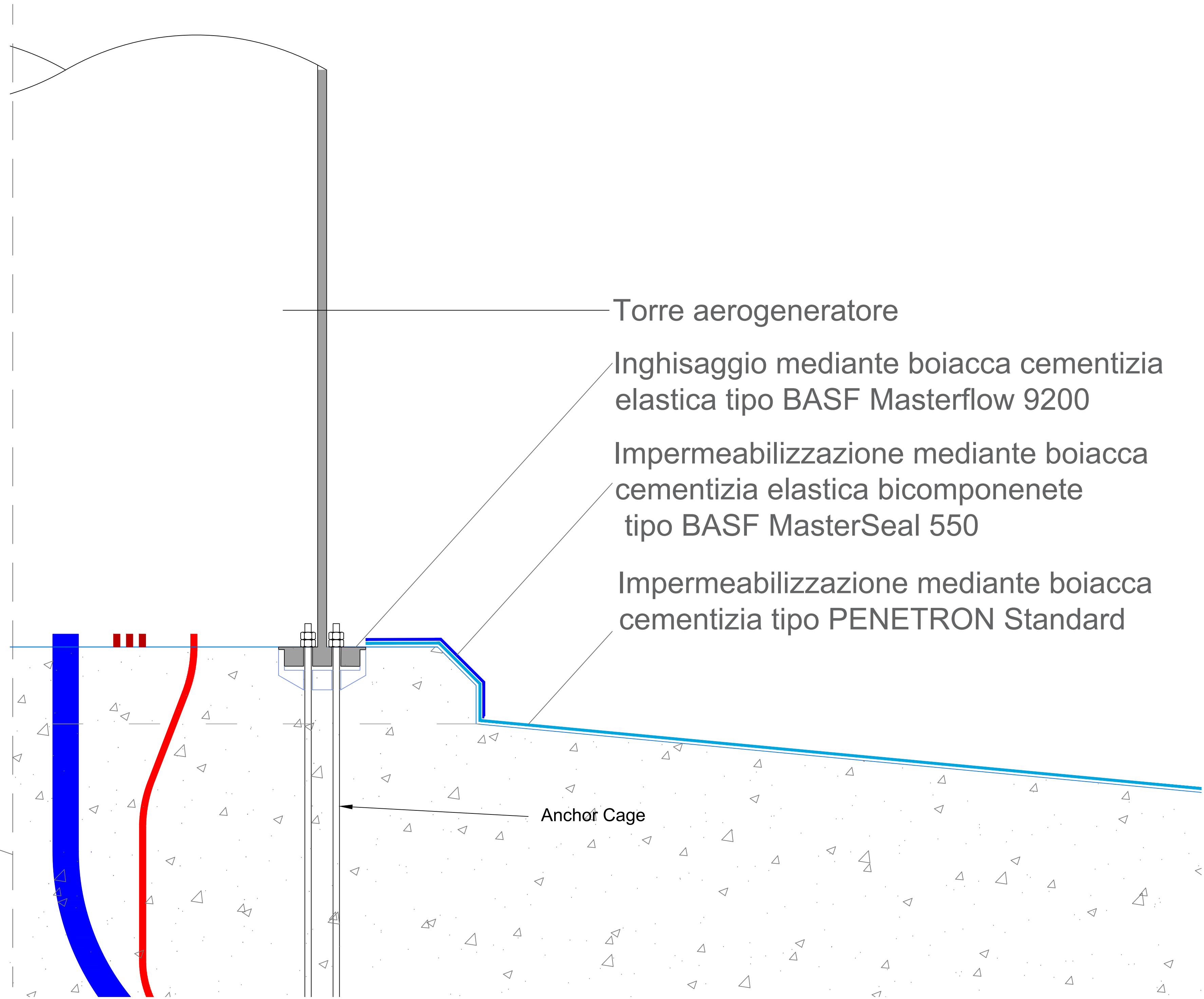
DETTAGLIO COLLETTO (scala 1:20)
