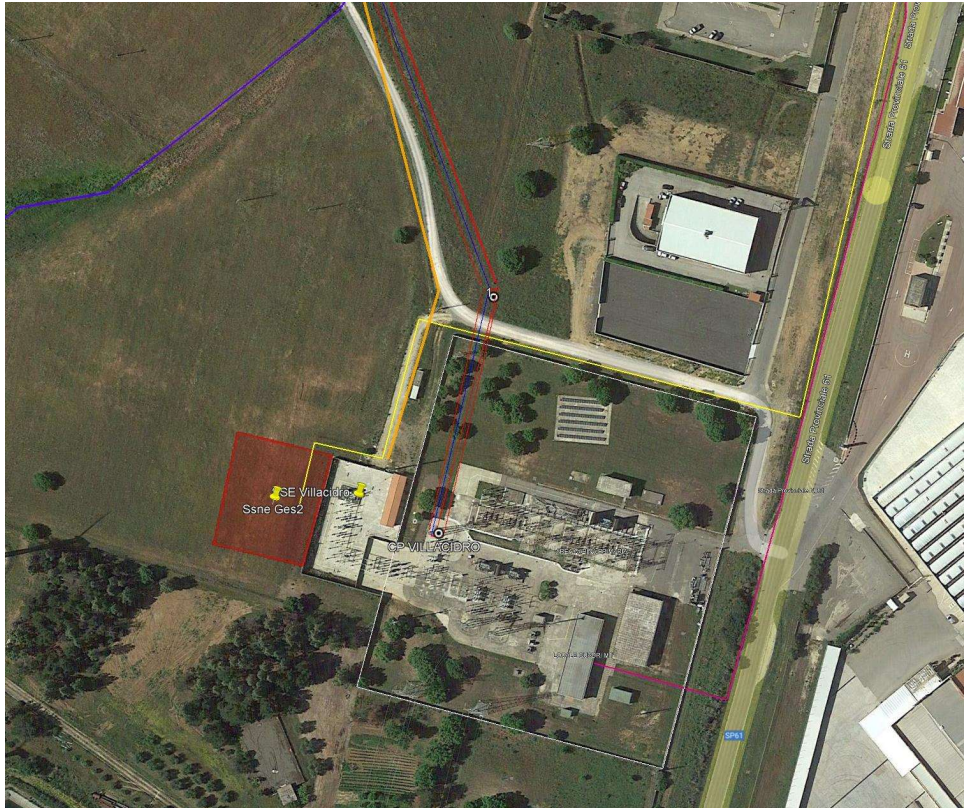
INQUADRAMENTO S.S. IMPIANTO "PV VILLACIDRO 2"
