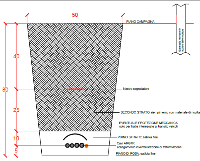
Figura 4-3: particolare dei cavi interni alle aree del parco fotovoltaico
