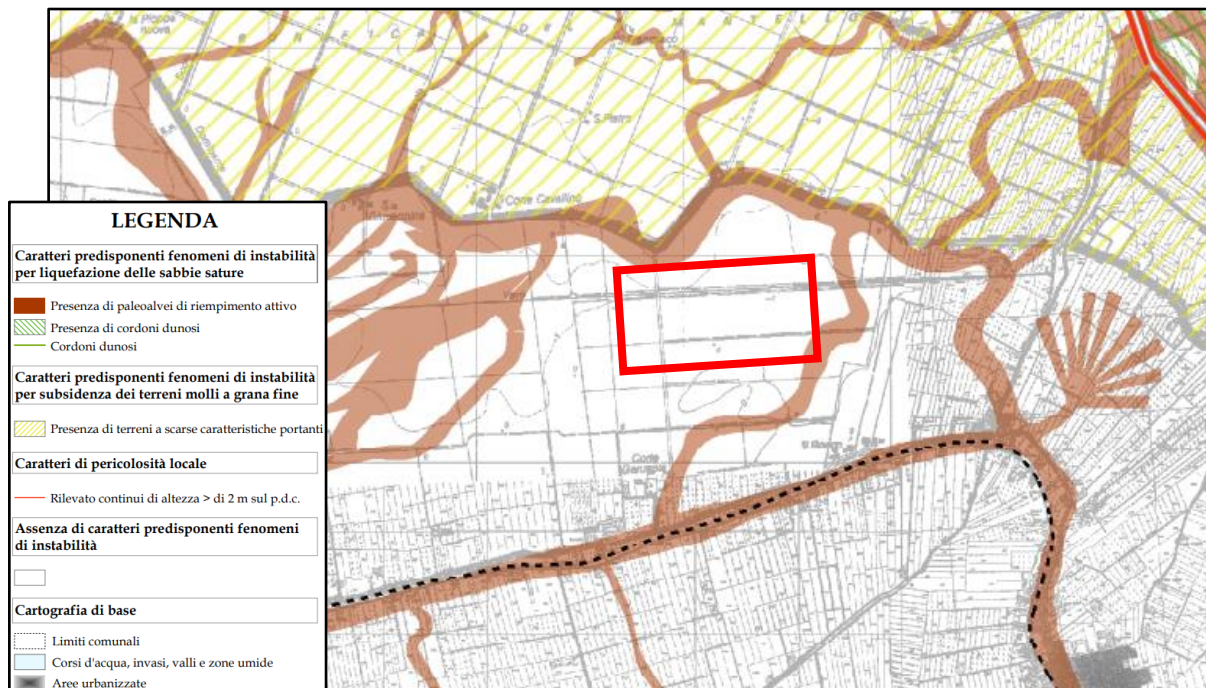
Figura 3-8: Inquadramento geomorfologico del territorio comunale di Argenta, con ubicazione dell'area in esame (rettangolo rosso), tratto dalla carta della potenziale presenza dei caratteri predisponenti agli effetti di sito a supporto del PSC.
