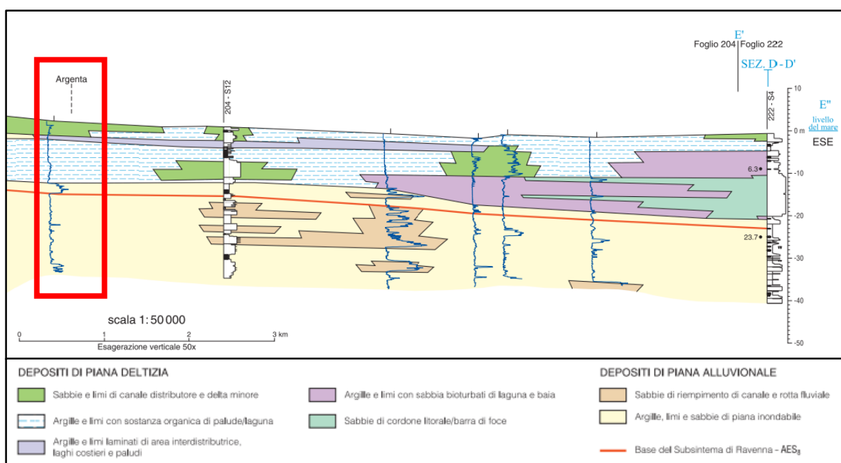
Figura 3-6: Sezione geologica di riferimento n.115 (geoportale dell'Emilia-Romagna) con ubicazione dell'area in esame (rettangolo rosso).
