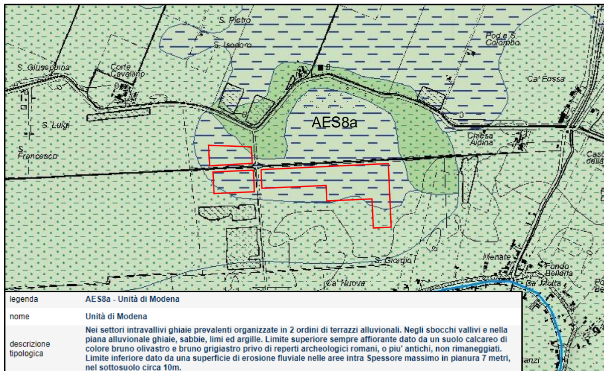
Figura 3-3: estratto della cartografia geologica della Regione Emilia-Romagna con ubicazione dell'area in esame (rettangolo rosso).
