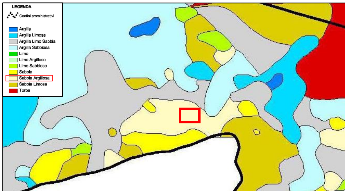
Figura 3-5: Inquadramento geologico del territorio comunale di Argenta, con ubicazione dell'area in esame (rettangolo rosso), tratto dalla carta delle litologie di superficie della Provincia di Ferrara.
