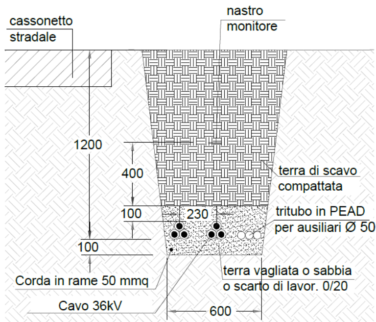
Figura 4-4: tipici di posa del cavidotto a 36 kV
