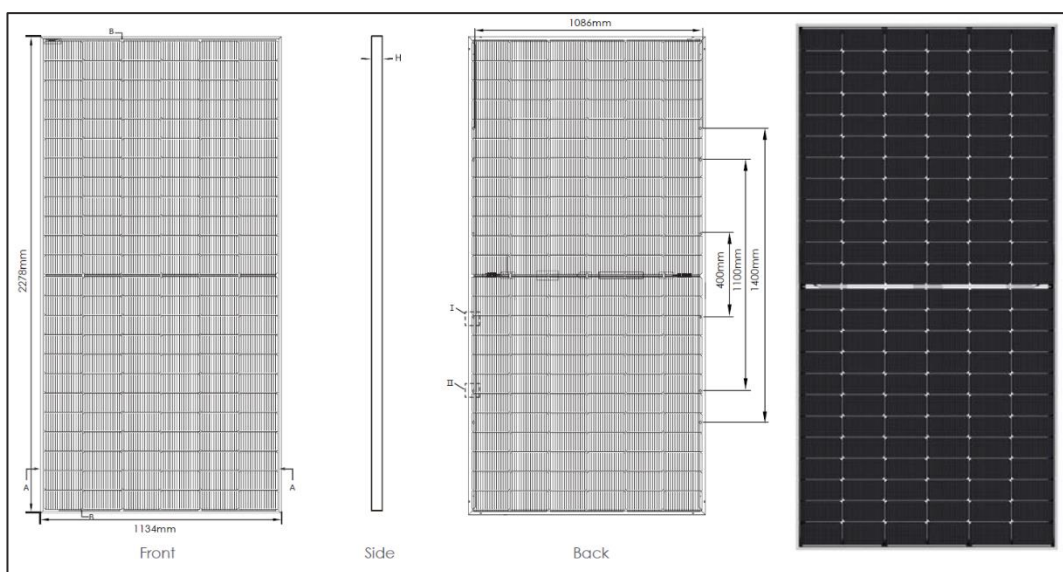
FIGURA 5: PANNELLO FV PARI A 570 Wp CON DIMENSIONI 2278 x 1134 x 30 MM
