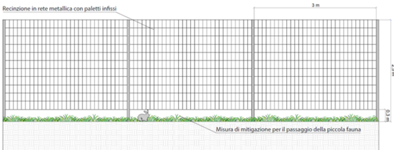
FIGURA 9: RECINZIONE TIPO
