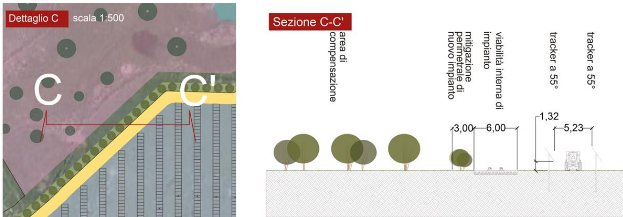
FIGURA 58 – PARTICOLARE FASCIA DI MITIGAZIONE E AREA DI COMPENSAZIONE – SEZIONE O-E DELL'IMPIANTO (ESTRATTO DALL'ELABORATO GRAFICO MAC2-PDT11)
