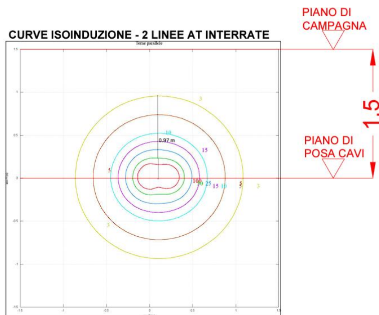
FIGURA 71 – CURVE ISOINDUZIONE – 2 LINEE AT INTERRATE (STRALCIO MAC2-PDT13)
