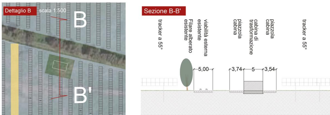
FIGURA 59 – PARTICOLARE FASCIA DI MITIGAZIONE E CABINA DI TRASFORMAZIONE – SEZIONE N-S DELL'IMPIANTO – ESTRATTO DALL'ELABORATO GRAFICO MAC2-PDT11)
