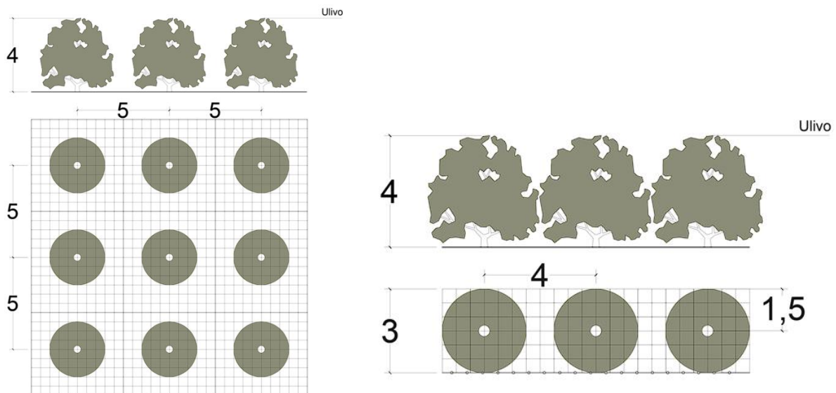
FIGURA 57 – SCHEMA D'IMPIANTO (ESTRATTO DALL'ELABORATO GRAFICO MAC2-PDT11)
