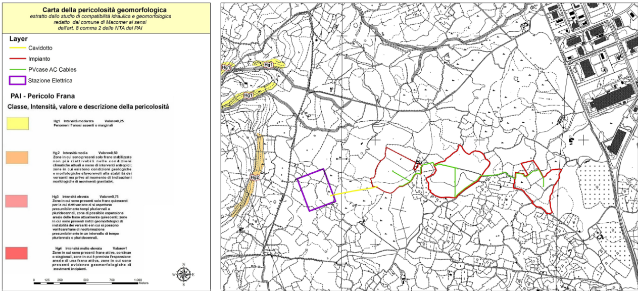
FIGURA 16 – INQUADRAMENTO AREA DI PROGETTO SU CARTA DELLA PERICOLOSITÀ DA FRANA – STRALCIO DELL’ELABORATO CARTOGRAFICO MAC2-IAT10
