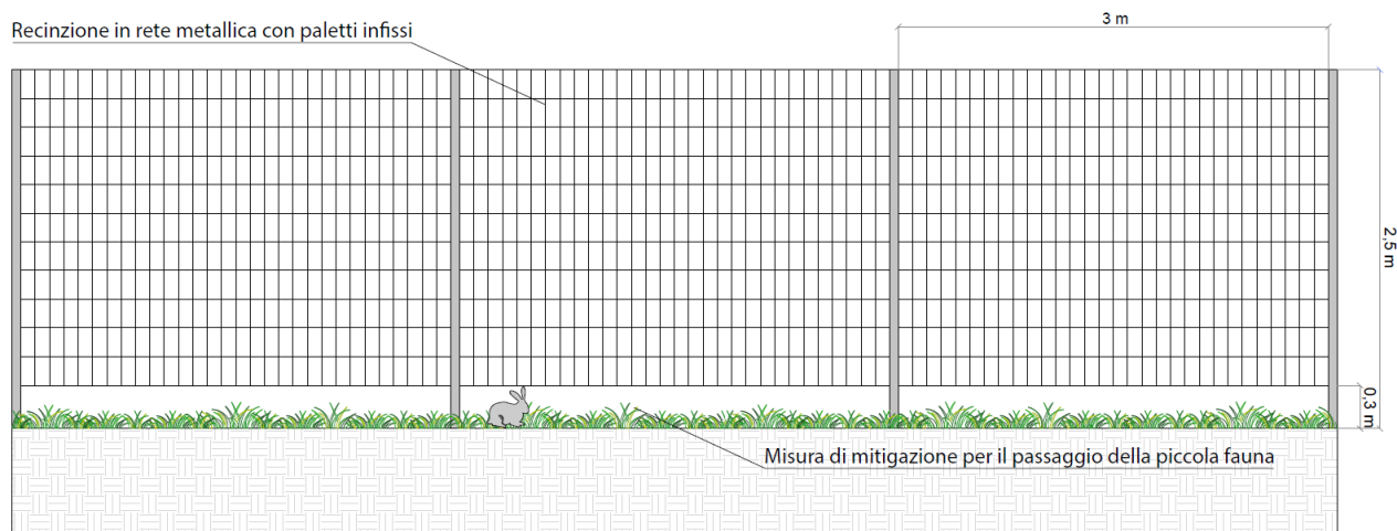
FIGURA 36 – ESEMPIO RECINZIONE METALLICA CHE DELIMITA L'AREA DI PERTINENZA DELL'IMPIANTO
