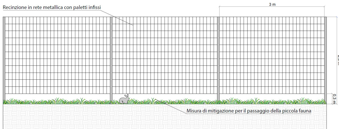
FIGURA 85 - RECINZIONE METALLICA A DELIMITAZIONE DELL'AREA DI IMPIANTO
