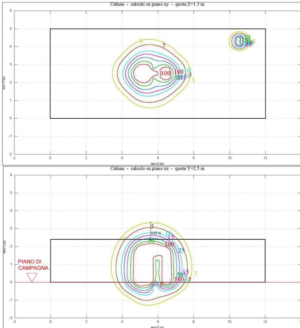
FIGURA 73 – CURVE ISOINDUZIONE CABINA AT CONSEGNA – PIANTA (IN ALTO) E PROSPETTO FRONTALE (IN BASSO). STRALCIO DELL'ELABORATO MAC2-PDT13.
