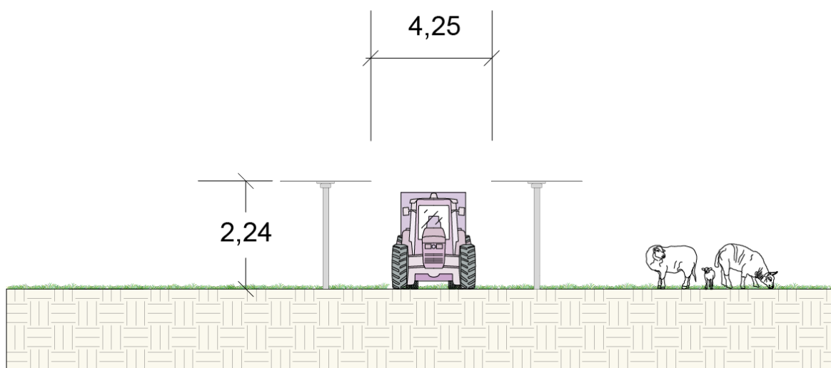
FIGURA 32 – SISTEMA AGRIVOLTAICO ELEVATO, SEZIONE TIPOLOGICA DELL'IMPIANTO
