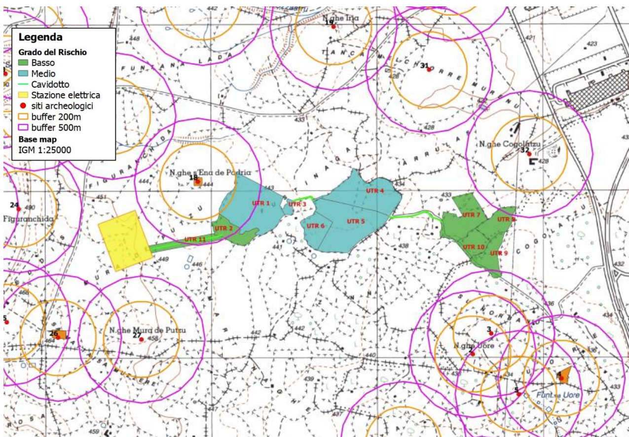
FIGURA 76 - CARTA DEL RISCHIO ARCHEOLOGICO - ESTRATTO ELABORATO MAC2-IAT14
