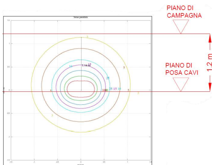
FIGURA 70 – CURVE ISOINDUZIONE – 3 LINEE BT INTERRATE (STRALCIO MAC2-PDT13)
