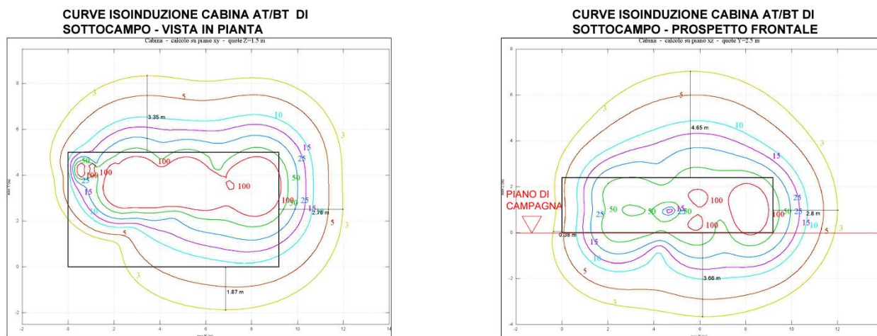
FIGURA 72 – CURVE ISOINDUZIONE AT/BT CABINA DI SOTTOCAMPO – VISTA IN PIANTA (A SX) E PROSPETTO (A DX). STRALCIO DELL'ELABORATO MAC2-PDT13
