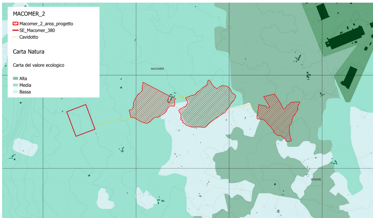
FIGURA 66 – INQUADRAMENTO AREA DI PROGETTO SU CARTA DEL VALORE ECOLOGICO – STRALCIO ELABORATO CARTOGRAFICO MAC2-IAT24
