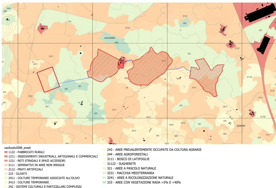
FIGURA 44 – INQUADRAMENTO DELL'AREA DI PROGETTO SU CARTA USO DEL SUOLO CLC2008 (STRALCIO DELL'ELABORATO CARTOGRAFICO MAC2-IAT04)
