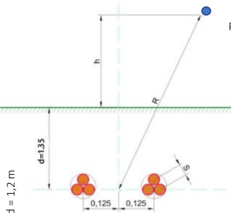
Figura 4: Modello fisico calcolo campo elettromagnetico – 2 terne
