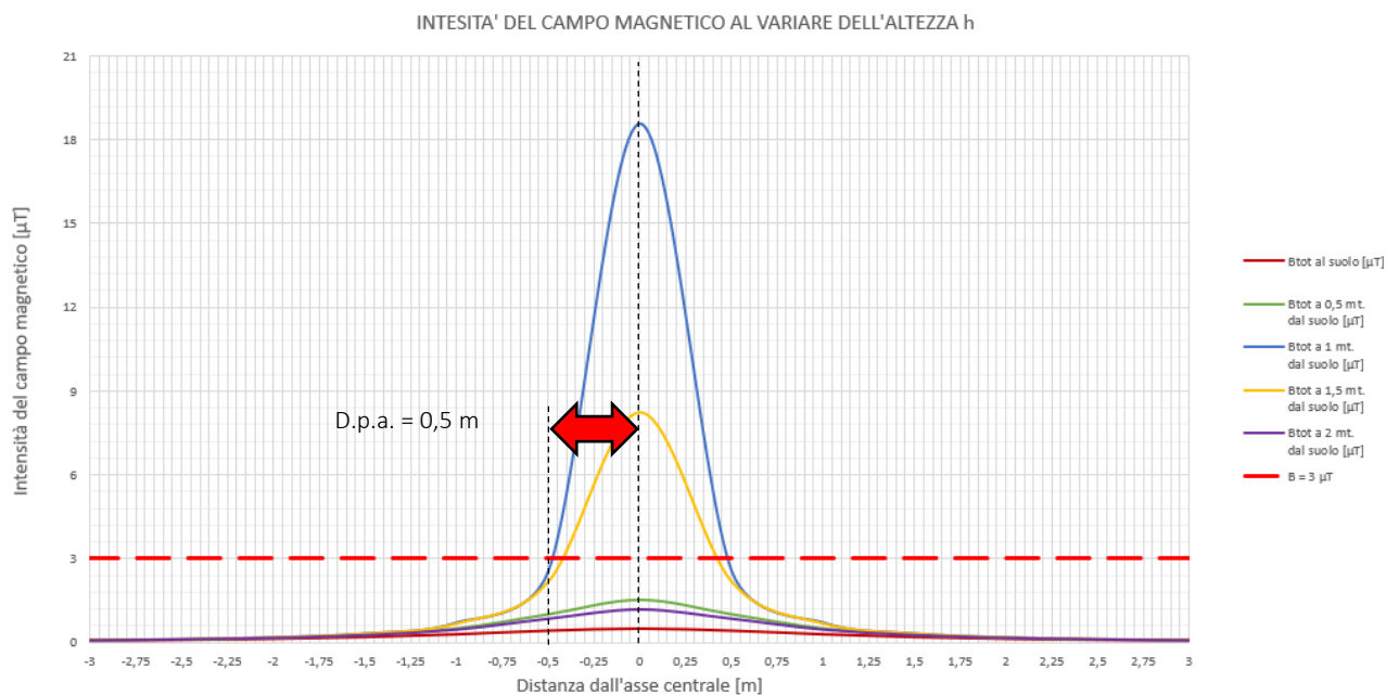
Figura 11: Diagramma dell'intensità dei campi elettromagnetici per la valutazione della D.P.A. – tratto S6
