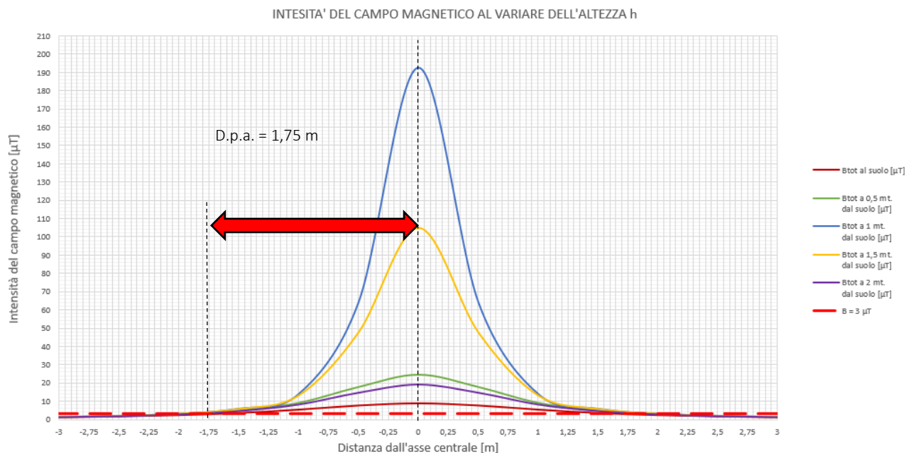
Figura 17: Diagramma dell'intensità dei campi elettromagnetici per la valutazione della D.P.A. – tratto S12
