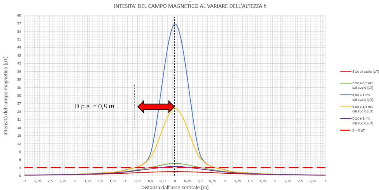
Figura 14: Diagramma dell'intensità dei campi elettromagnetici per la valutazione della D.P.A. – tratto S9
