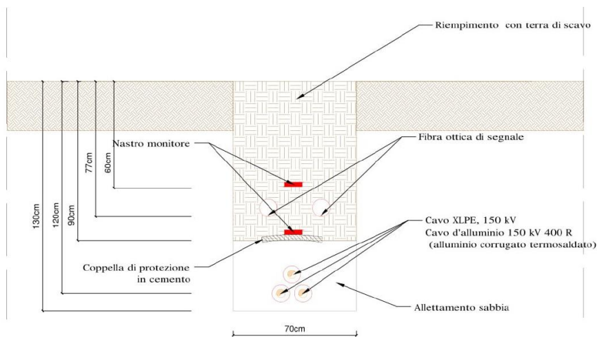
Figura 18: Particolari posa cavo interrato AT
