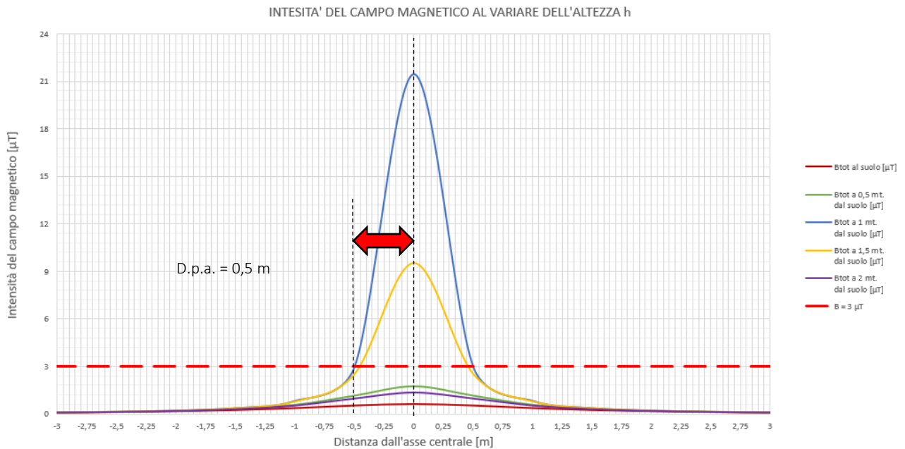
Figura 15: Diagramma dell'intensità dei campi elettromagnetici per la valutazione della D.P.A. – tratto S10
