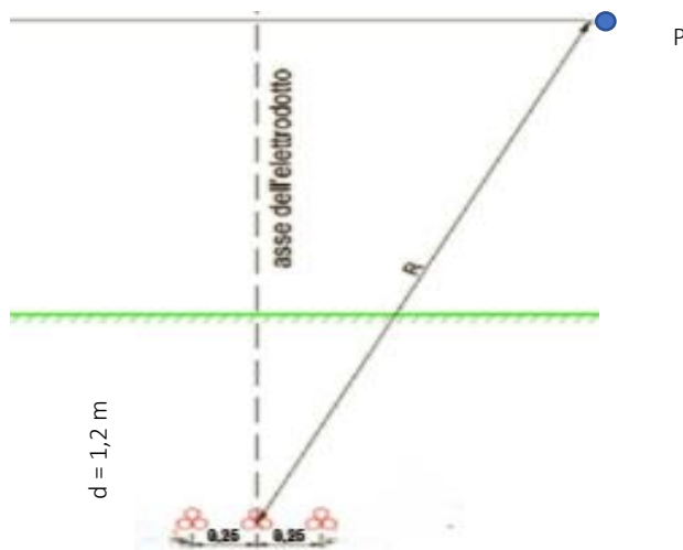
Figura 5: Modello fisico calcolo campo elettromagnetico – 3 terne
