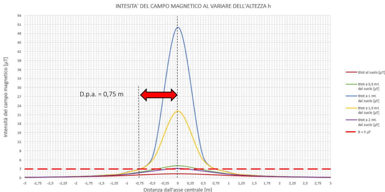
Figura 16: Diagramma dell'intensità dei campi elettromagnetici per la valutazione della D.P.A. – tratto S11
