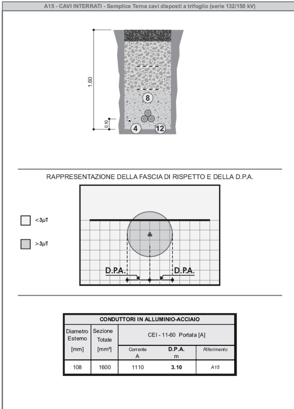
Figura 21: D.P.A. cavi interrati AT in semplice terna disposta a trifoglio - "Linea guida ENEL per l'applicazione del § 5.1.3 dell'allegato al D.M. 29.05.08"
