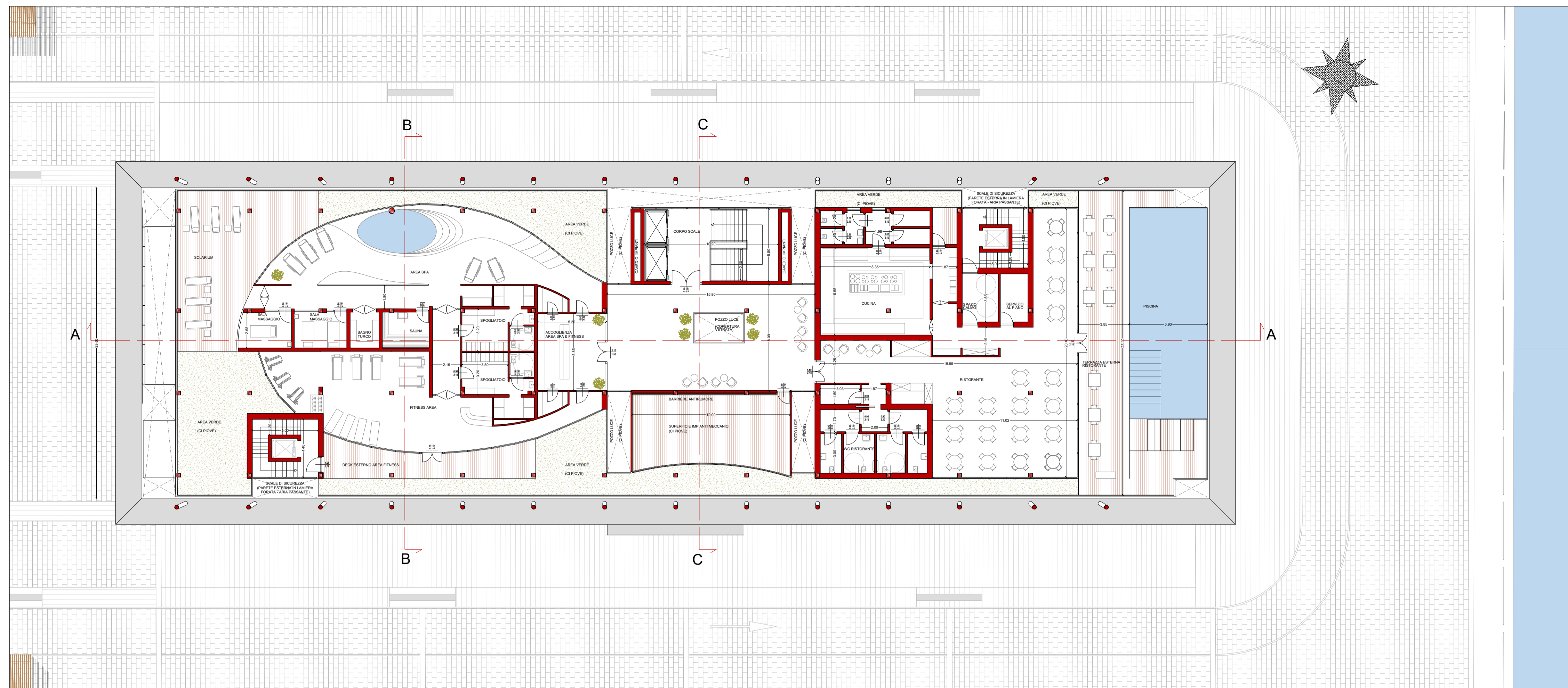
Centro servizi - Pianta quota +10.20 m_Piano terrazza: servizi per la nautica da diporto, area spa, area fitness e ristorante_ scala 1:200
