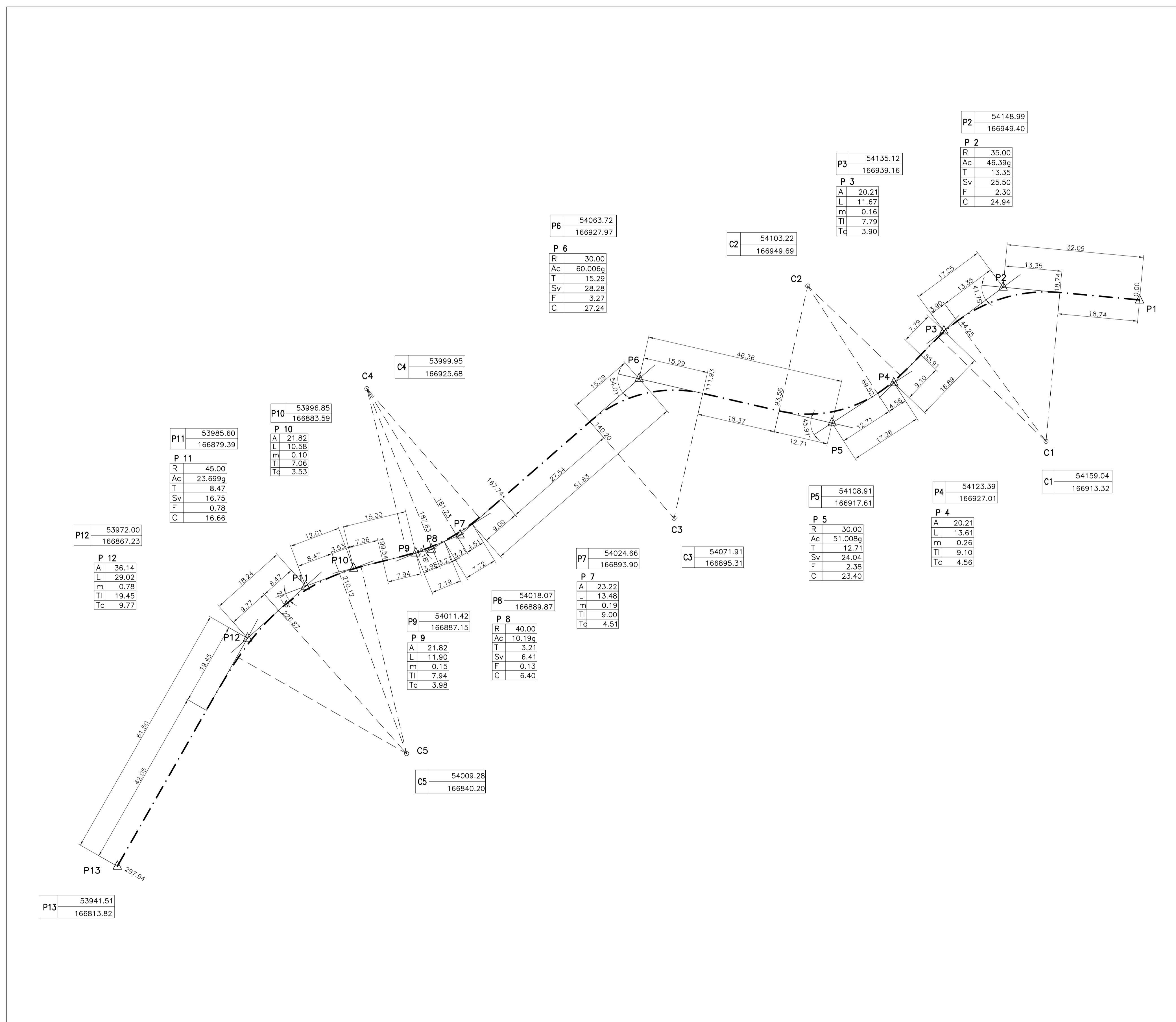
PLANIMETRIA DI TRACCIAMENTO Scala 1:500
