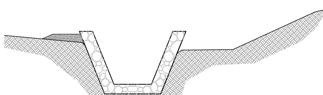
FASE 2: Rintiro laterale per strati; realizzazione rivestimento in massi cementati
