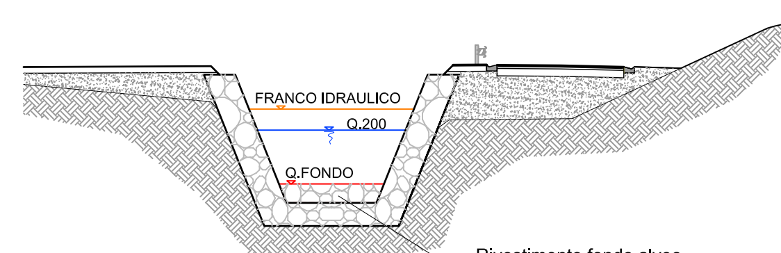
FASE 7: Fase finale, rivestimento fondo alveo in massi cementati fino alla quota di progetto
