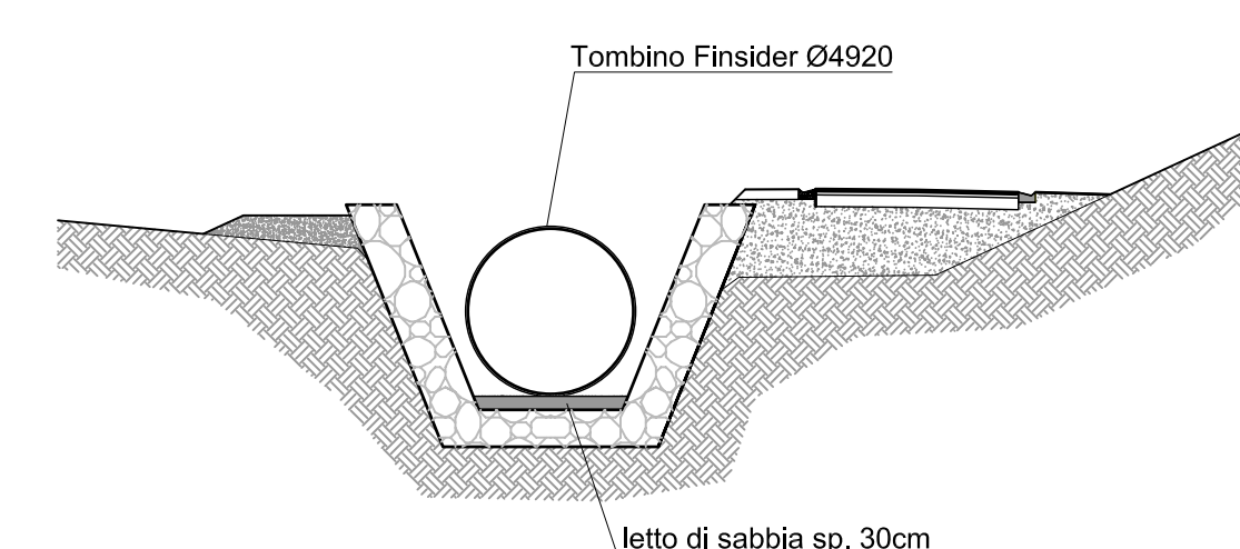
FASE 3: Realizzazione di letto in sabbia; Posa tombino Finsider; realizzazione strada
