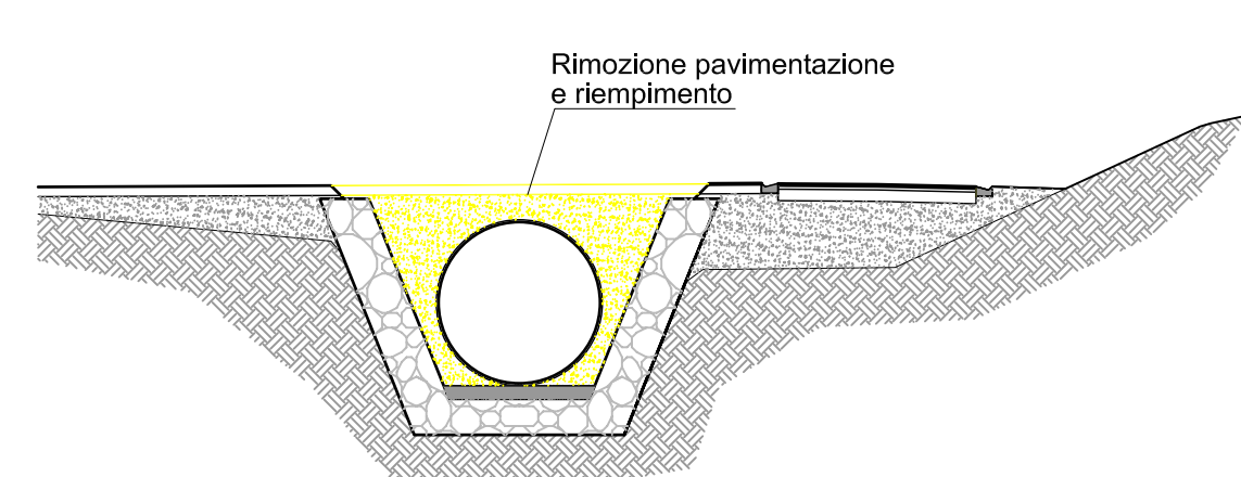
FASE 5: Scavo della parte del piazzale sovrastante il tombino
