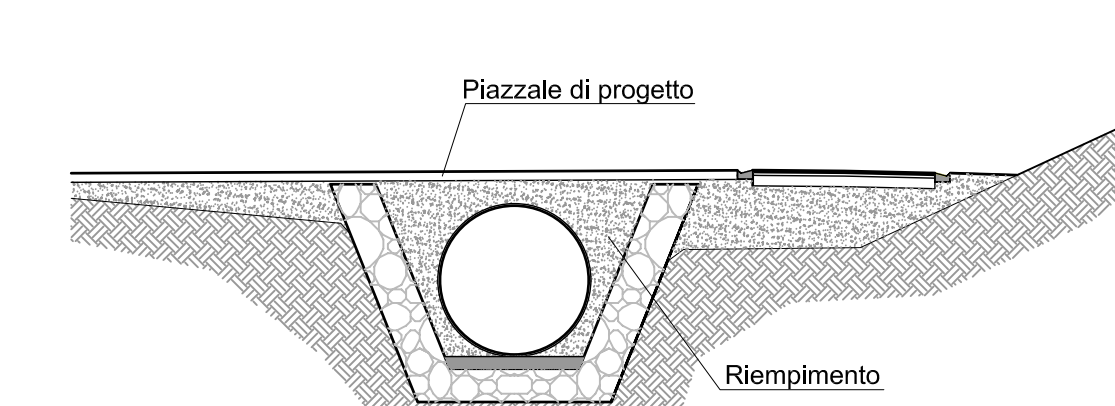
FASE 4: riempimento alveo e realizzazione piazzale
