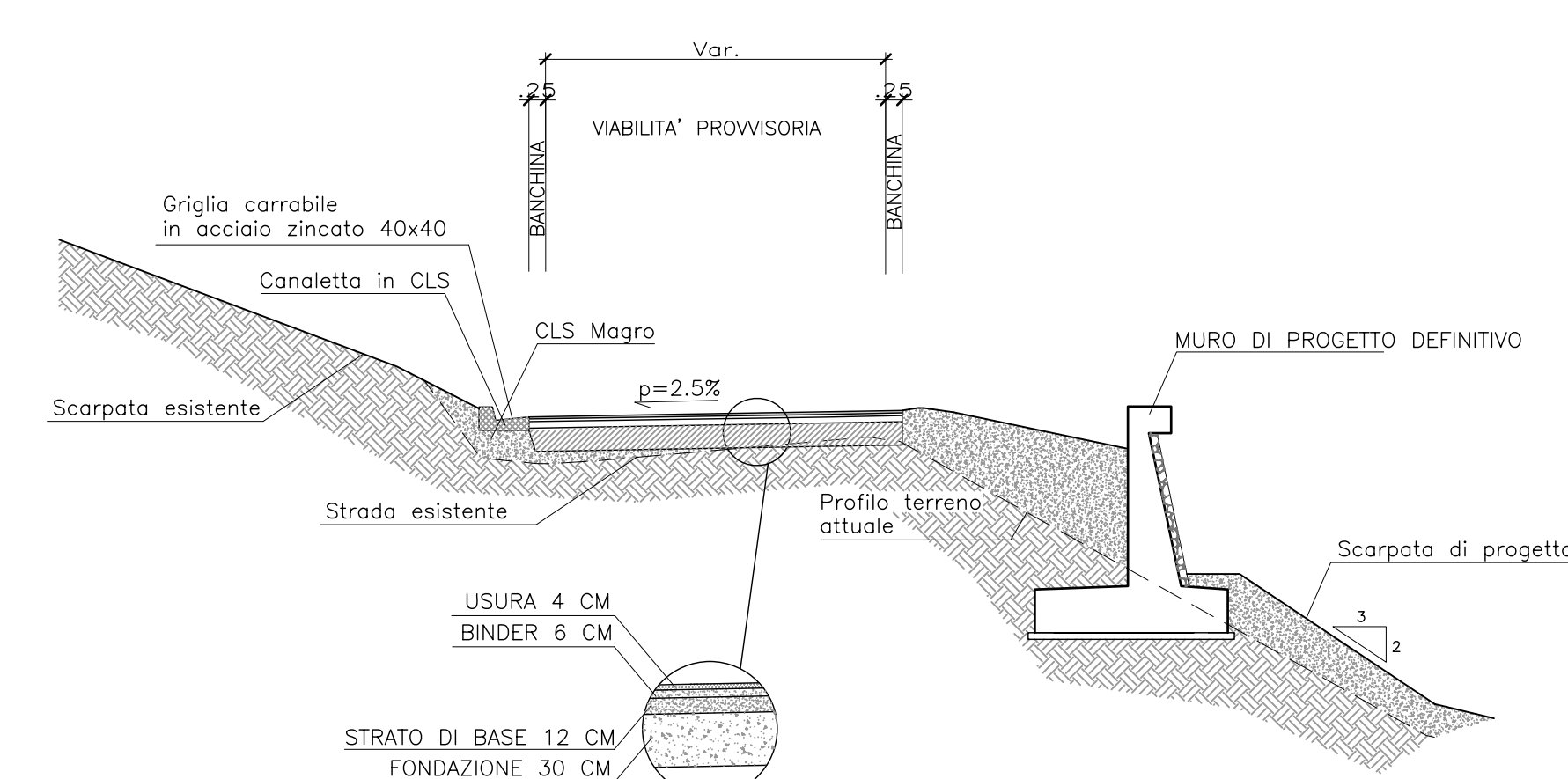
SEZIONE TIPO SITEMAZIONE PROVVISORIA SCALA 1:100
