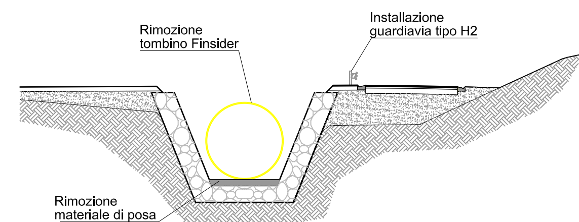
FASE 6: Rimozione del Finsider e del letto di sabbia; montaggio di guardiavia definitivi
