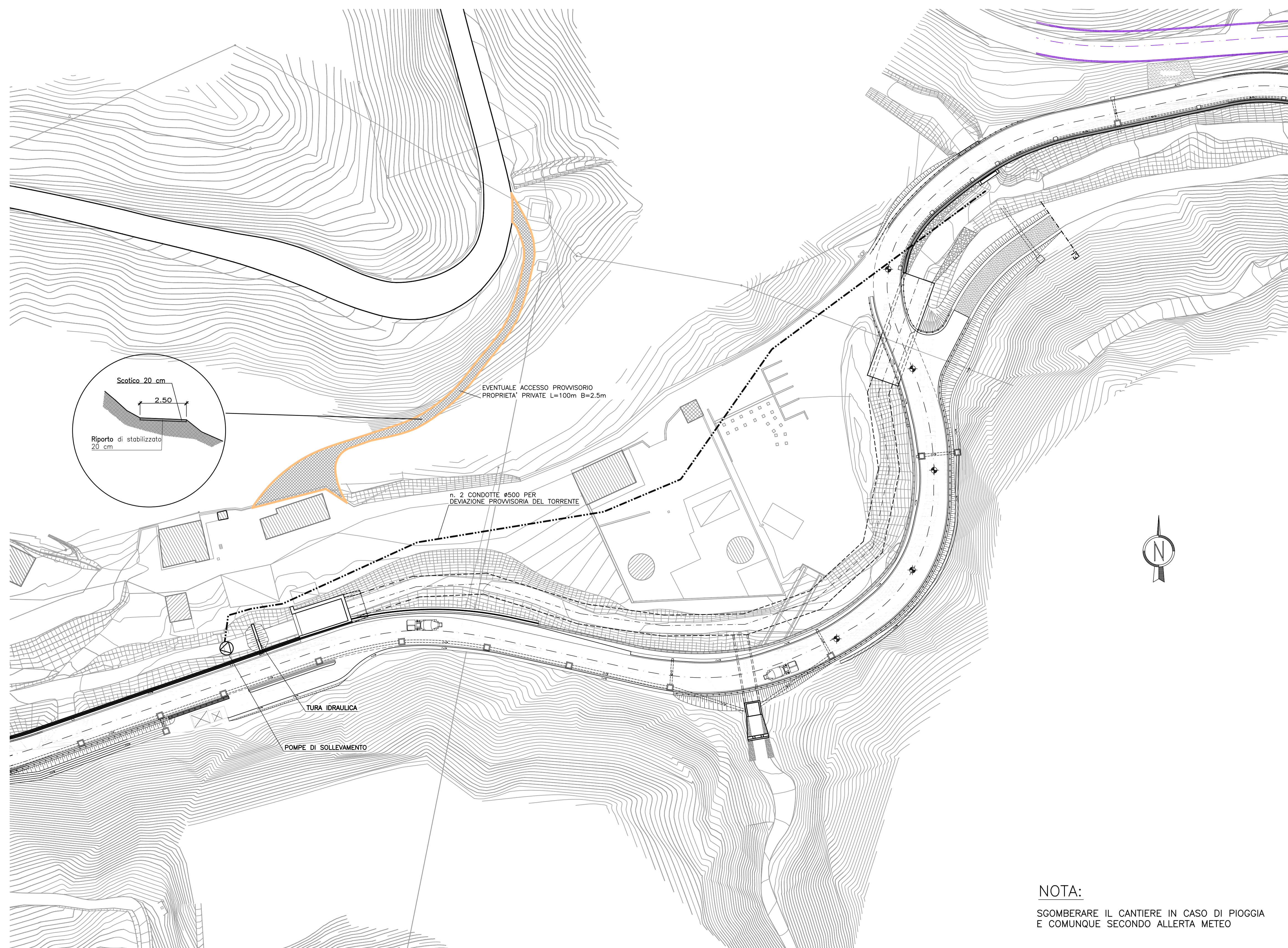
PLANIMETRIA SCALA 1:500
