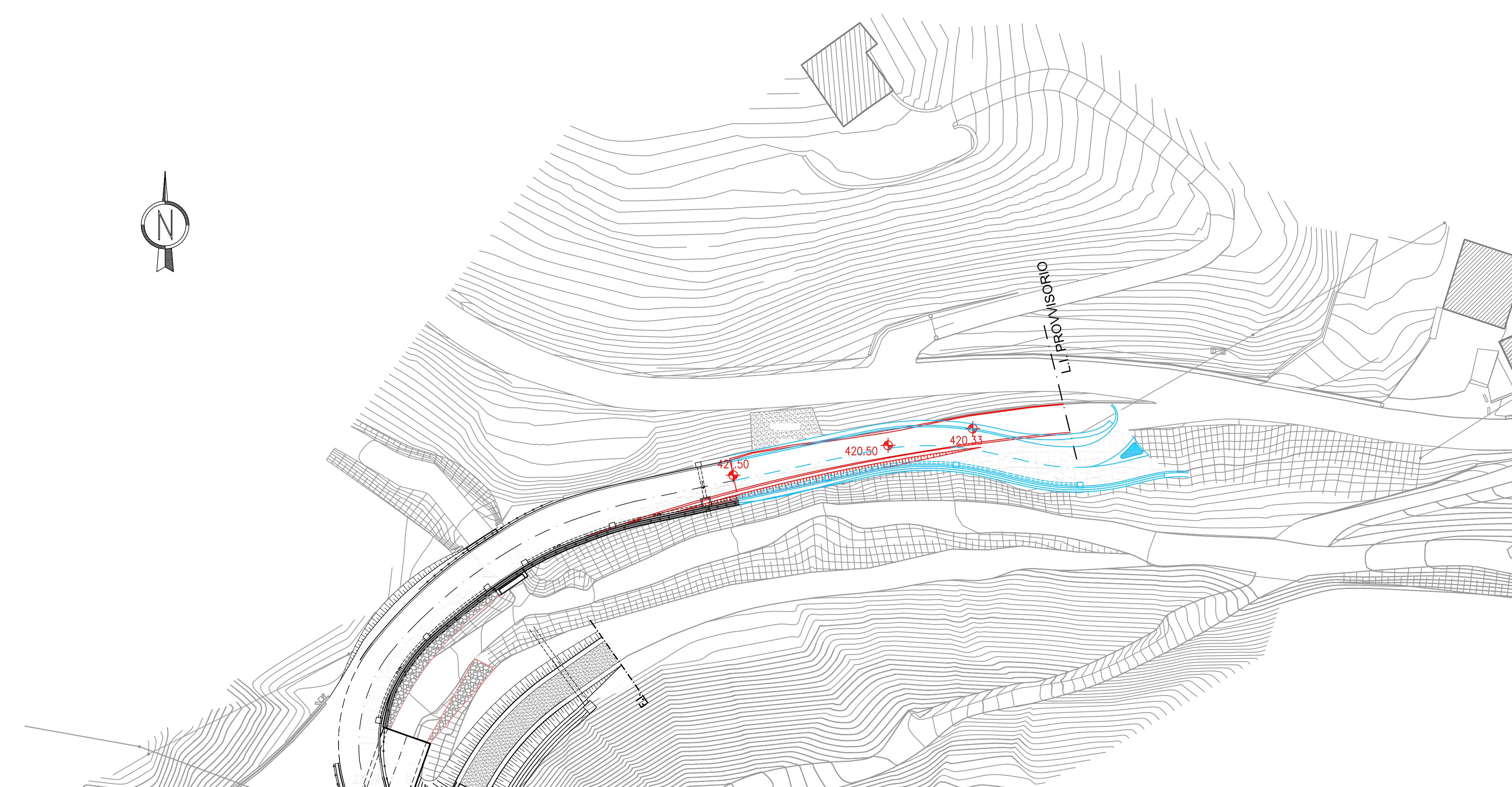
PLANIMETRIA SISTEMAZIONE PROVVISORIA Scala 1:500
