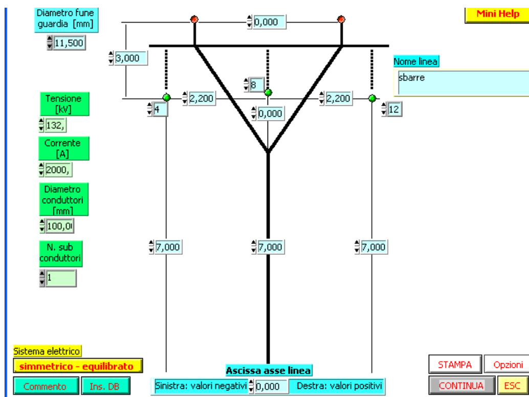
Figura 7: Linea AT con disposizione conduttori in piano assimilabile ad un sistema a sbarre a 220 kV
