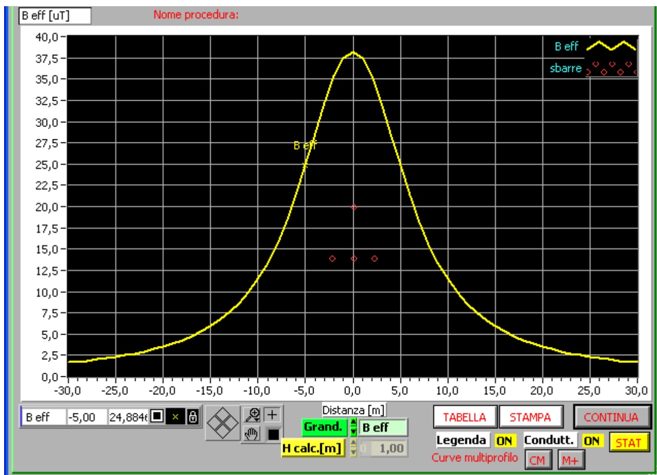
Figura 8: Andamento del campo di induzione magnetica per I = 2000\text{ A}
