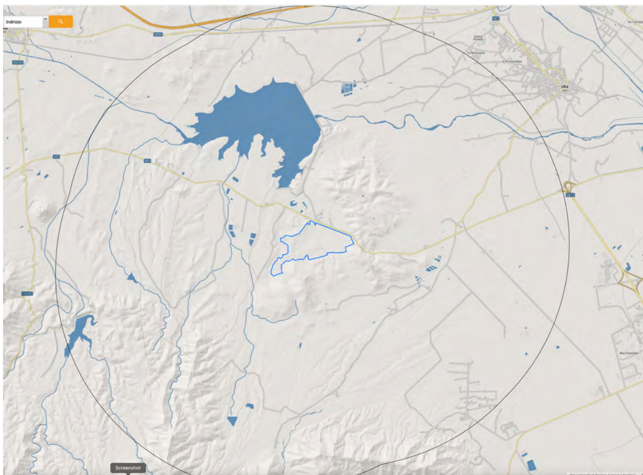
Figura 36 – elementi geomorfologici e territoriale (GDBT)
