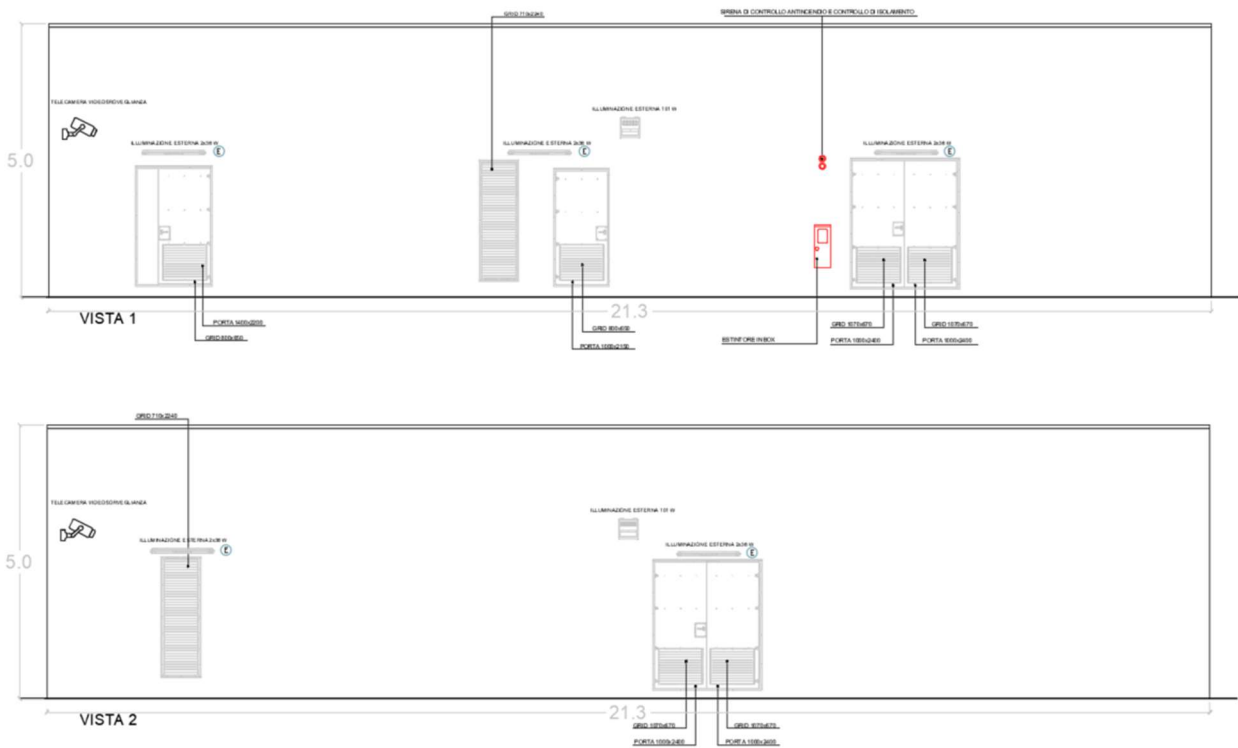
Figura 4.7 - Posizionamento sistema video sorveglianza e illuminazione esterna Gabina Generale AT
